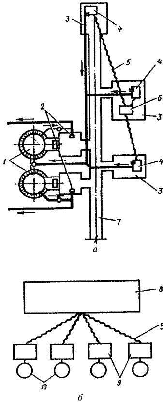
Рис. 4. Схема устройства резервного электроснабжения артезианских скважин a — план; б — электрическая схема; 1 — резервуар питьевой воды с фильтрами-поглопителями; 2 — колодец для отбора воды в передвижную тару; 3 — площадка для обслуживания артезианских скважин; 4 — водозаборная скважина, намеченная к работе в чрезвычайных ситуациях от временного источника электроснабжения; 5 — кабель; 6 — передвижная электростанция; 7 — подземная автодорога; 8 — панель выводов передвижной электростанции; 9 — станции управления погружными насосами; 10 — погружные насосы
