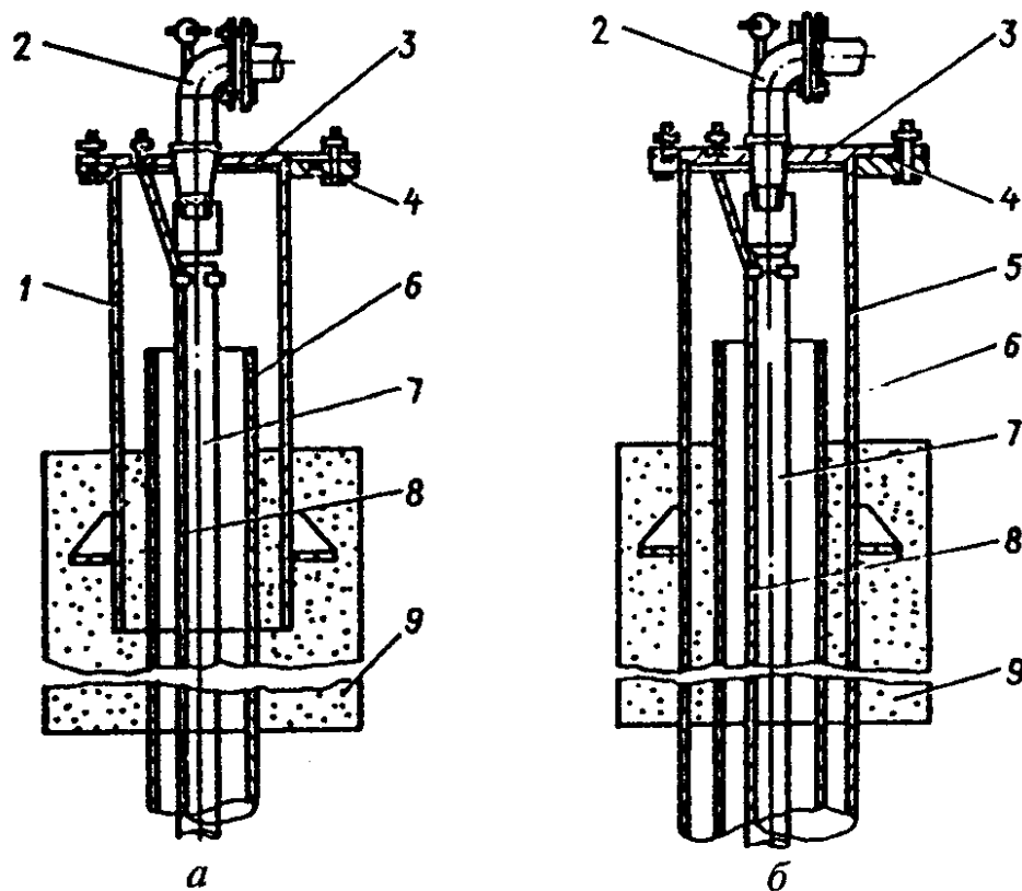
Рис. 3. Устройство герметизированных оголовков артскважин
