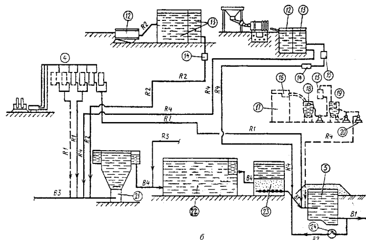
"Рисунок 7. Схема устройств для приготовления и дозирования реагентов на водоочистных станциях при двухступенной схеме очистки"
