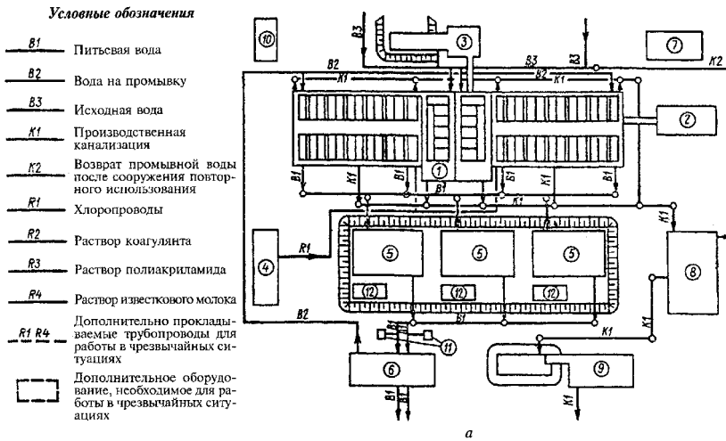
Рис. 6. Схема устройств для приготовления и дозирования реагентов на водоочистных станциях при одноступенной схеме очистки
