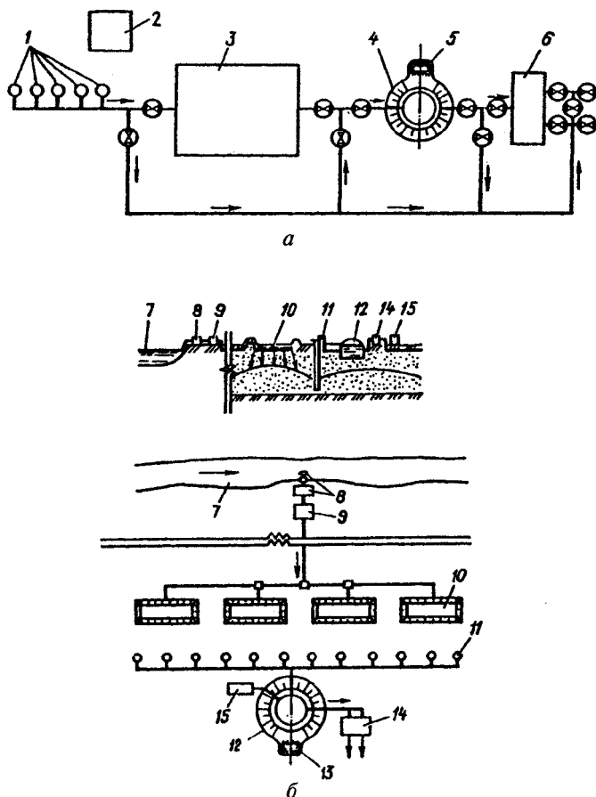
Рис. 2. Принципиальные технологические схемы сооружений
