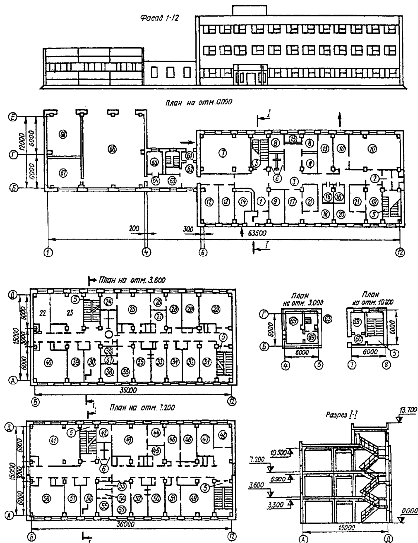
Рис. 10. Базовая лаборатория для проведения анализов питьевых и сточных вод
