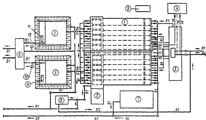
Рис. 7. Схема устройств для приготовления и дозирования реагентов на водоочистных станциях при двухступенной схеме очистки
