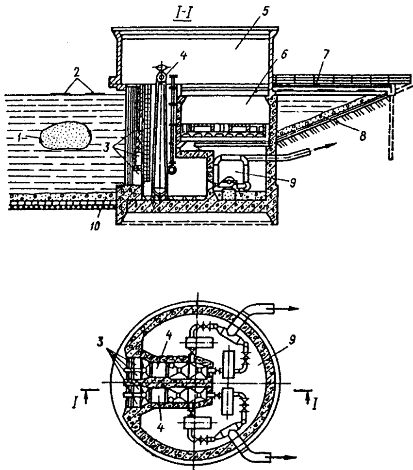
Рис. 5. Водозаборы из поверхностных водоисточников
