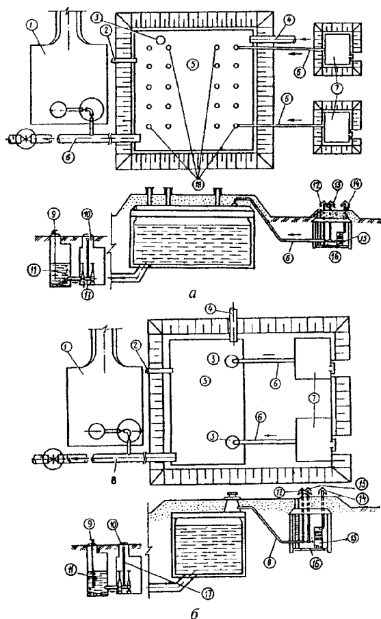
Рис. 8. Устройство герметизированных резервуаров питьевой воды с фильтрами-поглопителями и площадками для сбора воды
