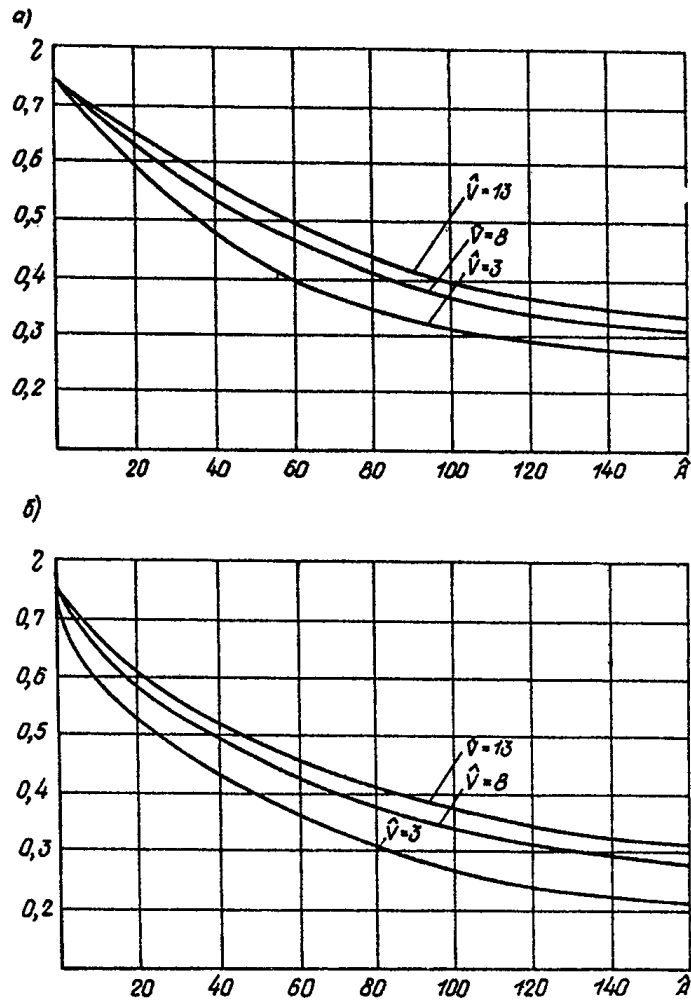
Зависимость сезонного (а) и годового (б) КПД установки солнечного горячего водоснабжения от величин \hat{A} и \hat{V}
