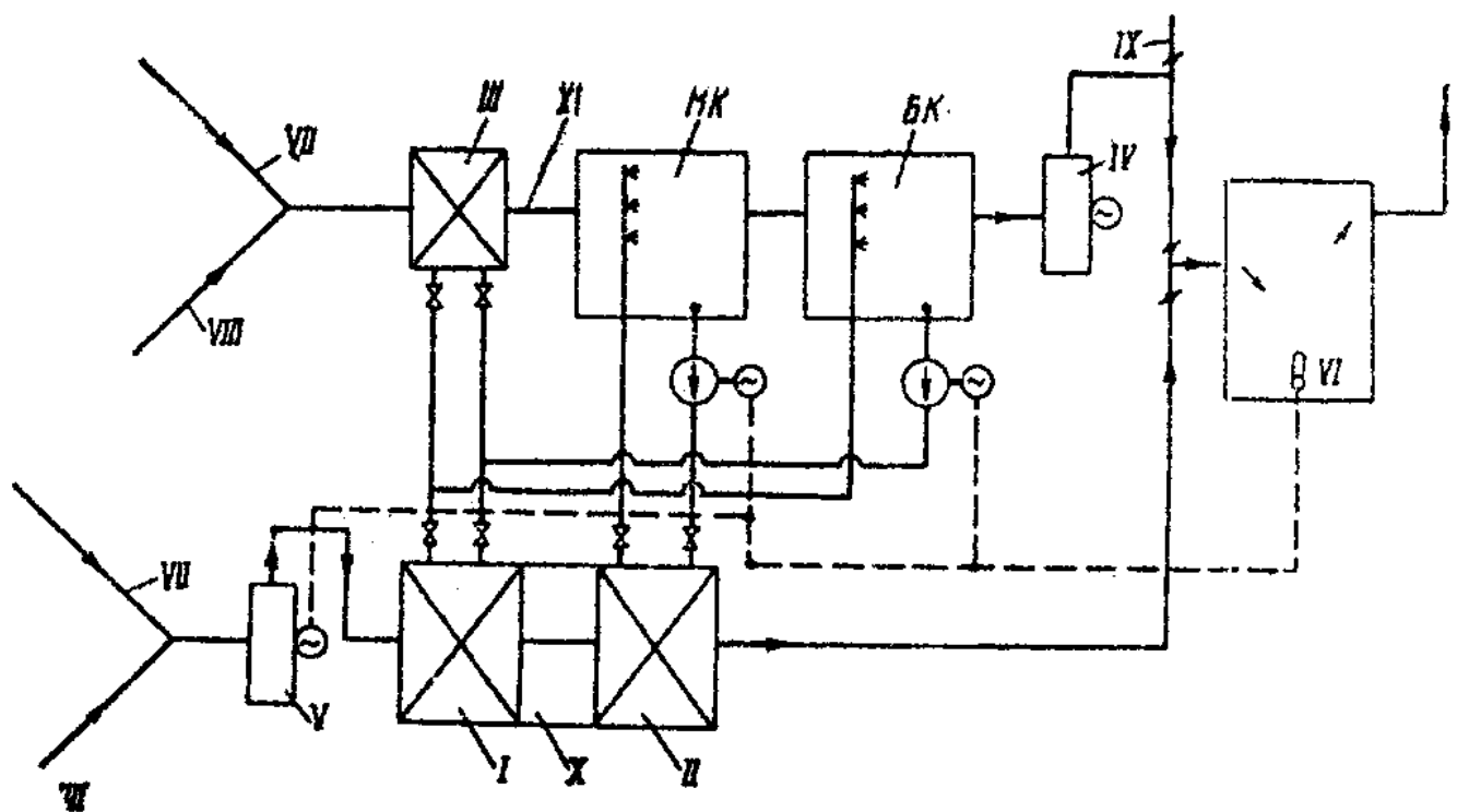
Рис. 7. Принципиальная схема двухпозиционного регулирования компрессорной системы кондиционирования воздуха I, II, III — теплообменники (воздухоохладители); IV, V — соответственно тиляторы испарительного и приточного кондиционеров; VI — датчик тем пературы воздуха в помещении; МК, БК — соответственно оросительные ка малого и большого контуров циркуляции; VII — наружный воздух; VIII — рециркуляционный воздух; IX — выброс в атмосферу воздуха в теплый п года; X — приточный кондиционер; XI — испарительный кондиционер
