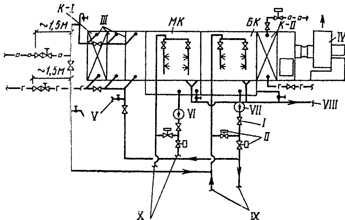
Рис. 3. Схема обвязки трубопроводами испарительного кондиционера
