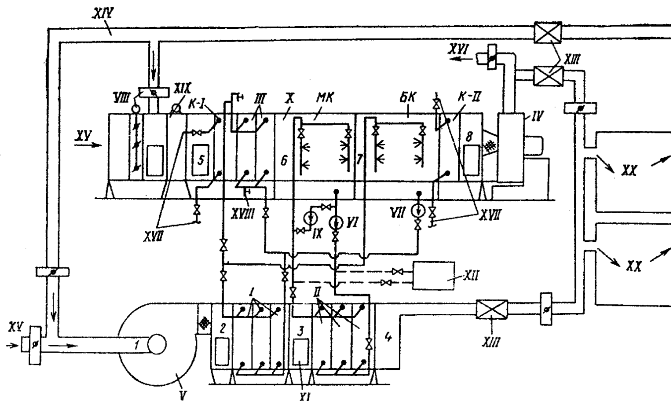
Рис. 1. Рабочая схема двухступенчатой бескомпрессорной системы кондиционирования воздуха. 1, 2, 3, 4 — состояние воздуха при его обработке в приточном кондиционере; 5, 6, 7, 8 — состояние воздуха при его обработке в испарительном кондиционере; I, II, III — теплообменники (воздухоохладители); K-I — теплообменник первого подогрева; МК — оросительная камера малого контура циркуляции; БК — оросительная камера большого контура циркуляции; IV, V — соответственно теплообменники испарительного и приточного кондиционеров; VI, VII — соответственно циркуляционные насосы малого и большого контуров циркуляции; VIII — воздушные заслонки; IX — насос для адиабатического увлажнения воздуха; X — испарительный кондиционер; XI — приточный кондиционер; XII — бак-аккумулятор; XIII — глушитель; XIV — вытяжной или рециркуляционный воздух; XV — наружный воздух; XVI — выброс в атмосферу; XVII — места присоединения к трубопроводам ТЭЦ; XVIII — кран для спуска воды из теплообменников; XIX — фильтр; XX — обслуживаемые помещения.
