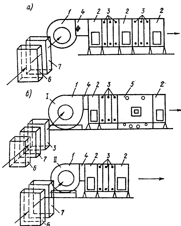
Рис. 5. Типовые компоновки приточных кондиционеров
