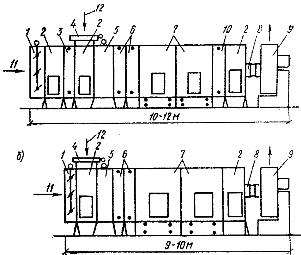
Рис. 4. Типовые компоновки испарительного кондиционера
