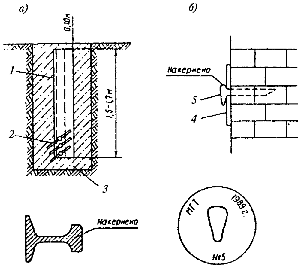
Рис. 2. Образец закрепления точек базисного и магистрального ходов грунтовыми и стенными знаками
