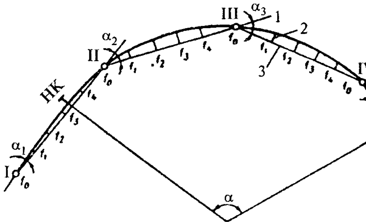
Рис. 2. Схема съемки кривых методом И.В. Гон I—V — стоянки теодолита; 1 — наружный рельс; 2 — ст
