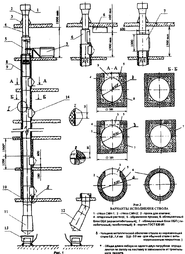
Рис. 1 СХЕМА ВАРИАНТОВ ИСПОЛНЕНИЯ СИСТЕМЫ МУСОРОУДАЛЕНИЯ И ПОЖАРОТУШЕНИЯ ТИПА СМ 1 - дефлектор Д-280; 2 - фланец дефлектора; 3 - фартук Ф-280; 4 - патрубок дефлектора ПД-280; 5 - система прочистки ствола мусоропровода СПСМ-1; 6 - система прочистки ствола мусоропровода СПСМ-2; 7 - система прочистки ствола мусоропровода СПСМ-3; 8 - ствол мусоропровода СМН-1; 9 - ствол мусоропровода СМН-2; 10 - опора ствола ОС-400; 11 - шибер ШМП; 12 - шибер ШМН; 13 - тележка грузовая (контейнер); 14 - клапан навесной КН. Рис. 2 ВАРИАНТЫ ИСПОЛНЕНИЯ СТВОЛА 1 - ствол СМН-1; 2 - ствол СМН-2; 3 - проем для клапана; 4 - кладочный раствор; 5 - обрамление проема; 6 - облицовочный блок ОБК (керамзитобетонный); 7 - облицовочный блок ОБГ (пенобетонный, газобетонный); 8 - кирпич ГОСТ 530-09 8 - толщина металлической оболочки ствола из нержавеющей стали 0,8...1,4 мм (0,8-3,0 мм - для обычной стали с антикоррозионным покрытием.) * - Общая длина набора из одного-двух патрубков определяется по заказу на поставку в зависимости от тротильного проекта.
