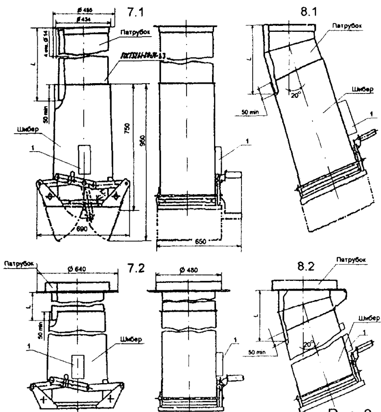
Рис.7 Шибер типа ШМП
