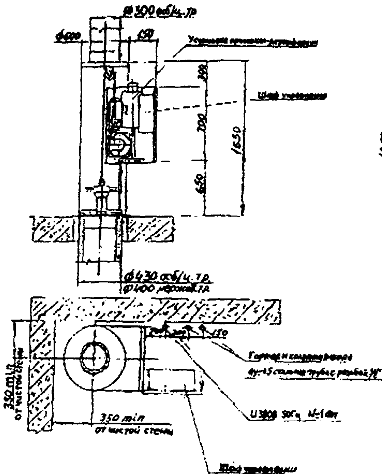
Вариант установки с встраиваемым шкафом управления.
