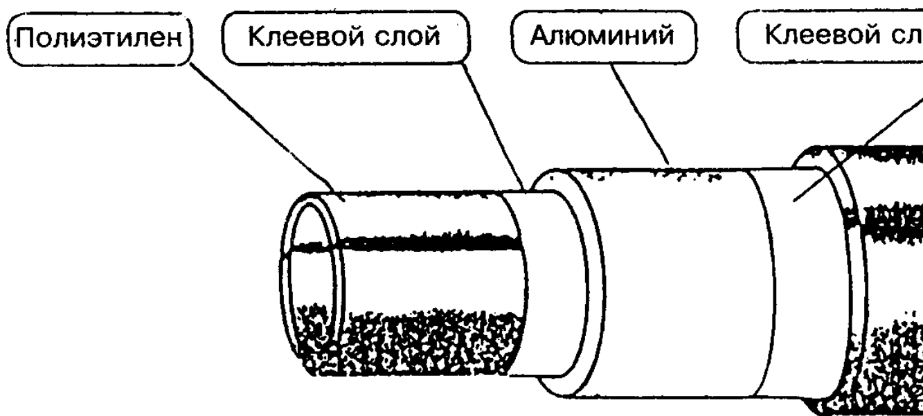
Рисунок 1 — Структура металлополимерной трубы
