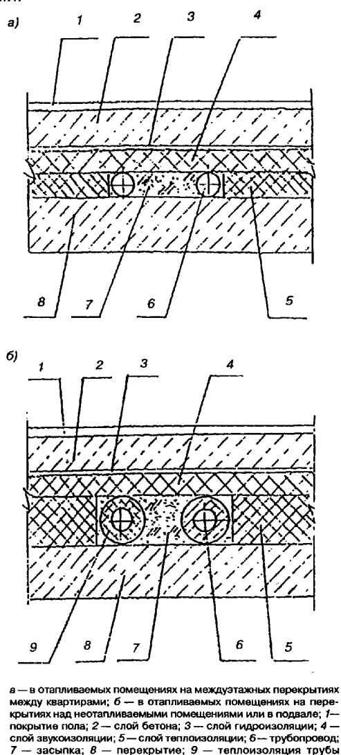
Рисунок 14 — Скрытая прокладка разводящих трубопроводов из металлополимерных труб в полу
