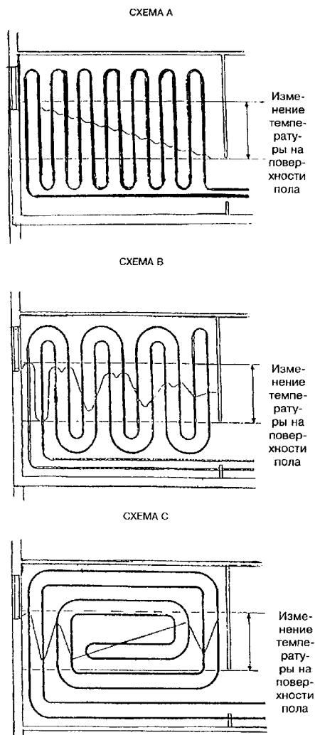
Рисунок 2 — Схемы укладки труб в системах напольного отопления и графики изменения температуры на поверхности пола
