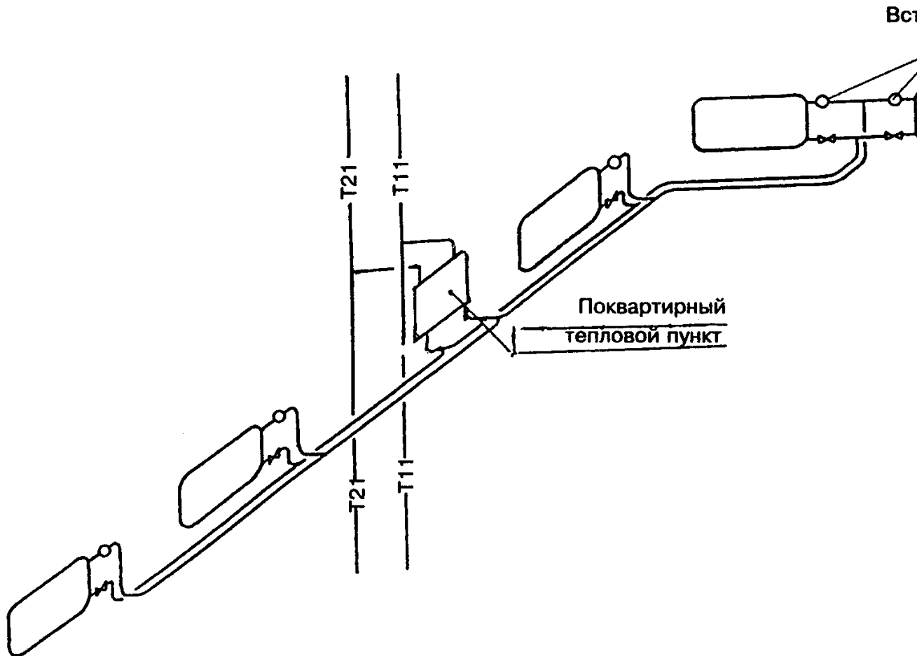
Рисунок 4 — Система отопления с горизонтальными двухтрубными ветками для группы параллельно-последовательно соединенных отопительных приборов
