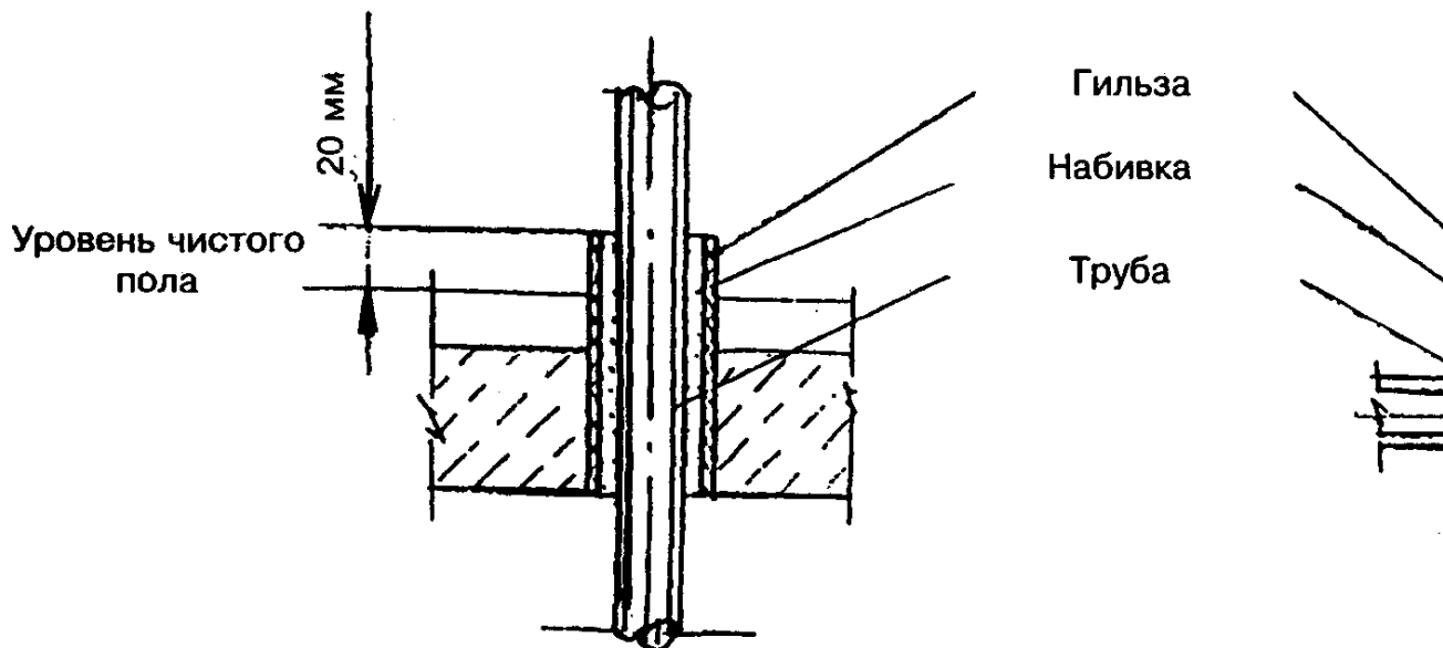
Рисунок 15 — Установка гильзы для прокладки труб в стенах и перекрытиях
