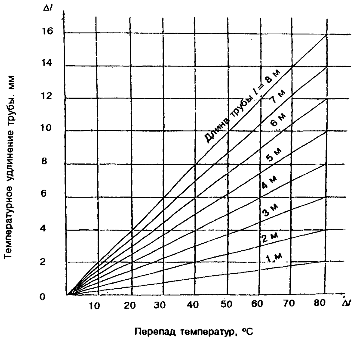
Рисунок 10 — Диаграмма для определения удлинения труб
