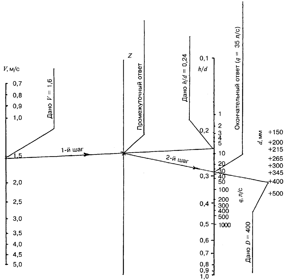
Рисунок В.1 — Номограмма для выбора диаметра d стеклопластиковых труб в зависимости от расхода q , скорости V и наполнения \frac{h}{d} для самотечного канализационного трубопровода ( Z — промежуточная шкала)
