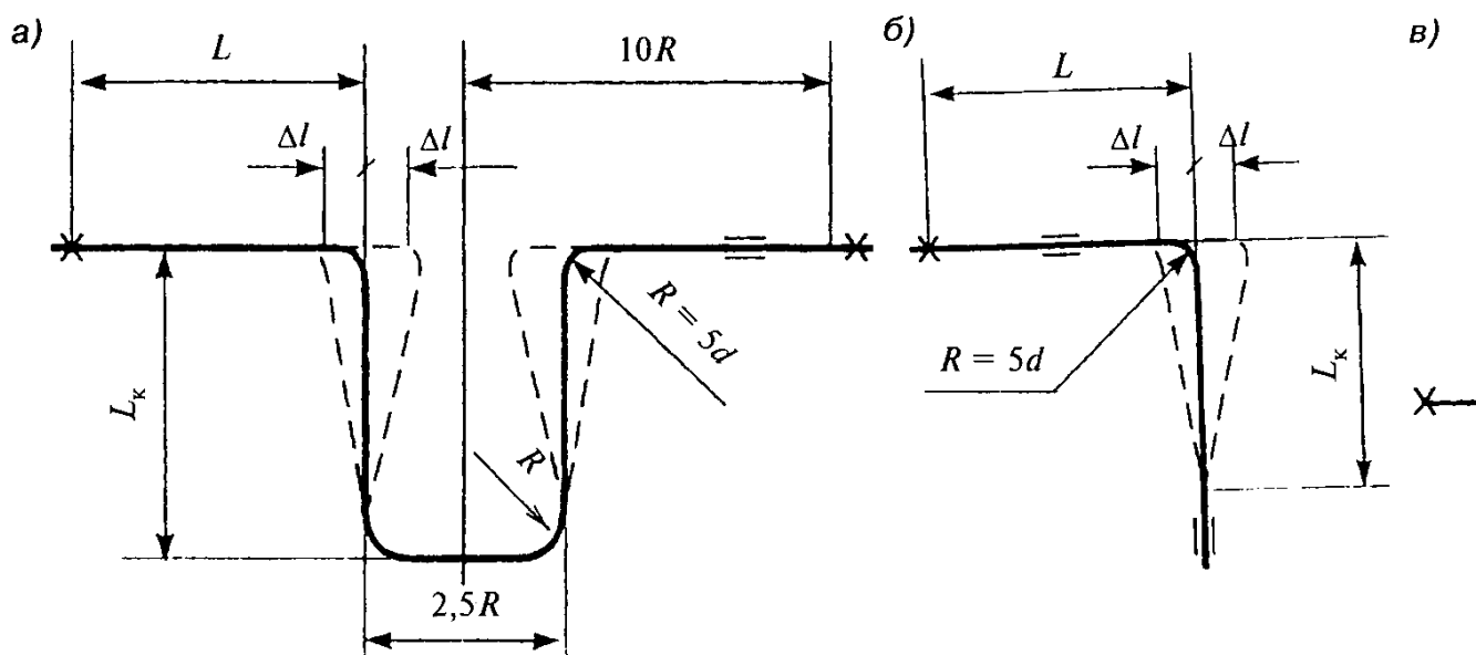
Рисунок 5 — Устройство компенсаторов П-образного (а), Г-образного (б), петлеобразного (в)
