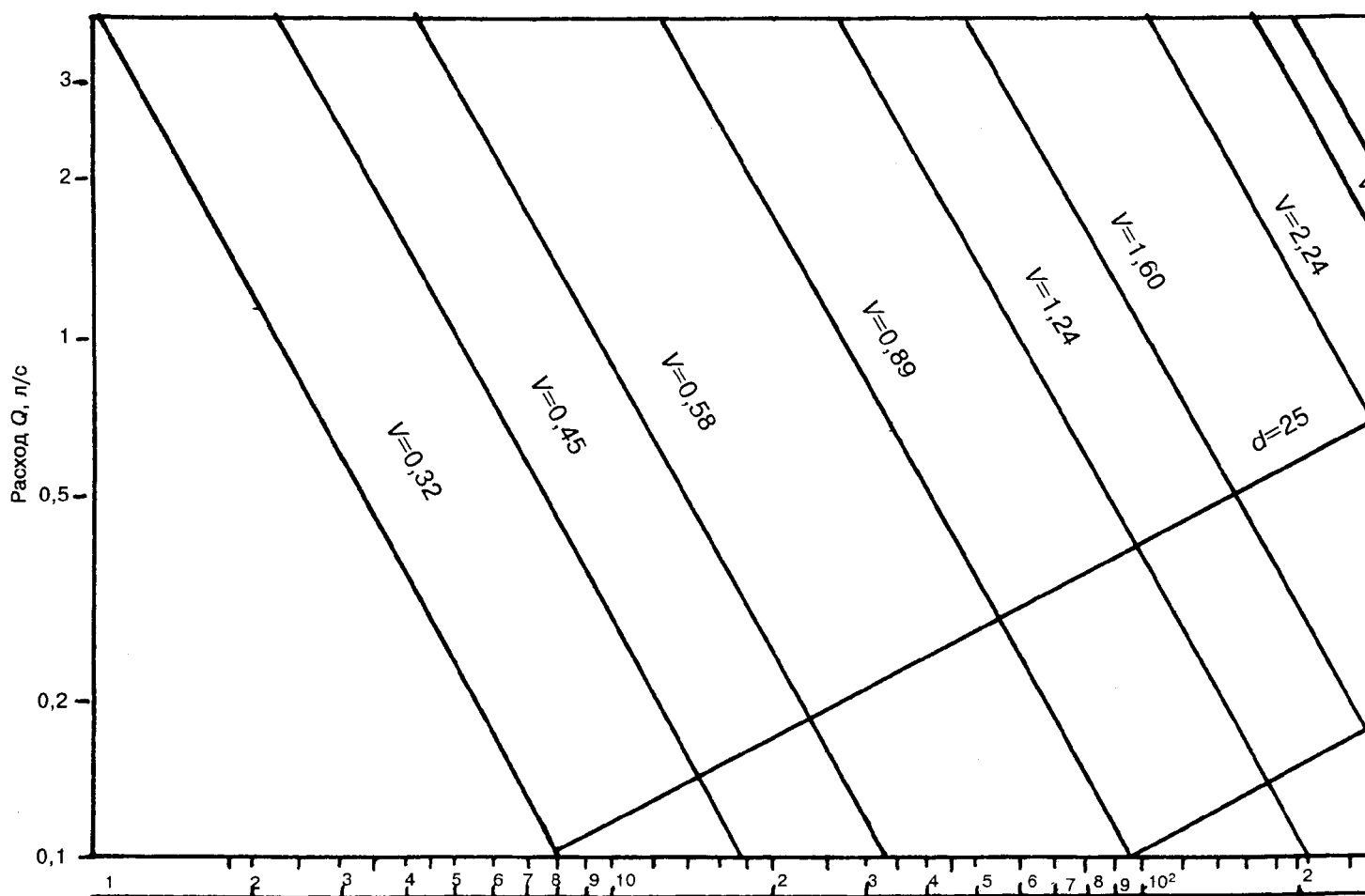
"Рисунок А.1 - Номограмма для приближенного гидравлического расчета водопровода холодной воды из металлополимерных труб по ТУ 2248-001-07629379-96"
