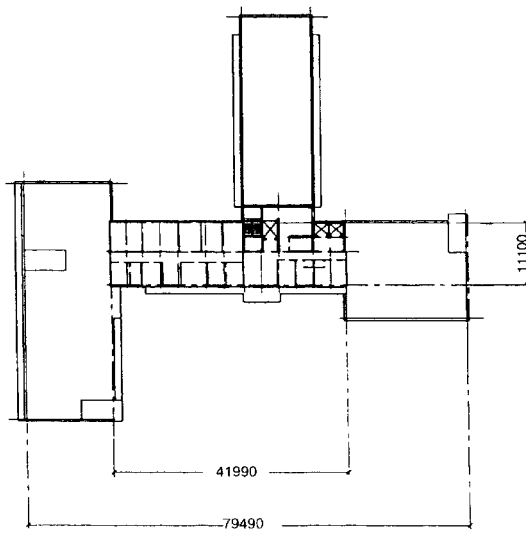
План надстроенного 3-го этажа
