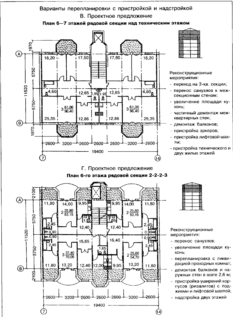
"Рисунок Б.11, а. Реконструкция и модернизация жилых домов серии 1-464"
