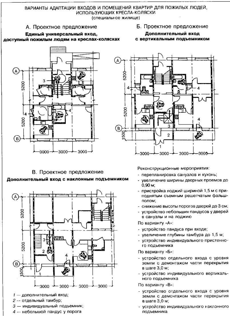
"Рисунок Б.13. Реконструкция и модернизация жилых домов серии 1-468"
