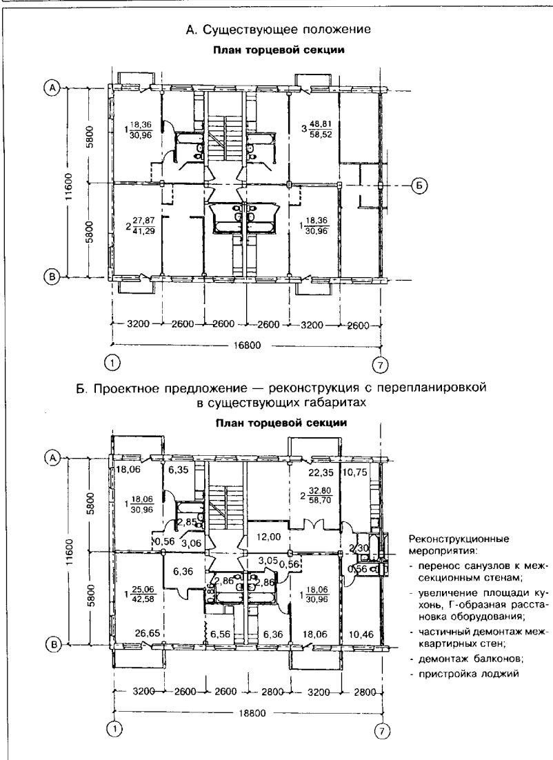
"Рисунок Б.2. Реконструкция и модернизация жилых домов серии 1-335"
