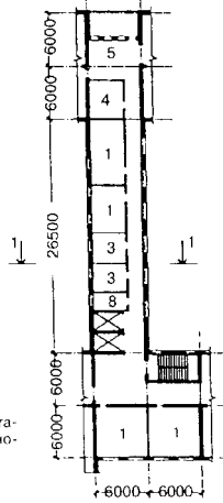
Фрагмент плана 3-го этажа
