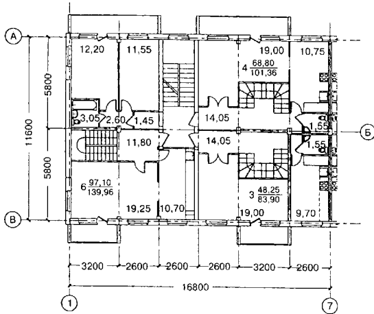
Г. Проектное предложение — план надстройки 6-го этажа
