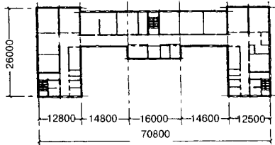
План 2-го этажа
