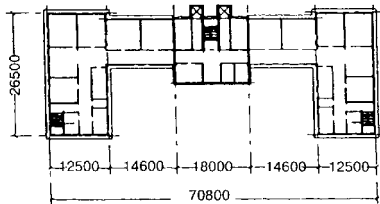
План 3-го надстраиваемого этажа
