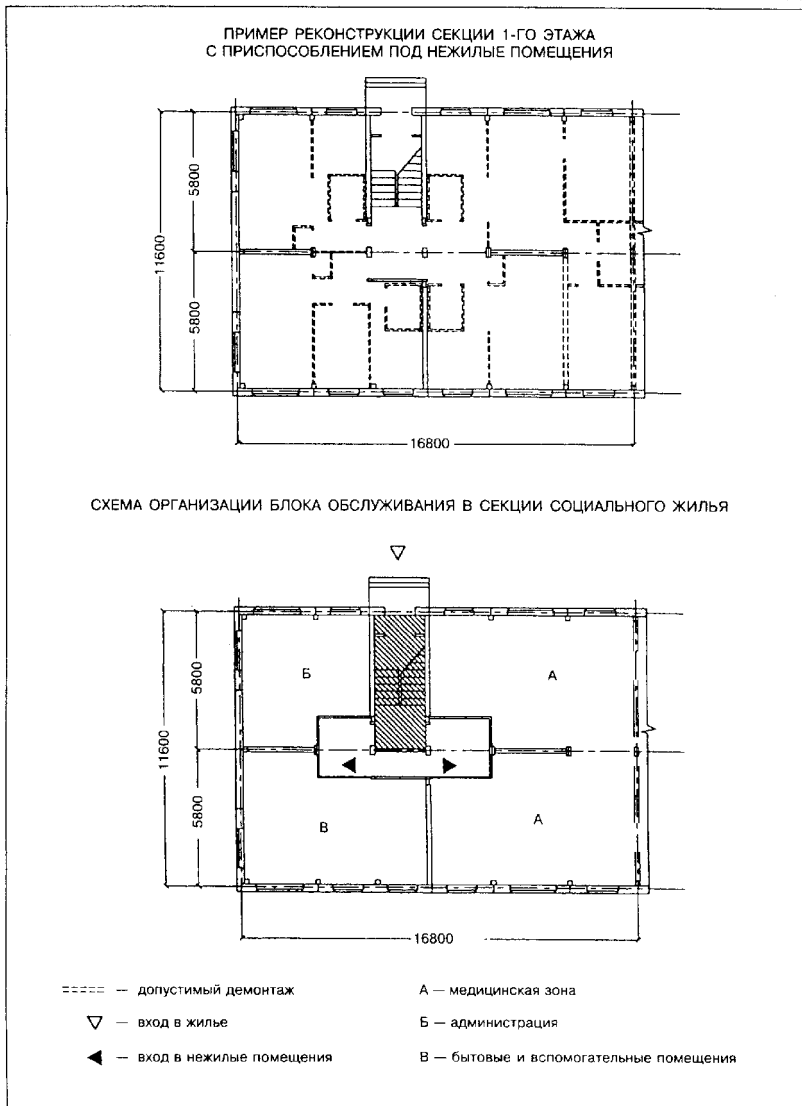
"Рисунок Б.6. Реконструкция и модернизация жилых домов массовых серий 1-335"
