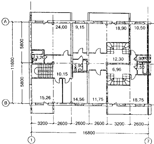
Г. Проектное предложение — план надстройки 6-го этажа
