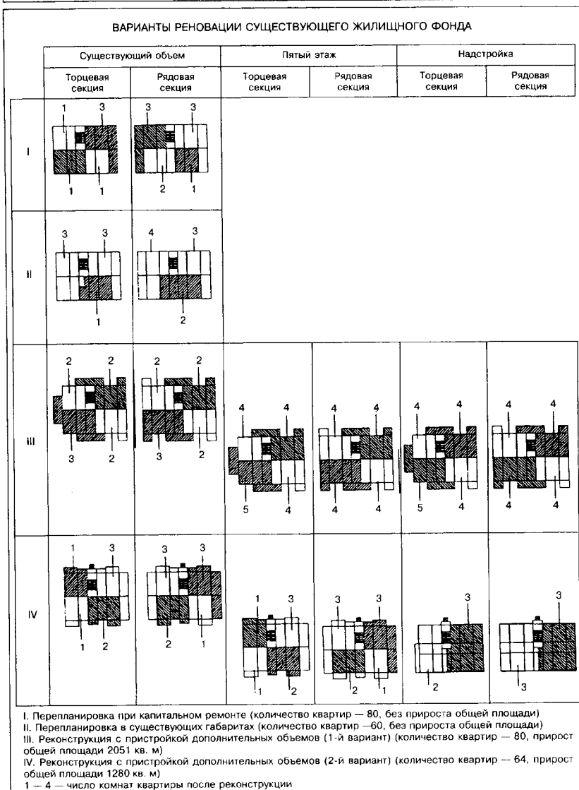
"Рисунок Б.9. Реконструкция и модернизация жилых домов серии 1-464"
