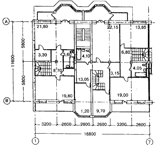
"Рисунок Б.5. Реконструкция и модернизация жилых домов серии 1-335"
