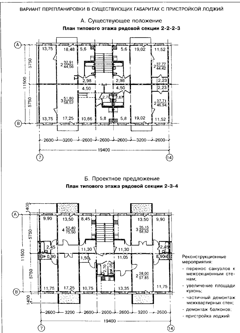
"Рисунок Б.10. Реконструкция и модернизация жилых домов серии 1-464"
