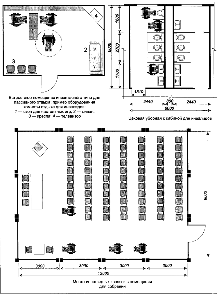
"Рис. 5. Помещения социального обслуживания"
