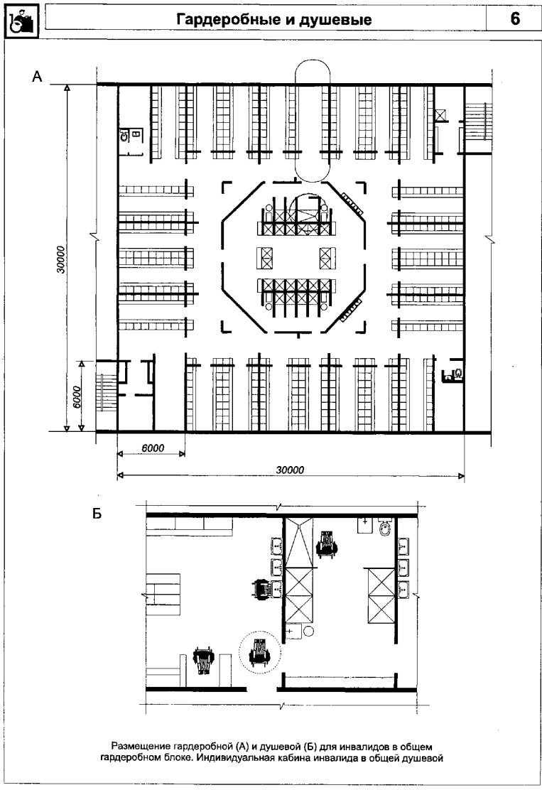
"Рис. 6. Гардеробные и душевые"
