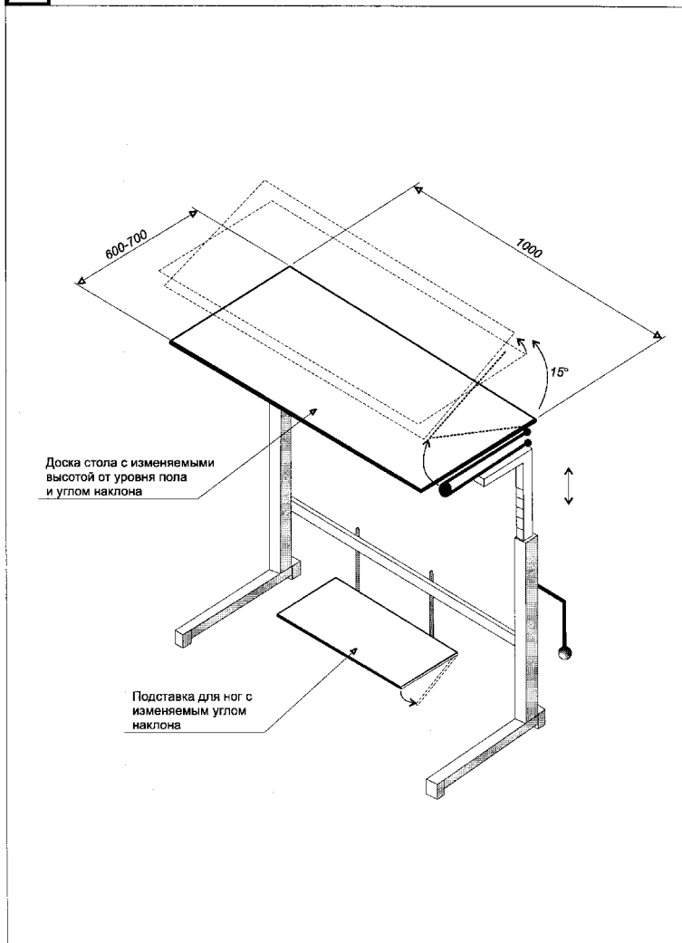
"Рис. 12. Трансформируемый рабочий стол для инвалида"
