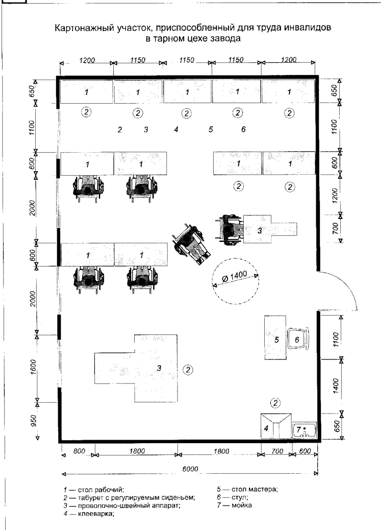
"Рис. 11. Пример планировки помещения"
