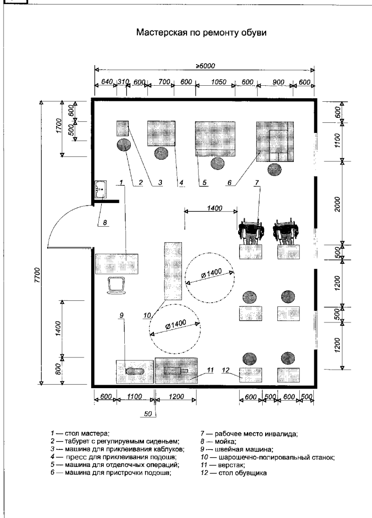
"Рис. 8. Пример планировки помещения"
