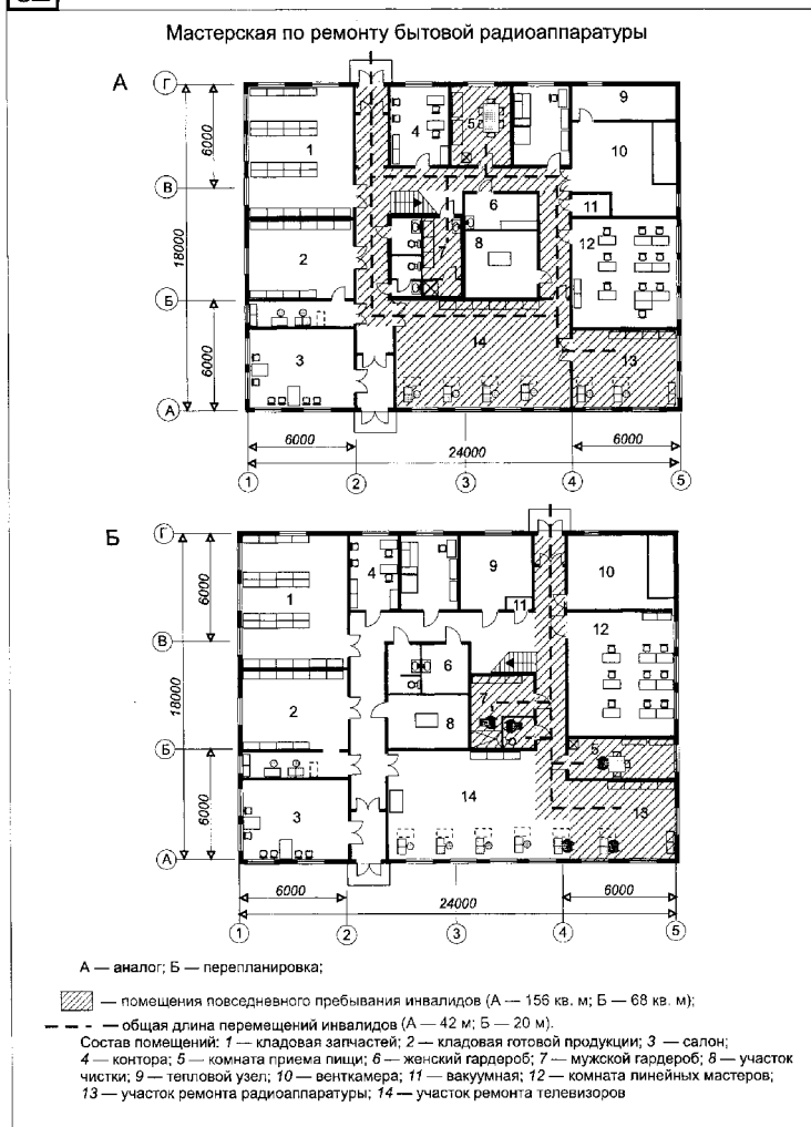
"Рис. 4. Адаптация здания для инвалидов"
