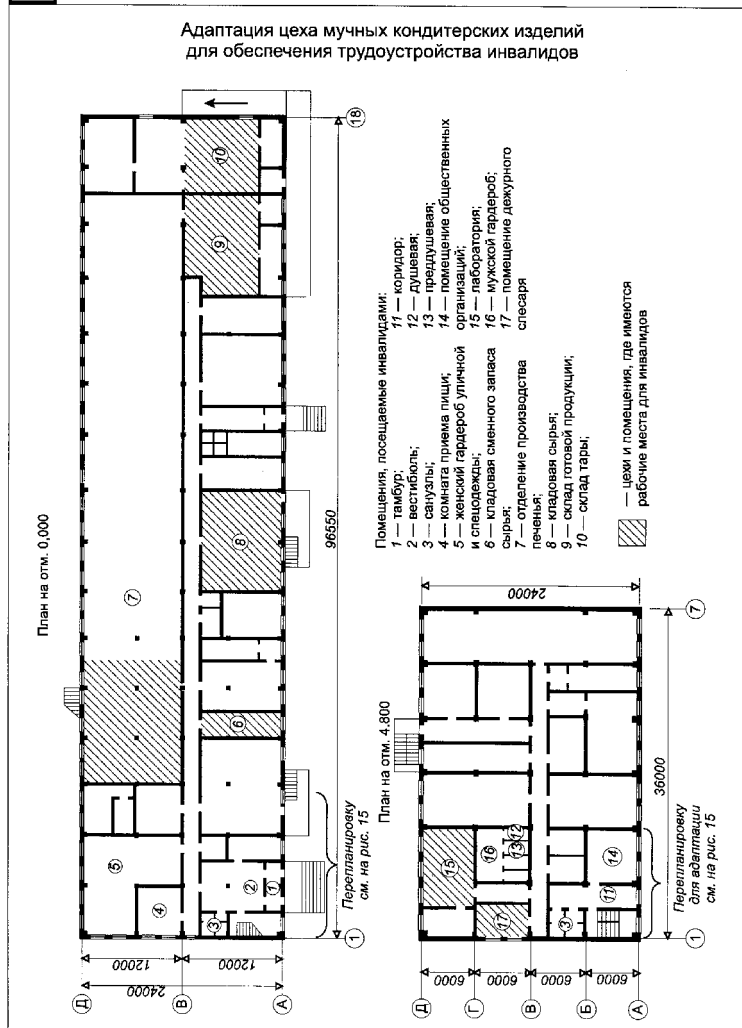
"Рис. 14. Адаптация здания для инвалидов"
