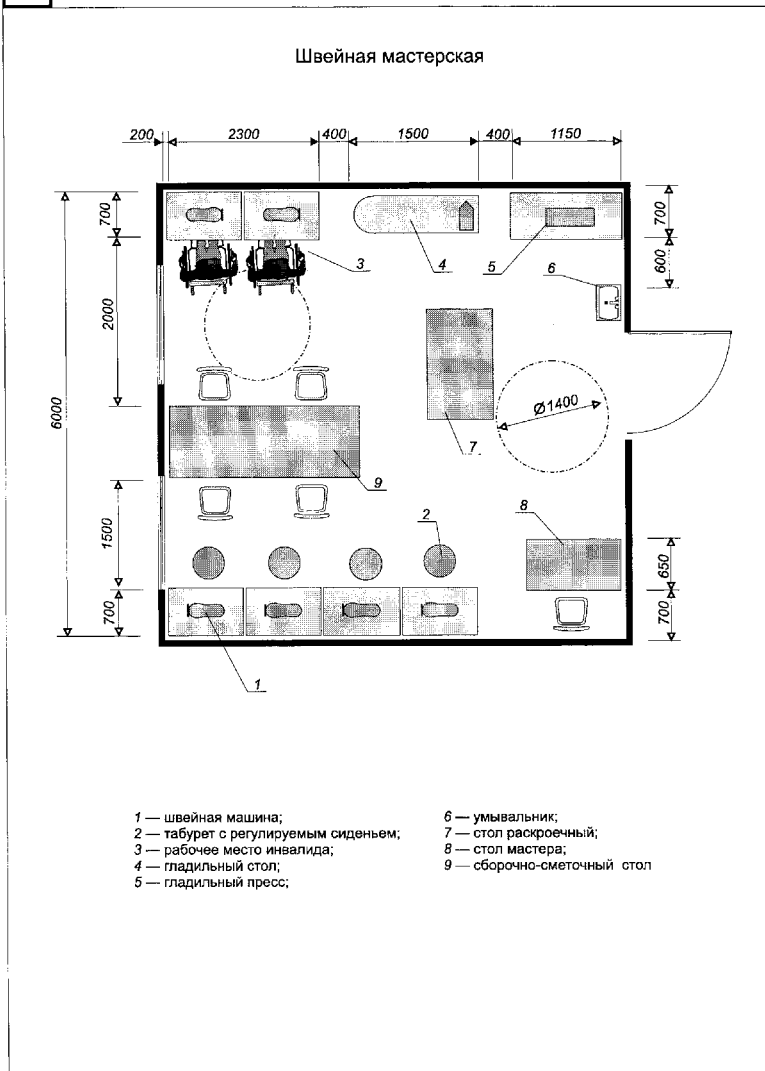
"Рис. 10. Пример планировки помещения"
