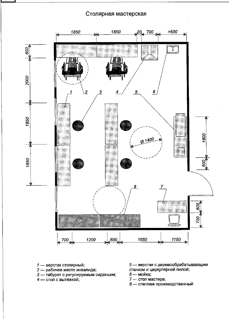
"Рис. 7. Пример планировки помещения"
