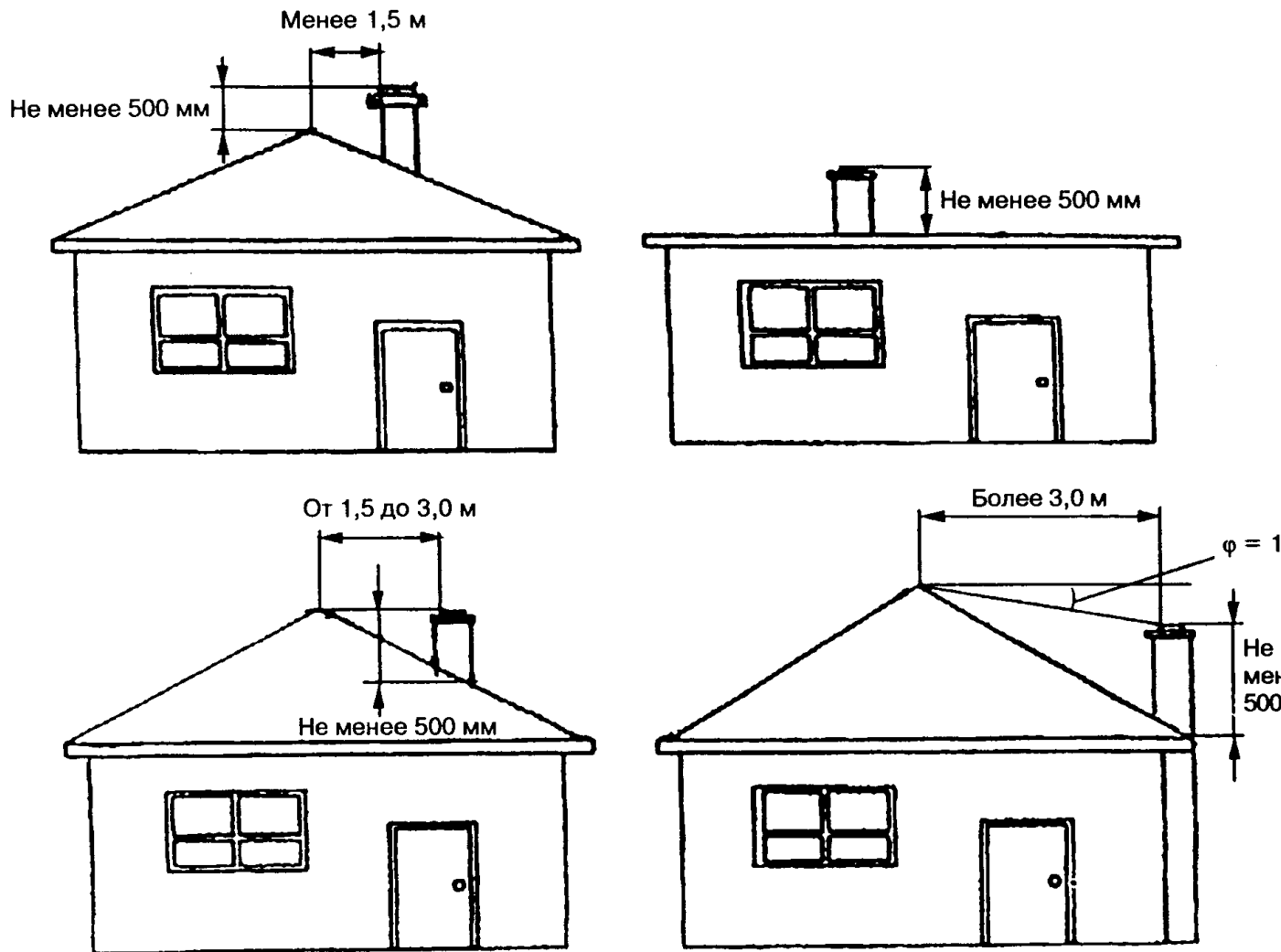
Рисунок 7.9 — Минимальная высота дымовой трубы
