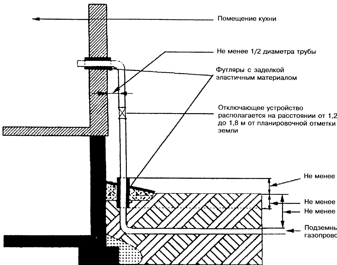
Рисунок 9.1 — Газовый ввод
