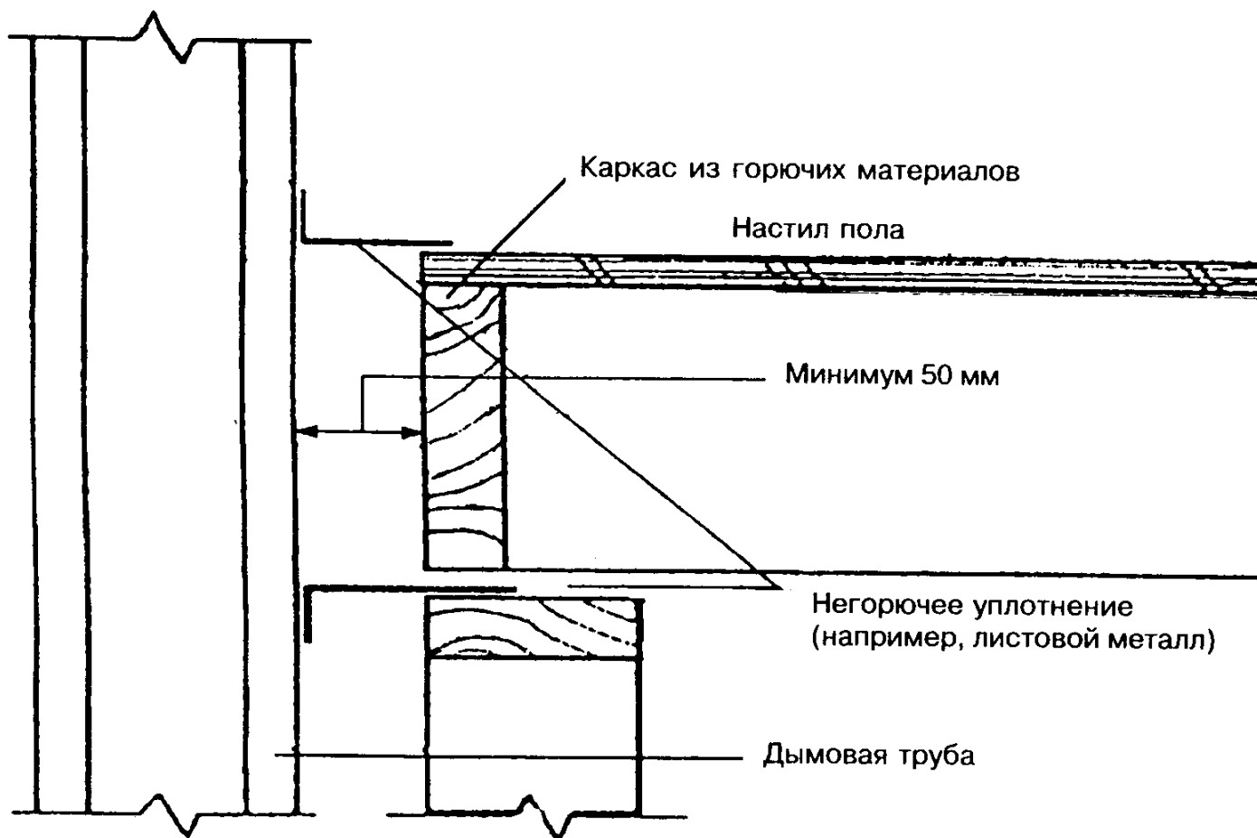
Рисунок 7.8 — Расстояние от дымовой трубы до строительных конс
