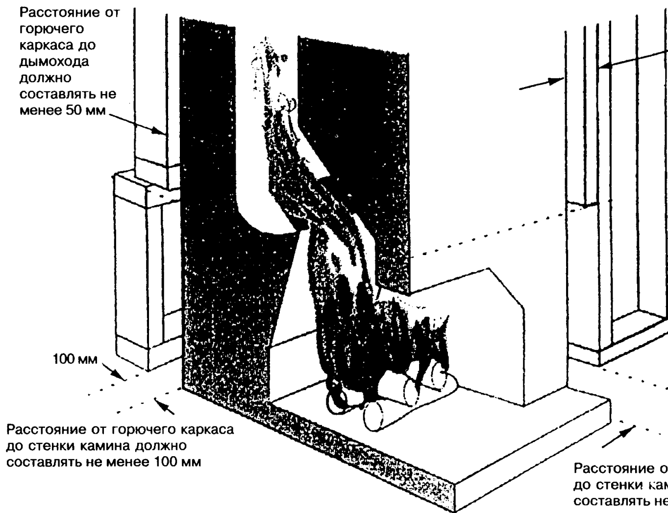
Рисунок 7.4 — Зазоры между камином и каркасом из горючих матери
