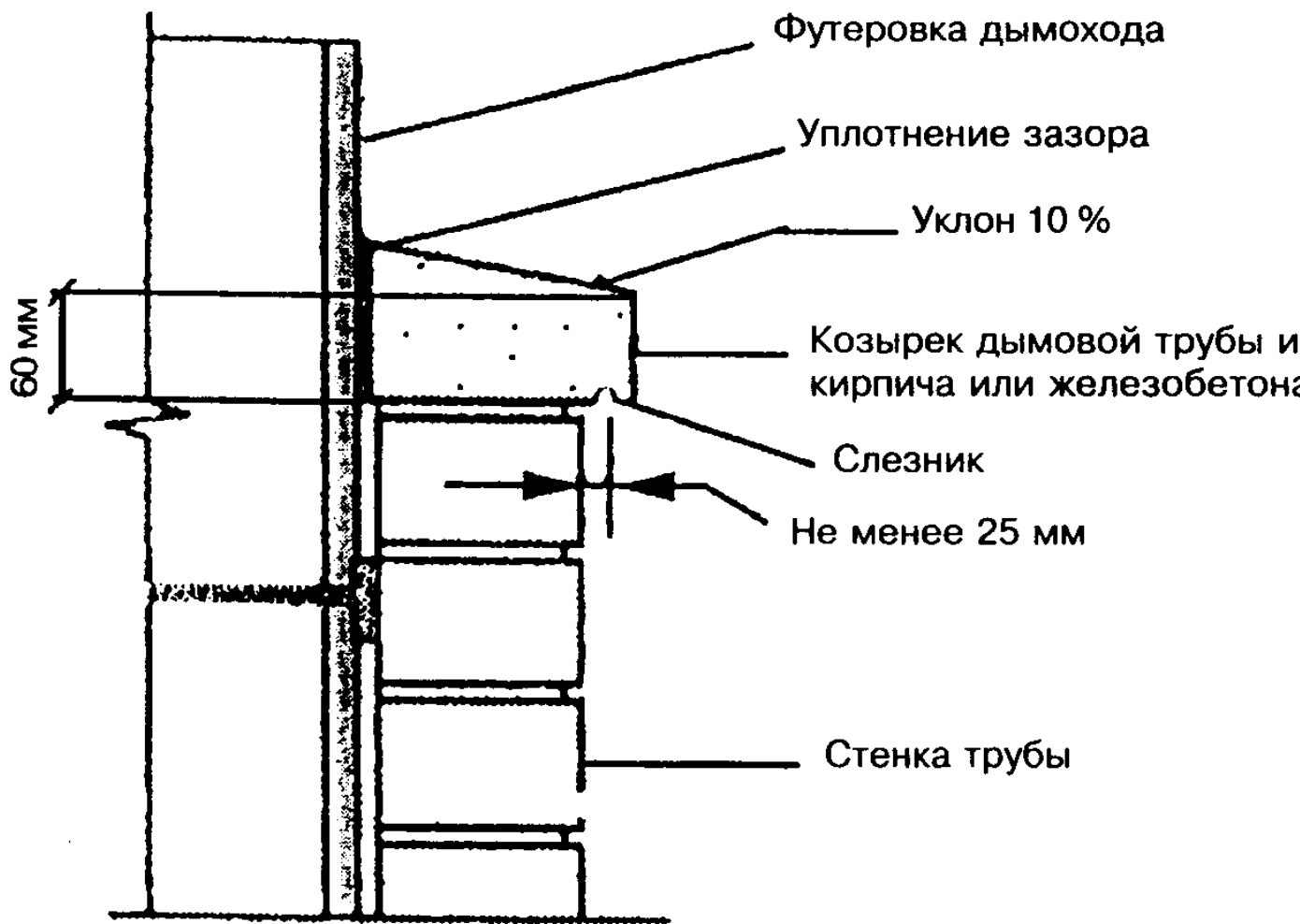
Рисунок 7.7 — Оголовок дымовой трубы
