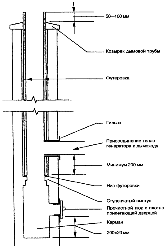
Рисунок 7.6 — Облицовка дымохода
