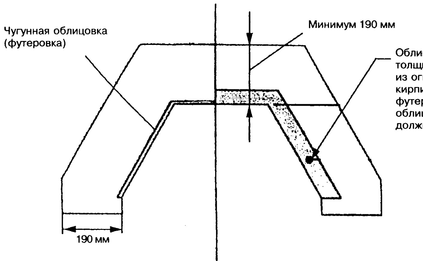
Рисунок 7.5 — Футеровка камина
