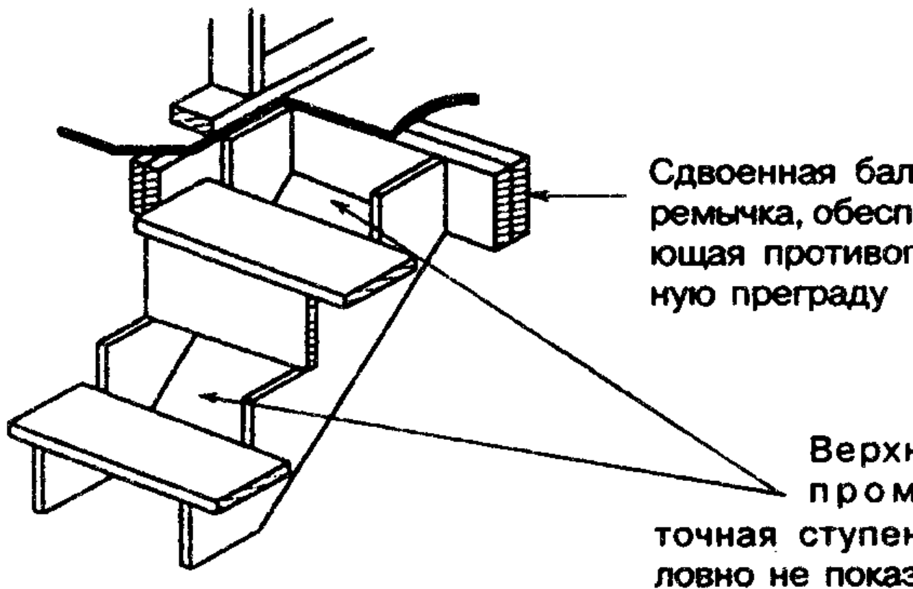
Рисунок 12-2 — Противопожарная преграда в лестничном проеме
