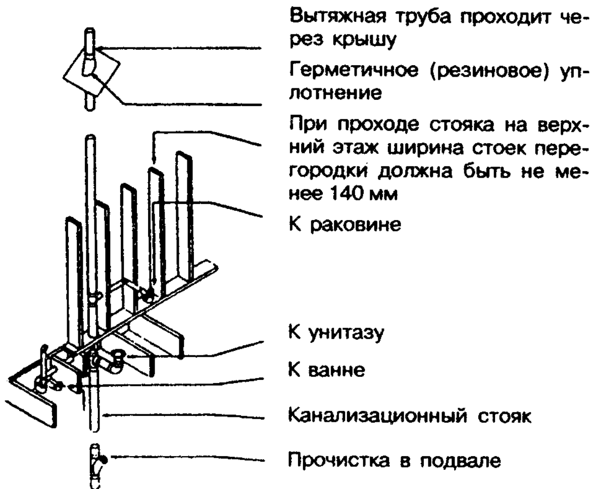
Рисунок 13-8 — Прокладка канализационных труб в каркасе дома
