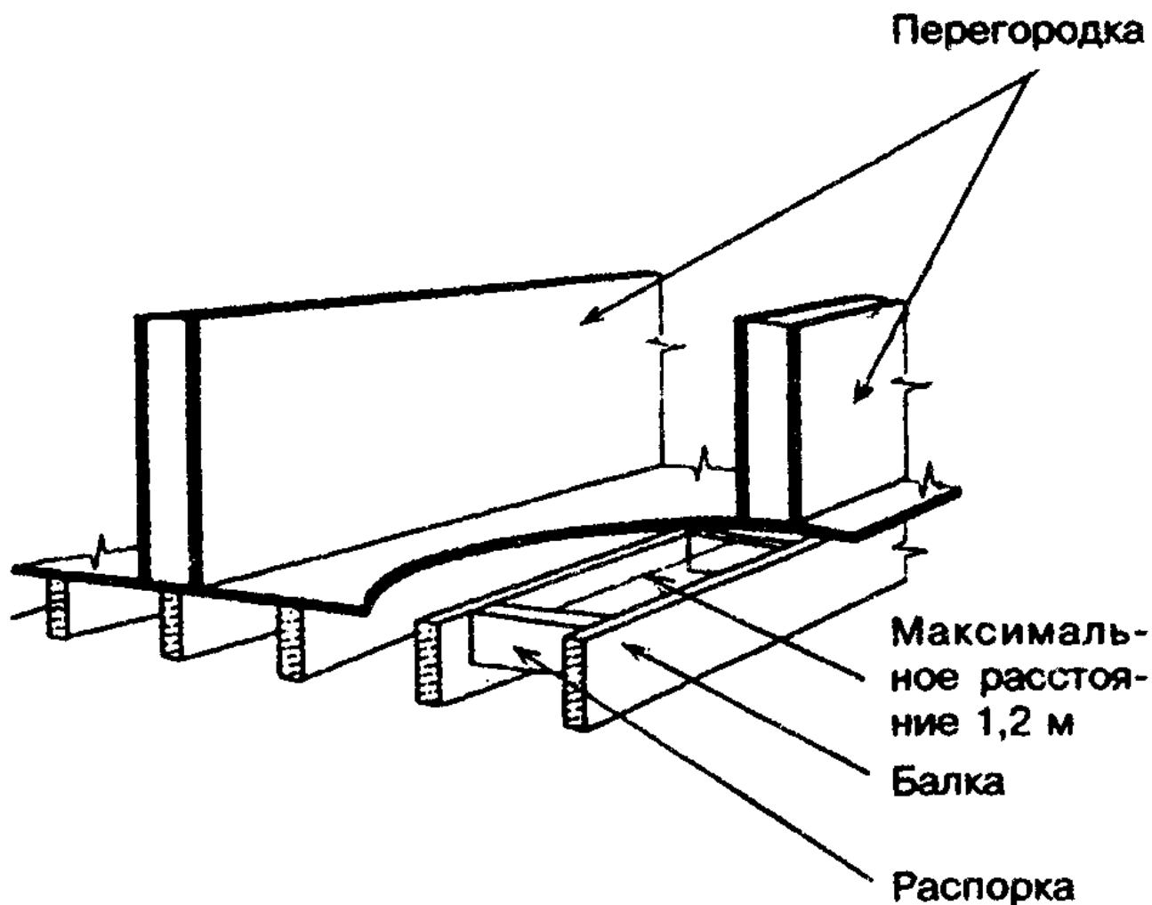
Рисунок 6-13 — Опираие перегородок
