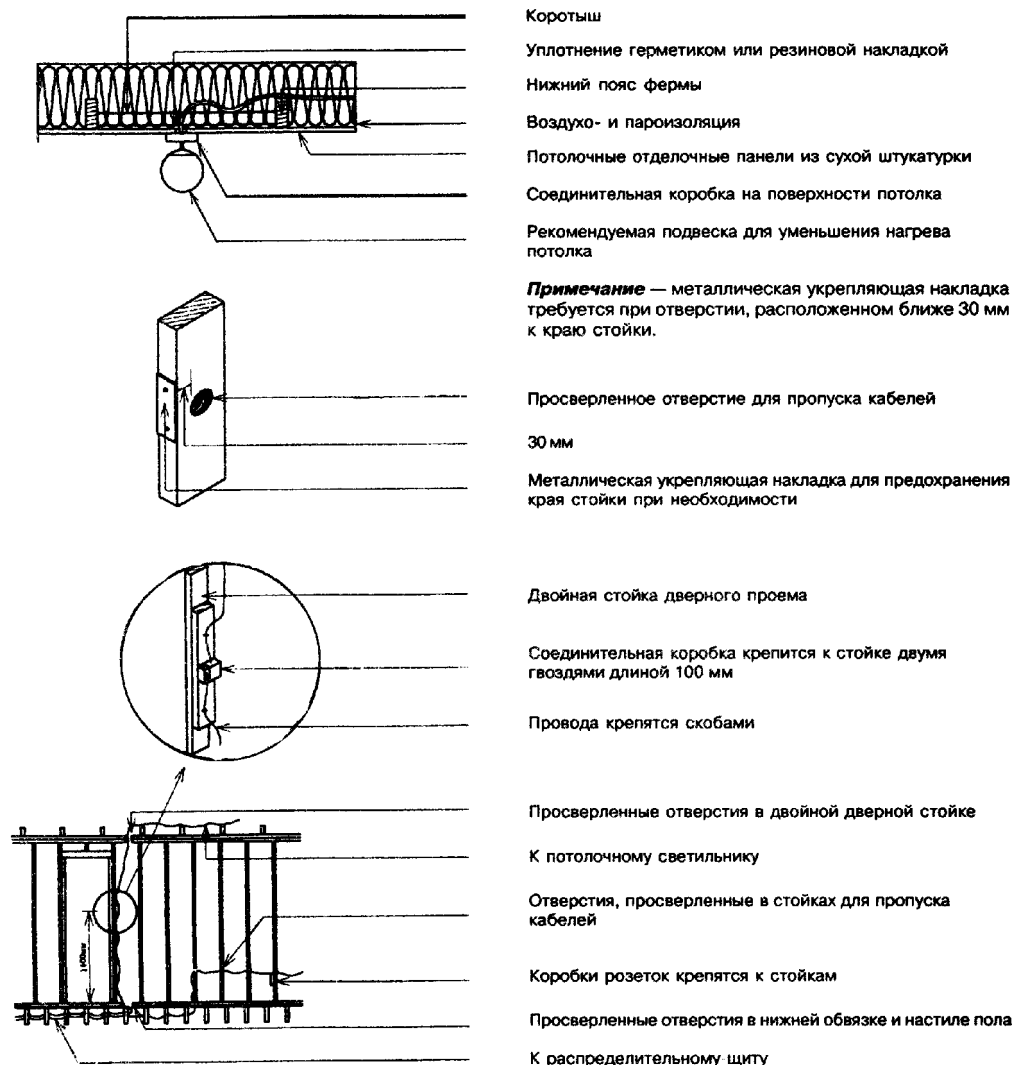
Рисунок 13-9 — Прокладка электрических проводов в элементах каркаса
