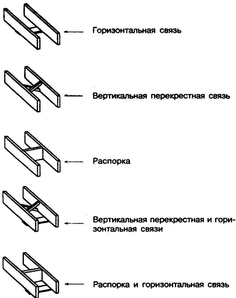
Рисунок 6-10 — Способы раскрепления балок
