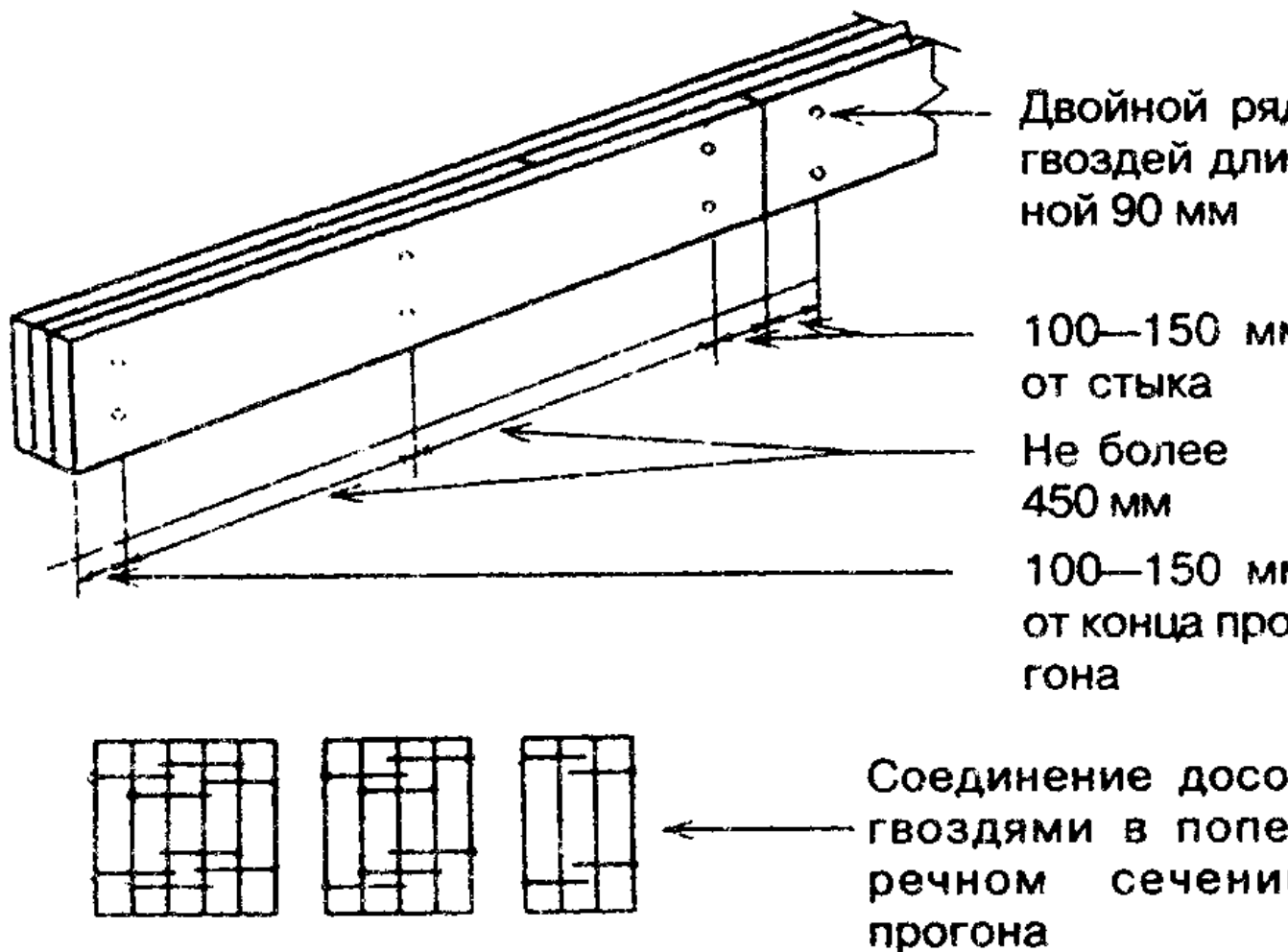
Рисунок 6-1 — Деревянные прогоны составного сечения
