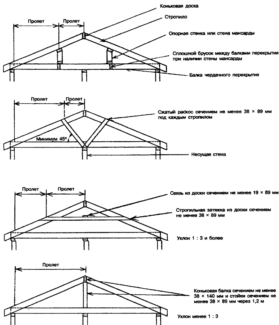
Рисунок 8-1 — Элементы несущего каркаса скатной крыши
