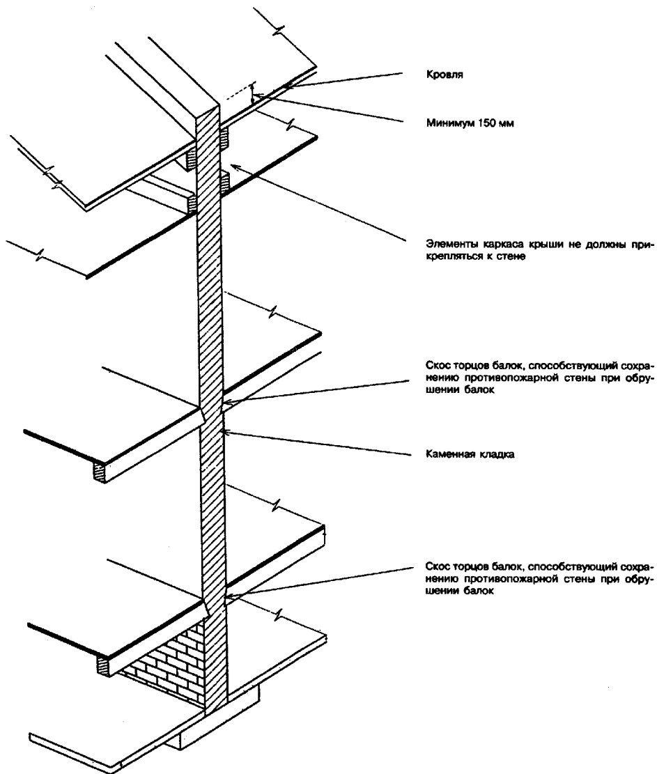
Рисунок 7-5 — Каменная противопожарная стена
