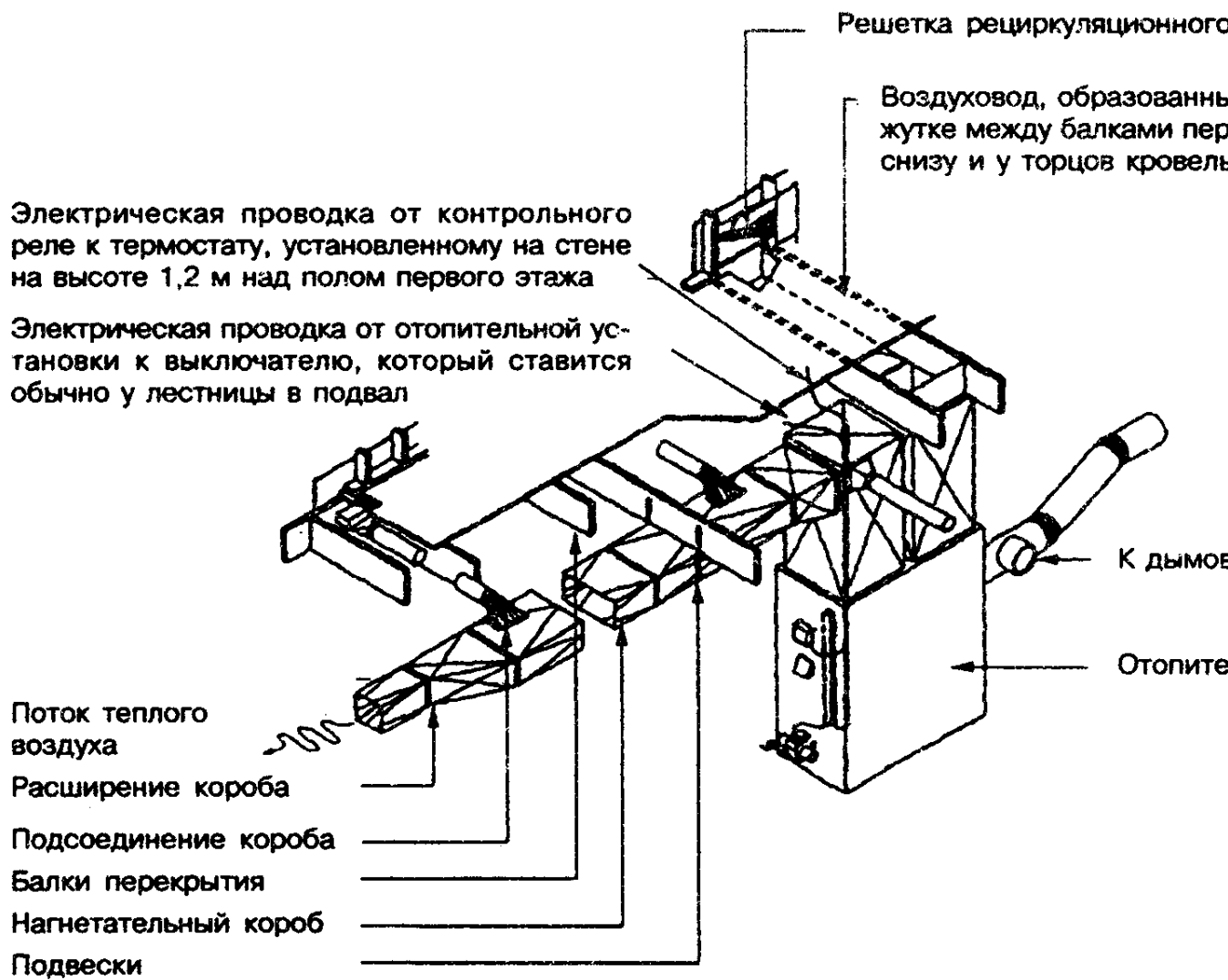
Рисунок 13-4 — Крепление воздуховодов
