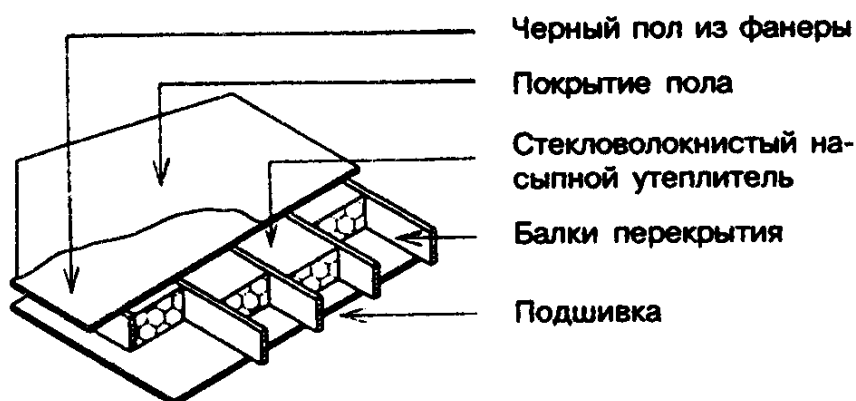
Рисунок 9-3 — Утепление перекрытий над неотапливаемыми помещениями
