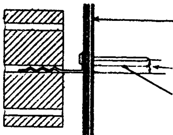
Рисунок 10-1 — Анкеры в каменной облицовке
