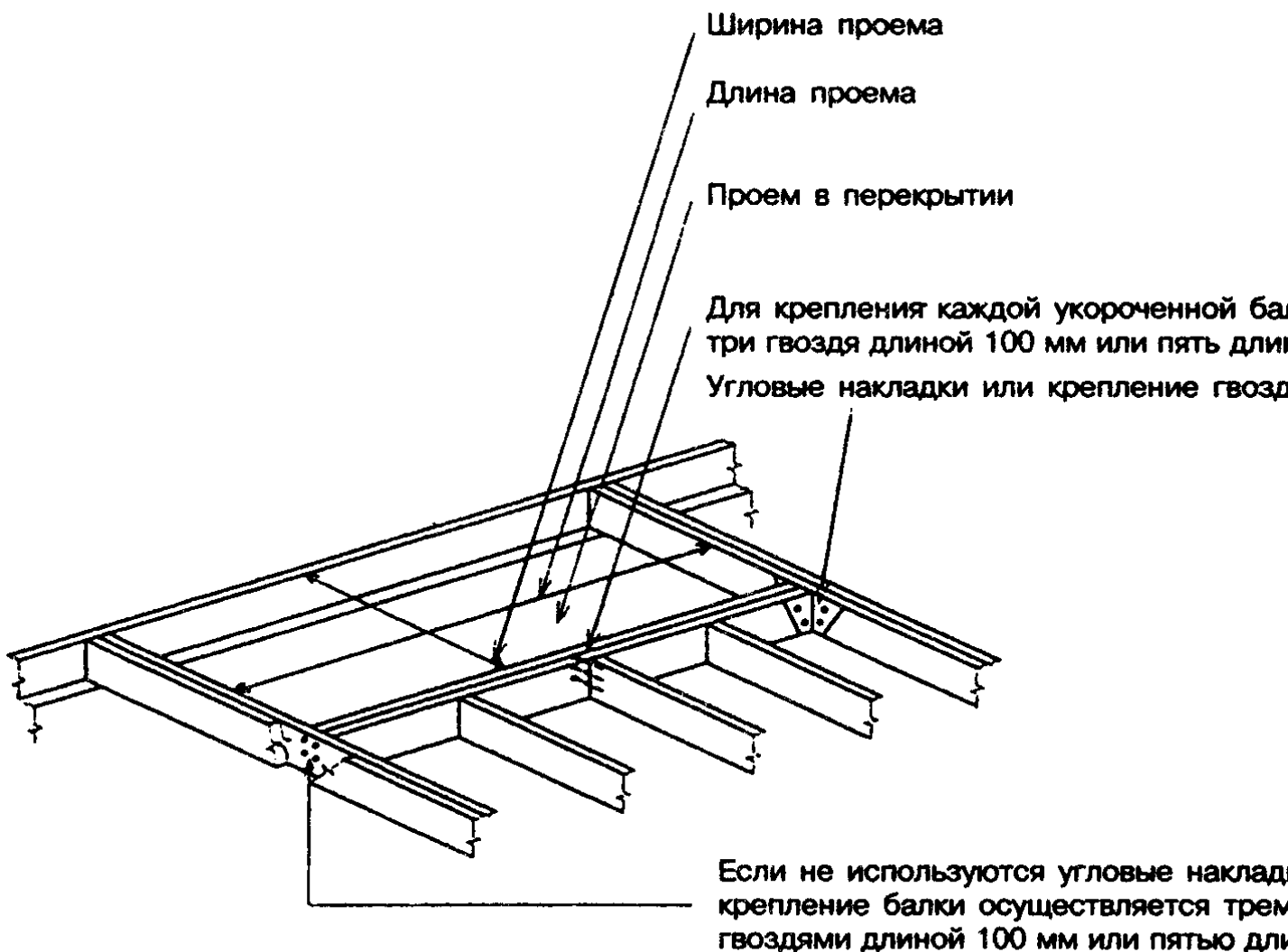
Рисунок 6-12 — Устройство проемов в перекрытии
