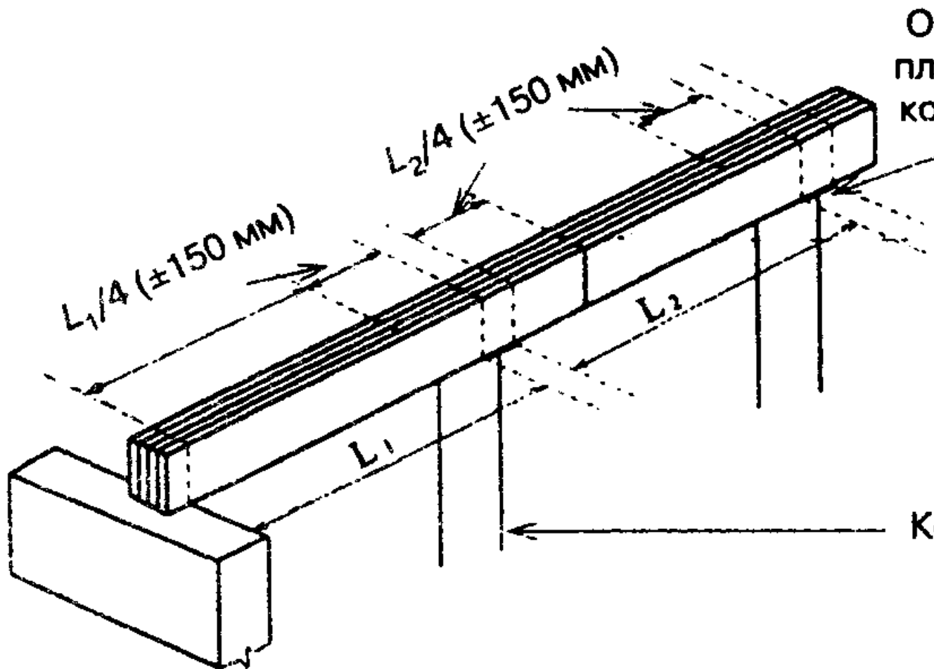
Рисунок 6-2 — Стыки досок в неразрезных прогонах составного сечения
