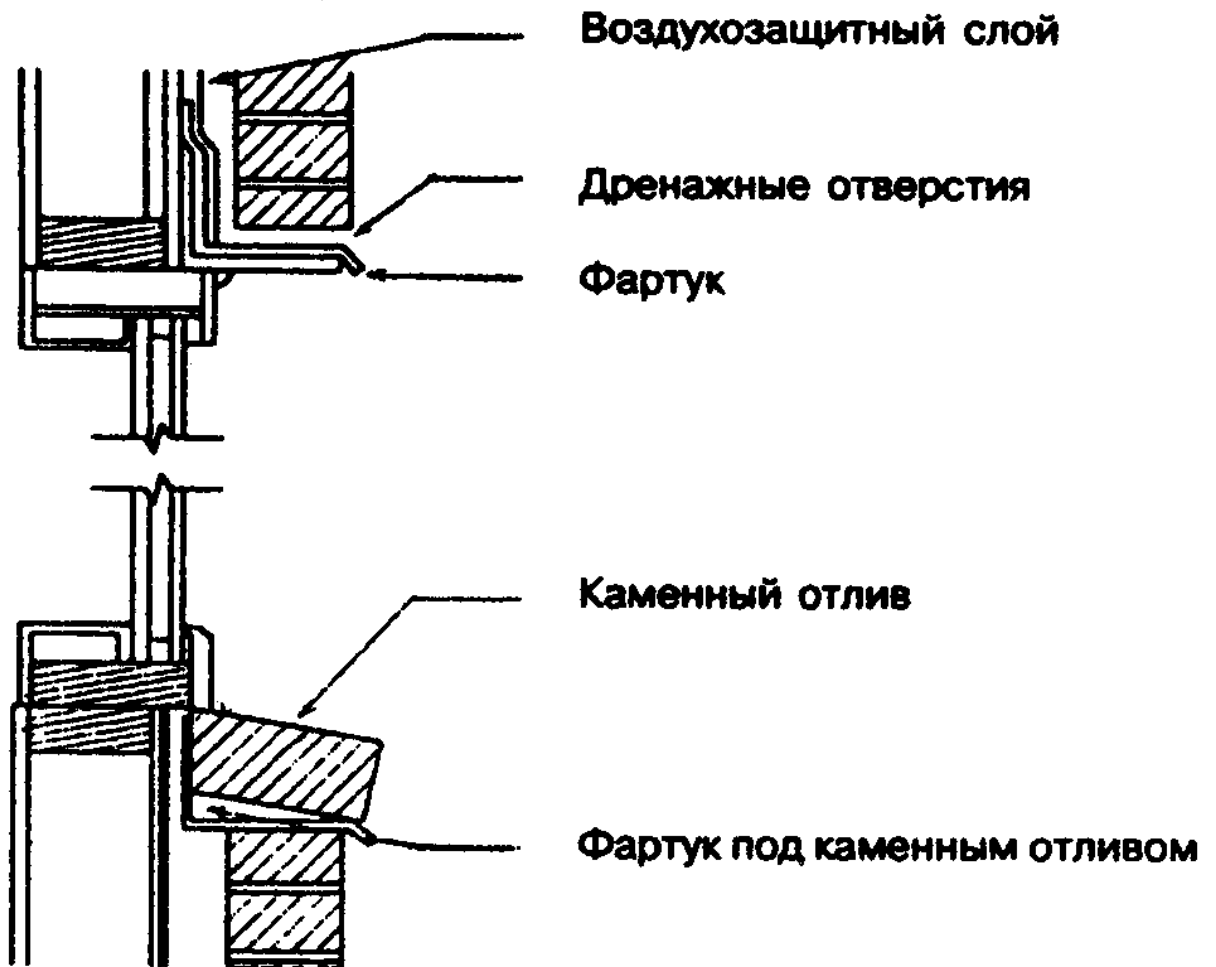
Рисунок 10-2 — Установка фартука под каменным отливом
