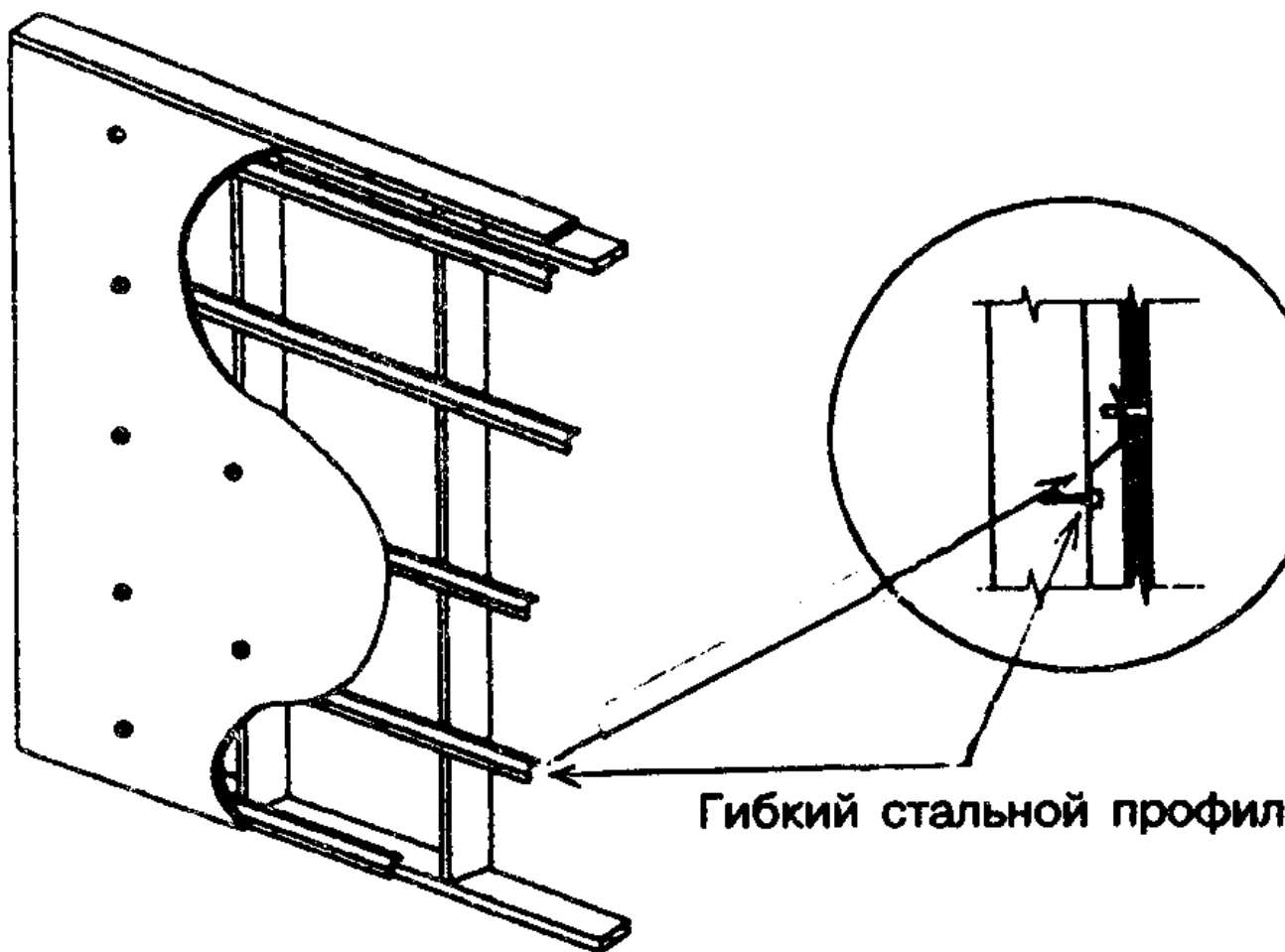
Рисунок 7-8 — Крепление обшивки каркаса для обеспечения звукоизоляции
