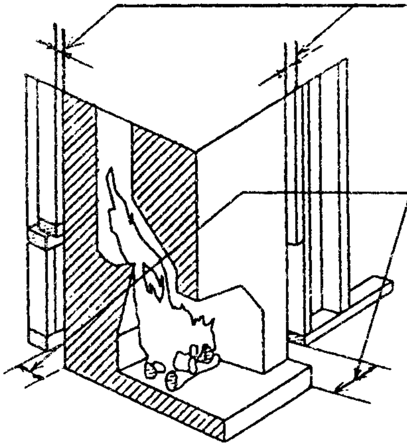
Рисунок 13-2 — Расстояние от стенок камина до каркаса здания
