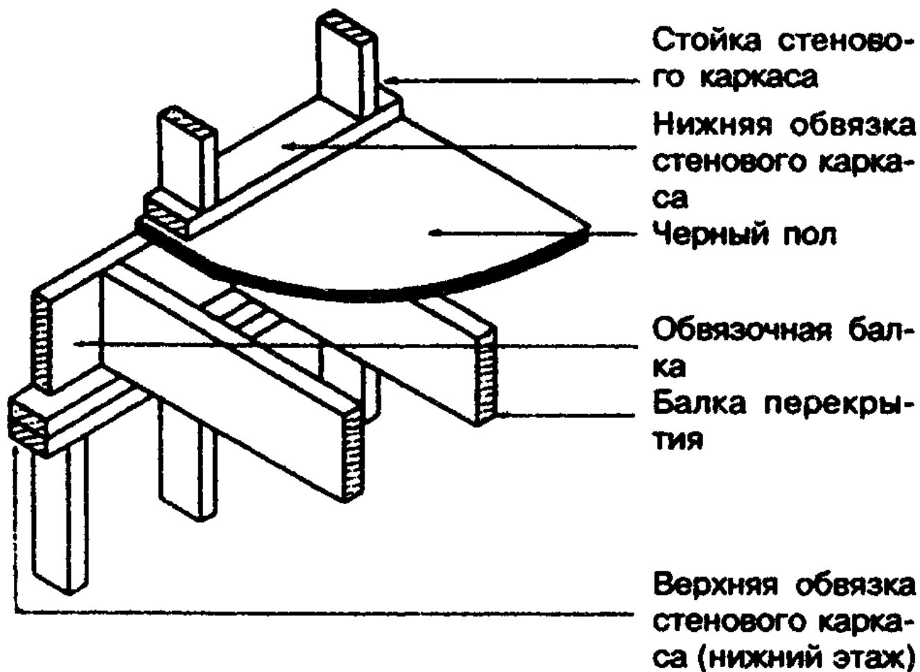
Рисунок 6-6 — Опираие балок перекрытия на каркас наружной стены
