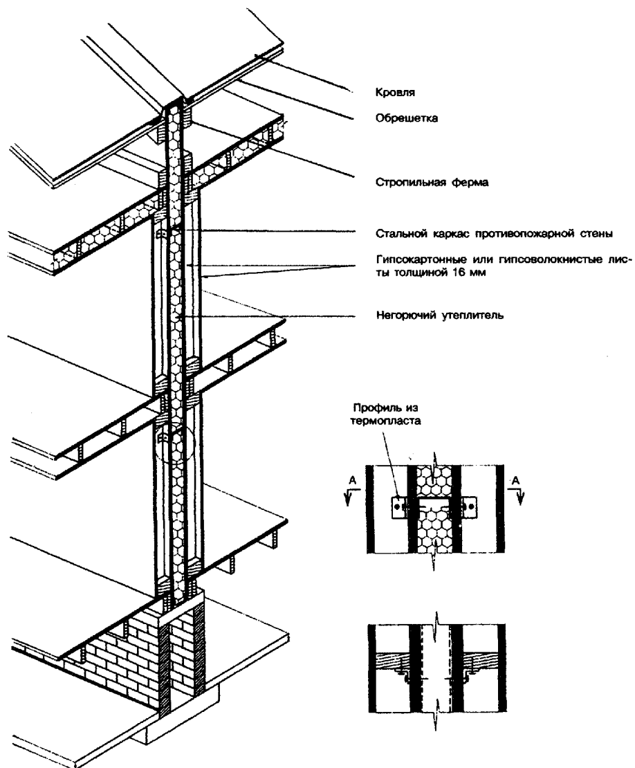
Рисунок 7-6 — Межквартирная противопожарная стена 2-го типа каркасной конструкции
