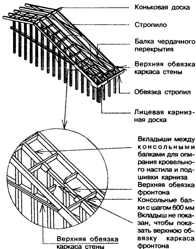
Рисунок 8-7 — Карниз над фронтоном с выносом более 300 мм
