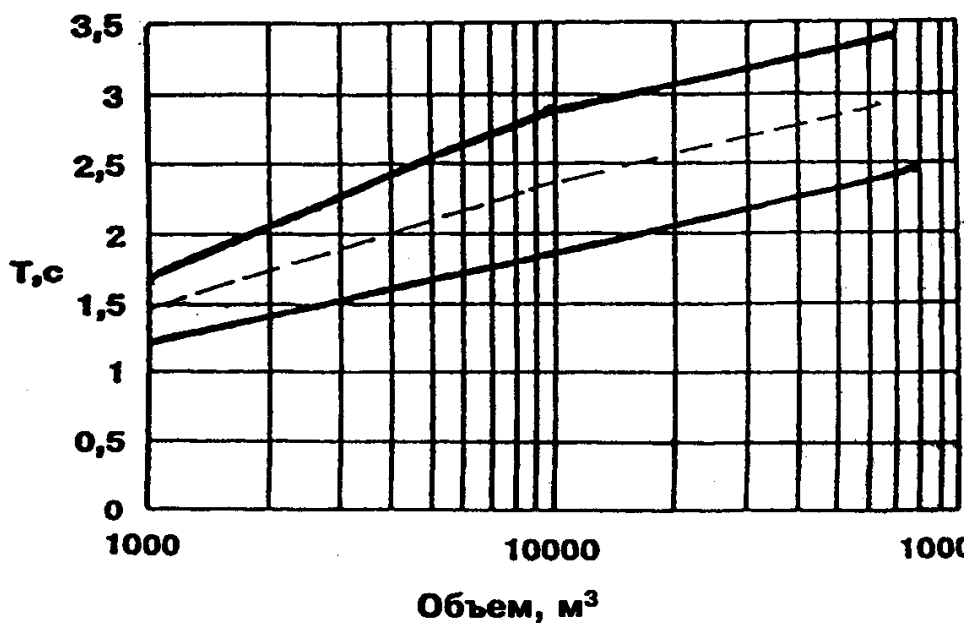
Рисунок М.1 — Рекомендуемое время реверберации на средних частотах для помещений в зависимости от их объема
