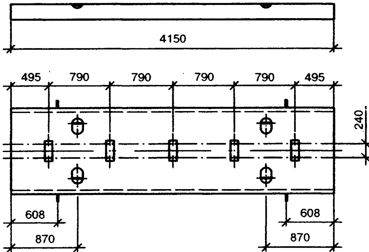
"Б4. Железобетонная плита"
