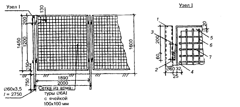
1 — стойка; 2 — патрубок; 3 — полускоба; 4 — рамка вертикальная; 5 — рамка горизонтальная; 6 — стержень вертикальный; 7 — стержень горизонтальный
