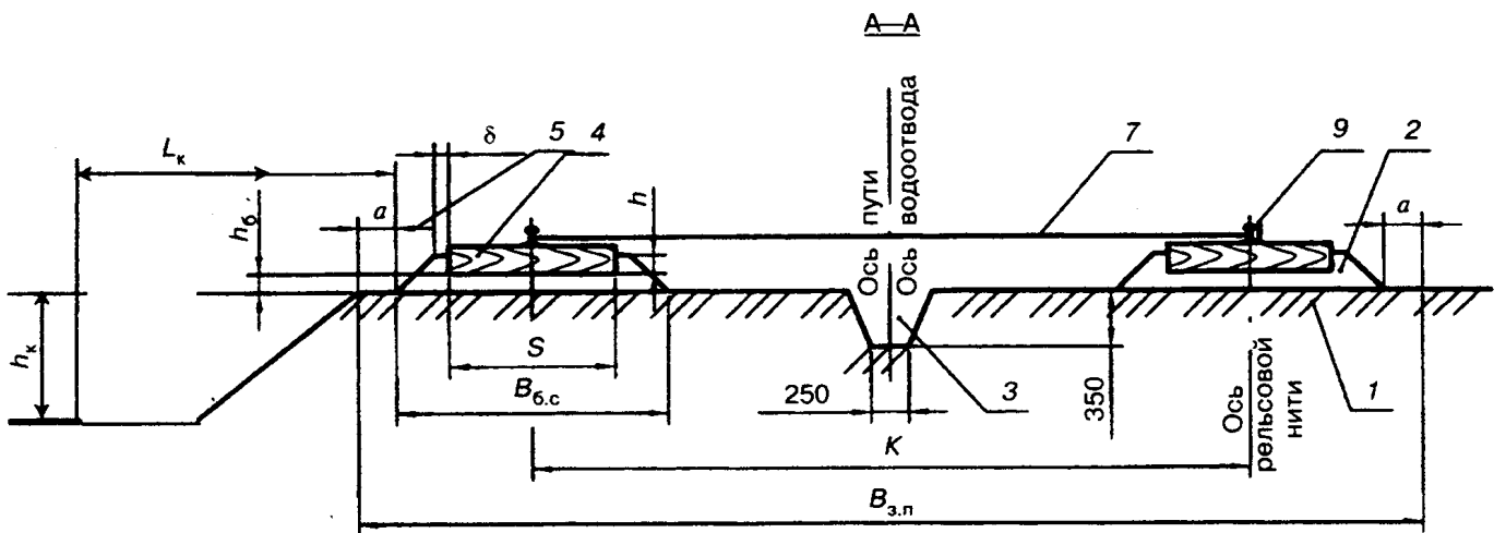
"Г.1 Конструкция кранового пути на деревянных полушпалах"
