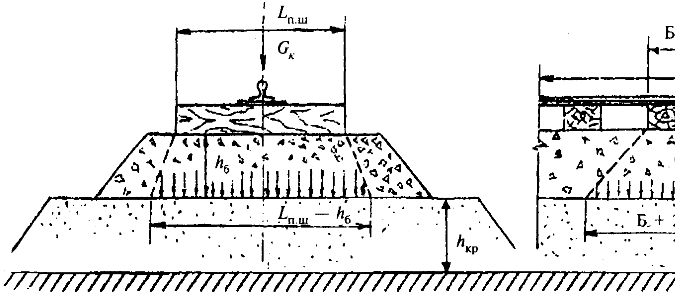
Рисунок И.2 — Схема нагрузок и воздействий на земляное
