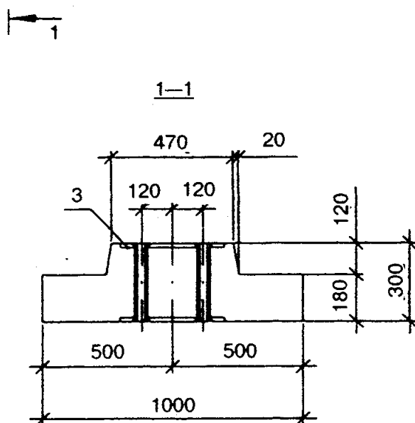
"Б5. Железобетонная балка типа БРК-6.24-04"
