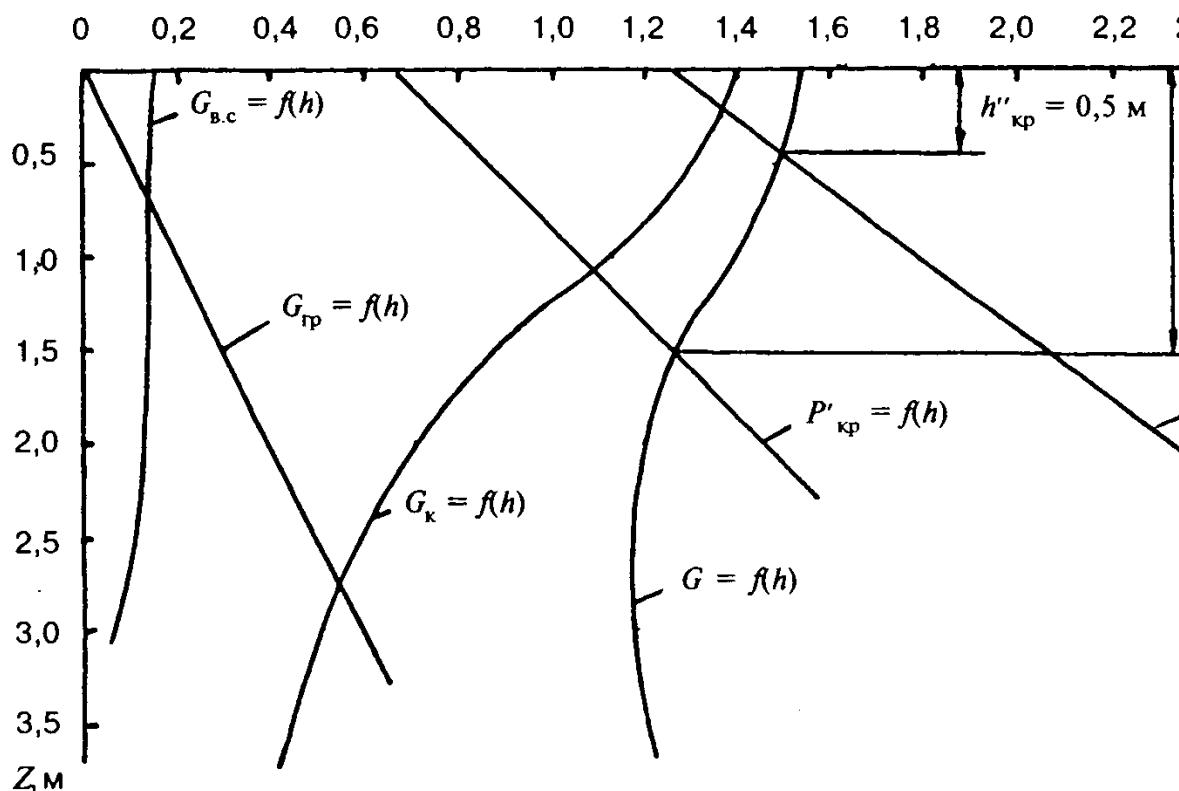
Рисунок И.3 — Распределение по глубине эпюр напряжений и критических нагрузок. G_{в.с} — эпюра напряжений от верхнего строения кранового пути; G_{к} — эпюра напряжений от крана; G_{гр} — эпюра напряжений от собственного веса грунта; G — суммарная эпюра напряжений; P'_{кр} и P''_{кр} — критические нагрузки 1-го и 2-го вариантов расчета; h'_{кр} и h''_{кр} — толщина защитного слоя для 1-го и 2-го вариантов расчета.
