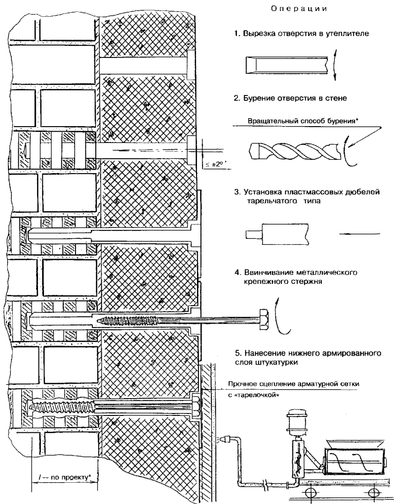
Рисунок А7 — Крепление плиты утеплителя с помощью пластмассовых дюбелей тарельчатого типа с металлическим стержнем (вариант: стеновой материал из пустотелых блоков)
