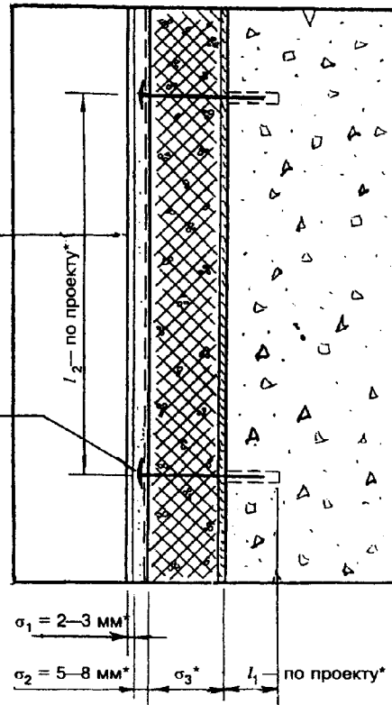
Рисунок А8 — Фрагмент наружной теплоизоляции здания с тонкой штукатуркой по утеплителю
