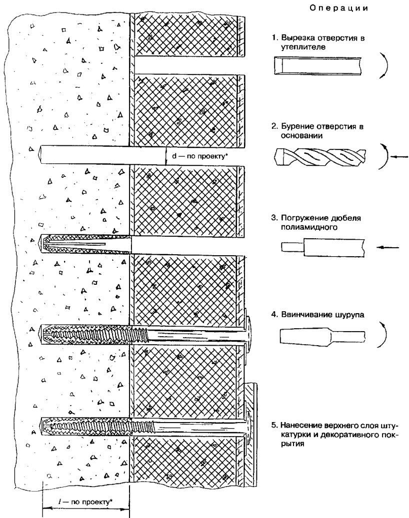
Рисунок А6 — Крепление плиты утеплителя с помощью дюбеля полиамидного и шурупов
