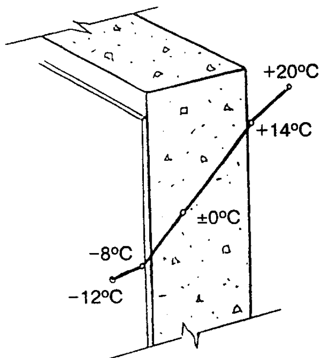
Рисунок 1 – Температурная кривая зимой
