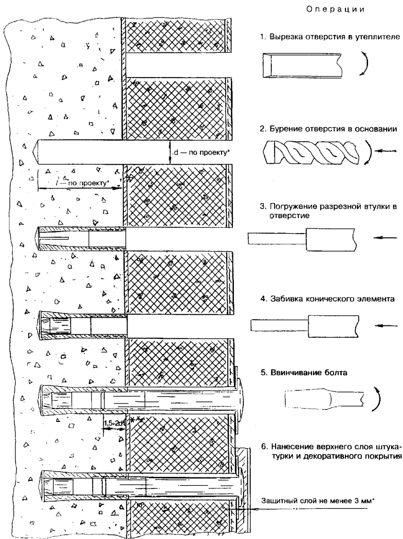
Рисунок А5 — Крепление плиты утеплителя с помощью дюбелей-втулок и винтов
