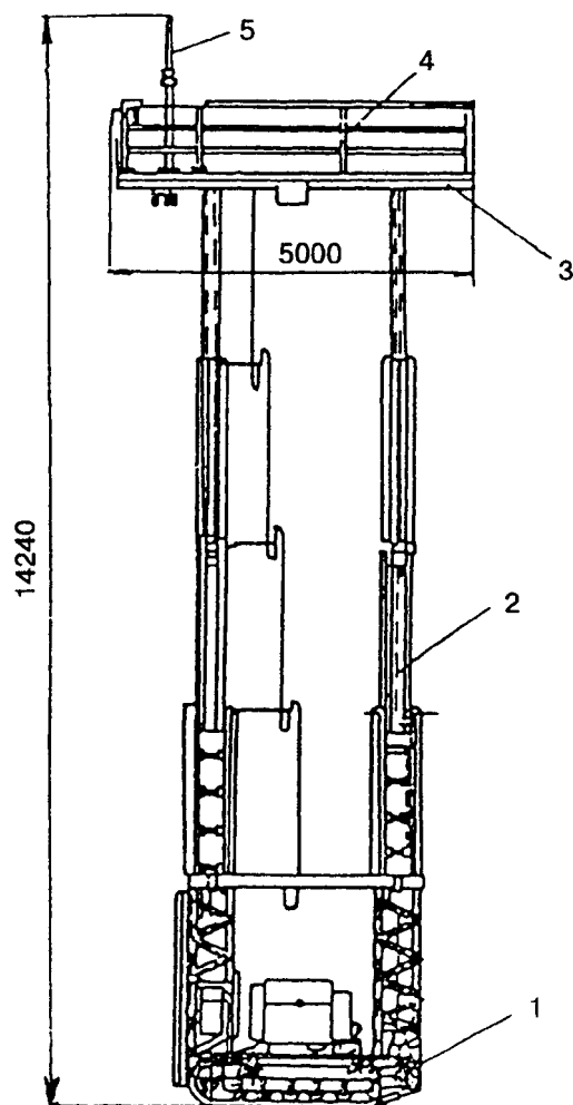
Подмости ПВС-12
