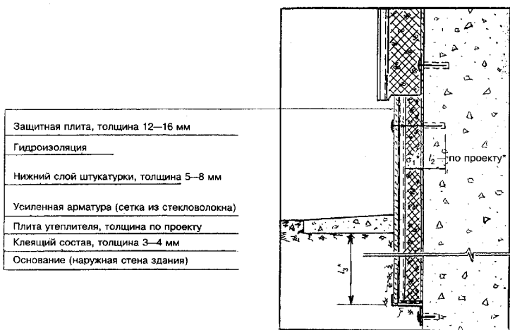
Рисунок А10 – Фрагмент утепления нижней (и ее заглубленной) части стены здания
