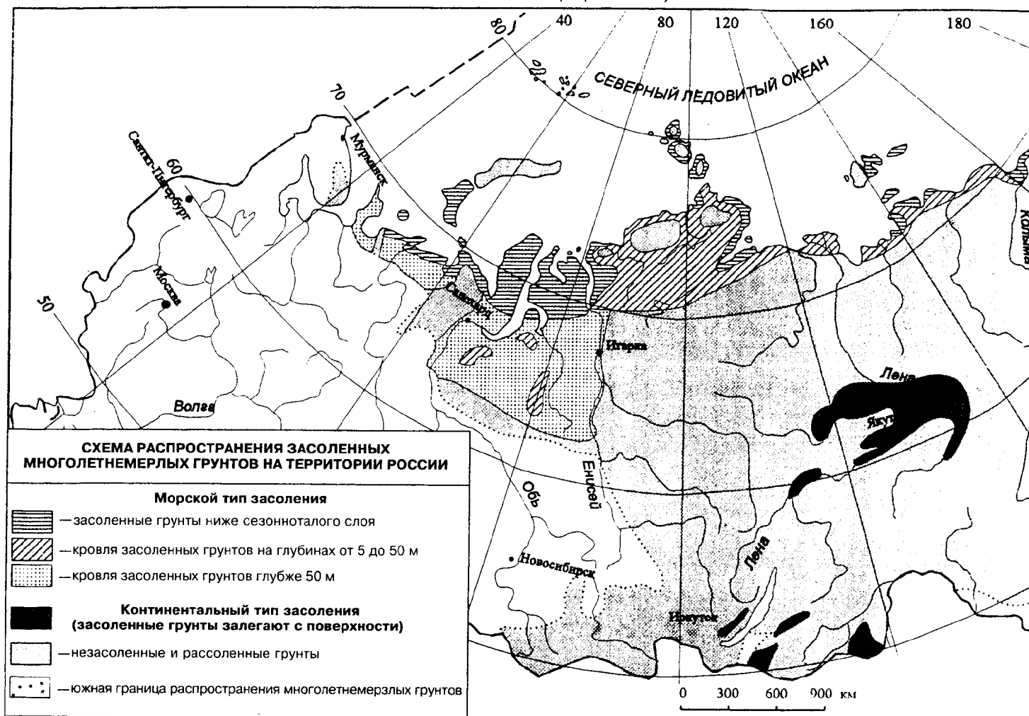
"Схема распространения засоленных многолетнемерзлых грунтов на территории России"
