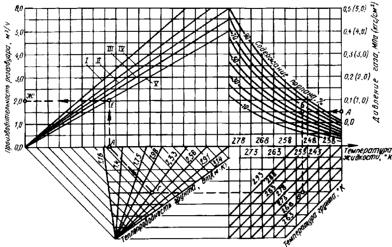
Номограмме для определения производительности резервуара сжиженного газа вместимостью 2,5 и 5 м³ (подземного) I – резервуар 5 м³, заполнение 85%; II – резервуар 5 м³, заполнение 50%; III – резервуар 5 м³, заполнение 35% и резервуар 2,5 м³, заполнение 50%; IV – резервуар 2,5 м³, заполнение 85%; V – резервуар 2,5 м³, заполнение 35%
