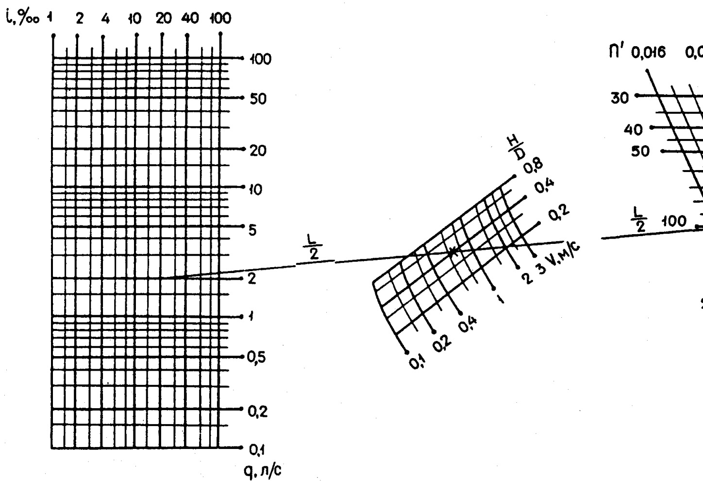
"Приложение 9. Номограмма для гидравлического расчета канализационных трубопроводов"
