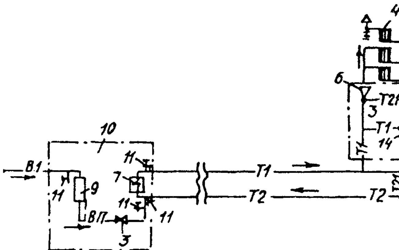
Рис. 2. Схема открытой системы теплосна
