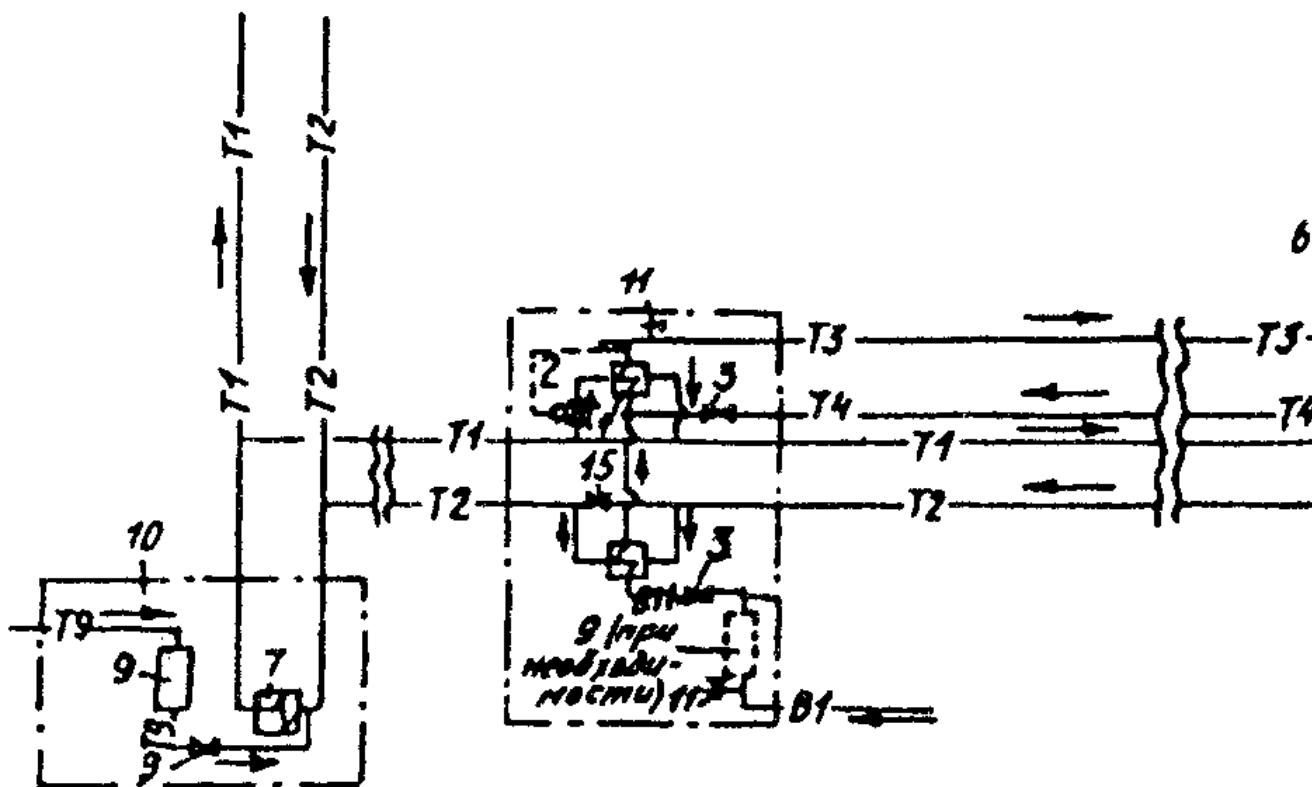
Рис. 1. Схема закрытой системы теплоснабжения
