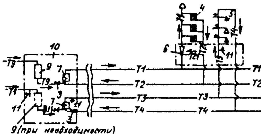
Рис. 3. Схема теплоснабжения с отдельными сетями горячего водоснабжения
