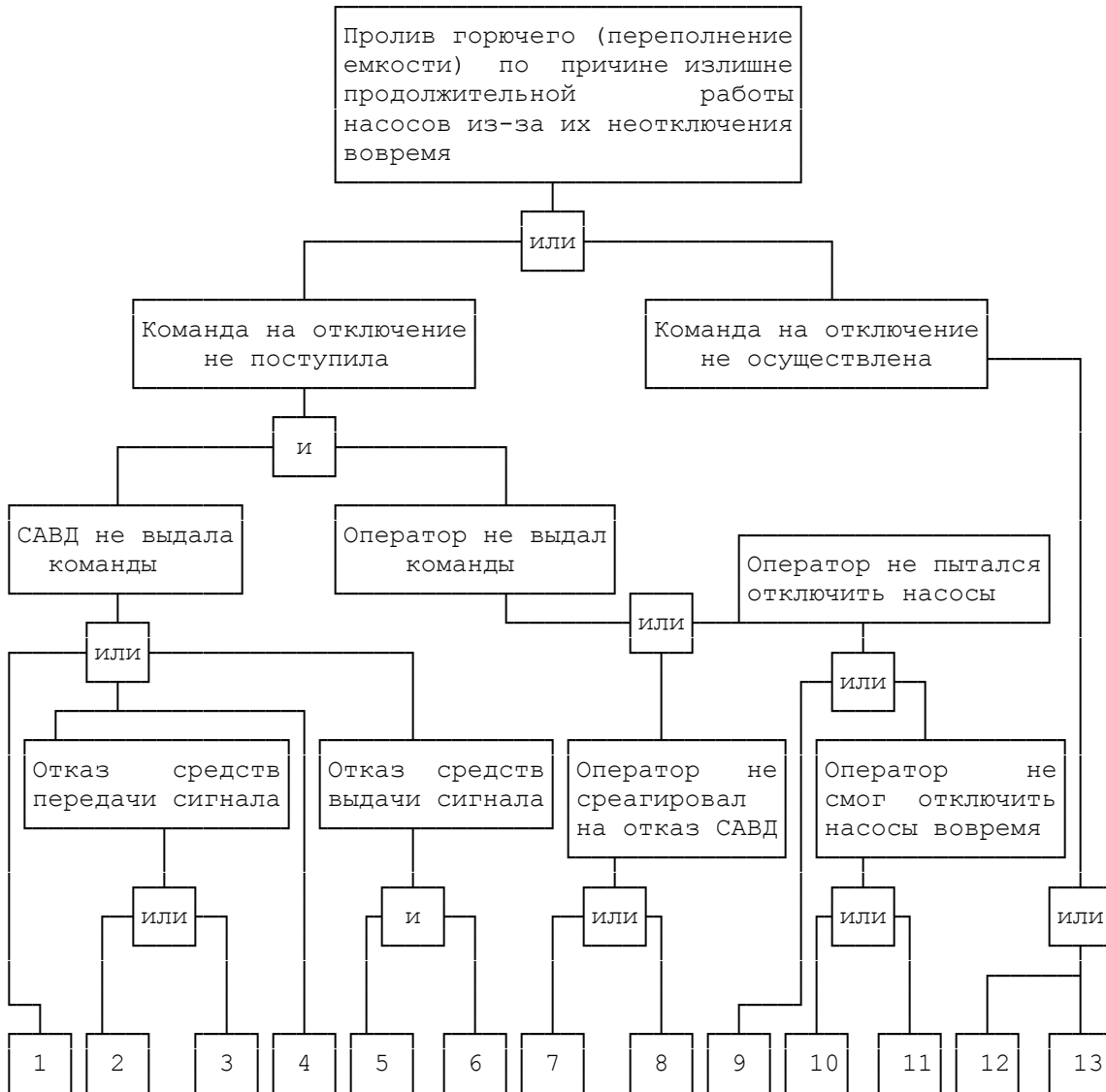
Рис. 2. "Дерево отказа" заправочной операции
