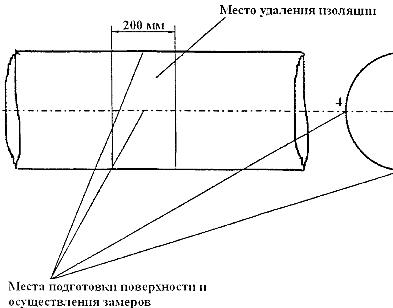
Рисунок К.4 – Схема расположения мест замера
