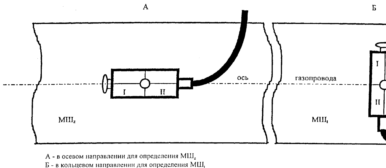
Рисунок К.6 – Расположение датчика при замерах НДС и ударной вязкости (КСУ) металла
