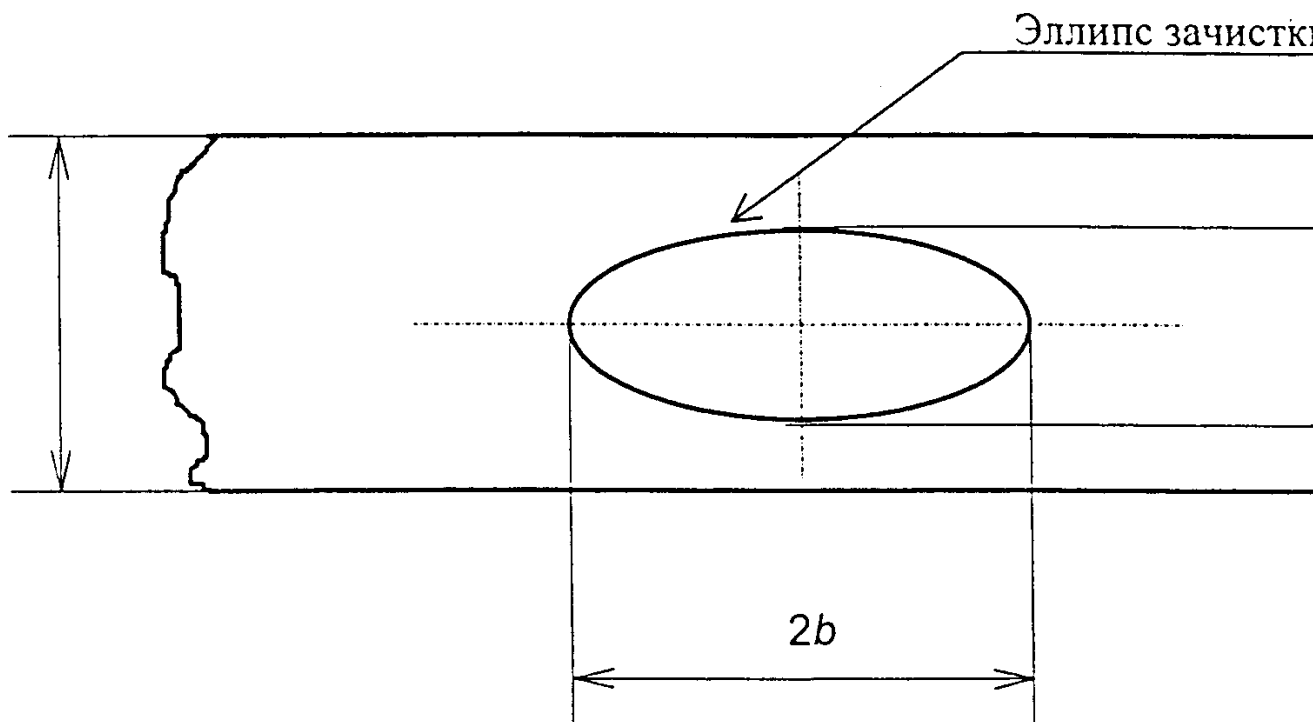
Рисунок И.2 – Схема зачистки на трубопроводе
