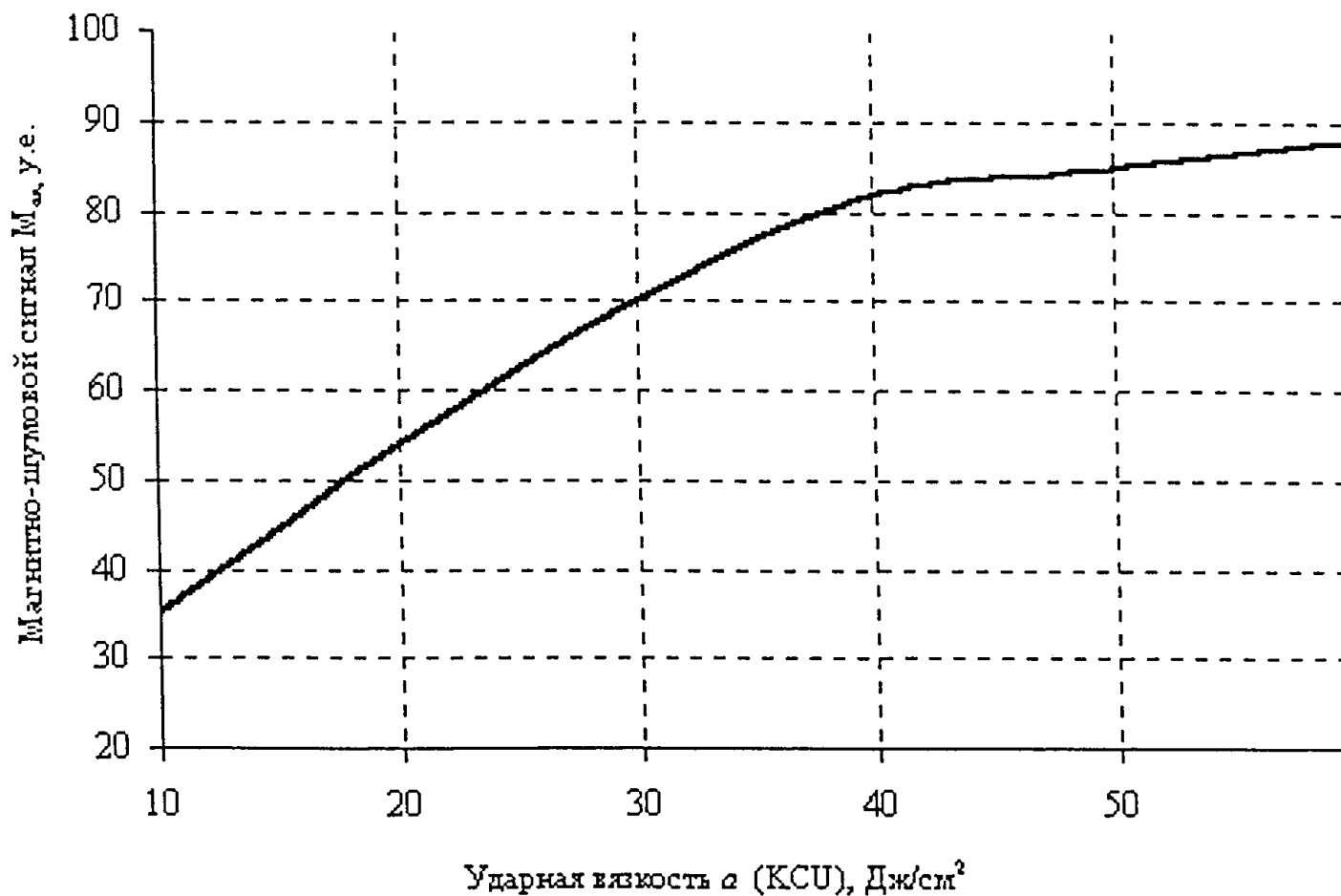
Рисунок К.3 – Зависимость ударной вязкости (КСУ) от магнитно-шумового сигнала. Прибор «ПИОН-01» зав. № 12. Ст 3, 4
