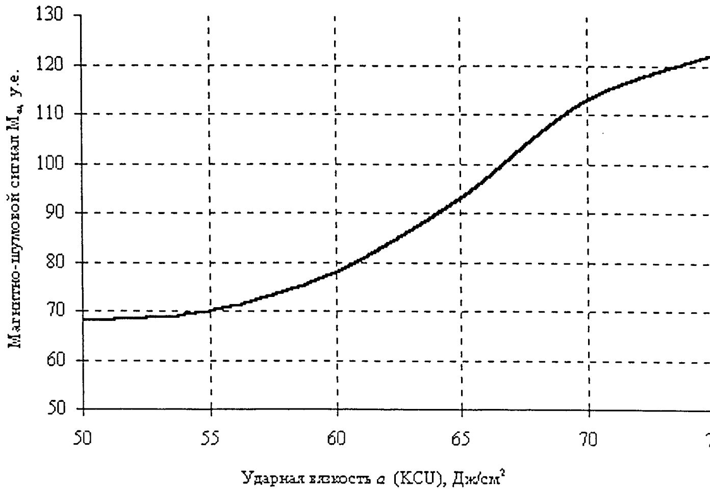
Рисунок К.2 – Зависимость ударной вязкости (КСУ) от магнитно-шумового сигнала. Прибор «ПИОН-01» зав. № 12. Сталь 10
