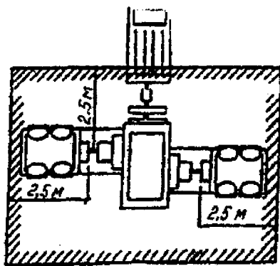
Газовый компрессор
