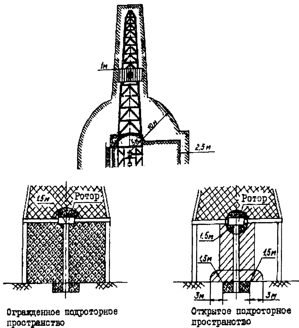
Рис. 2. Буровая установка с укрытием и привышечным сооружением для бурения скважин на море и месторождениях, содержащих сероводород
