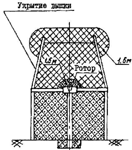
Буровая установка с огражденным подроторным пространством
