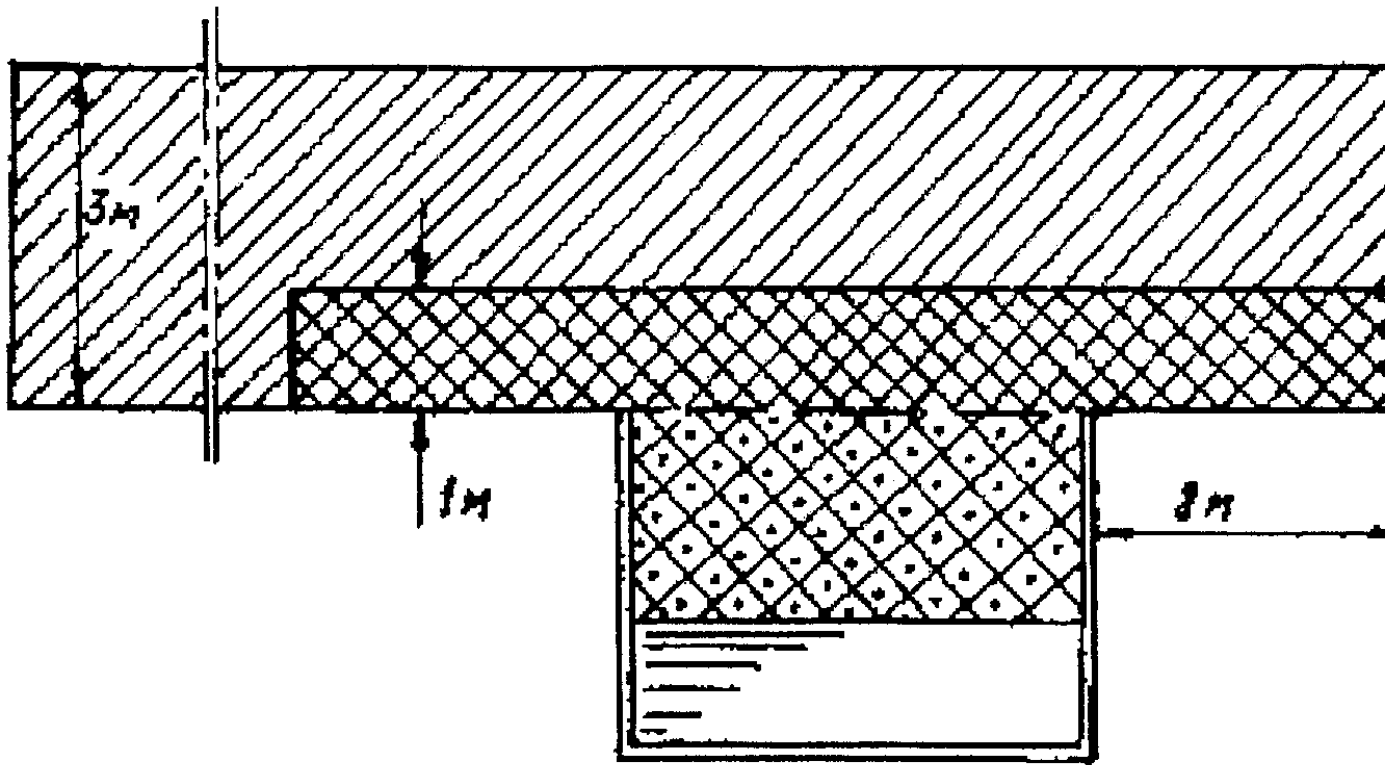
Рис. 7. Открытые пространства вокруг открытого сепаратора
