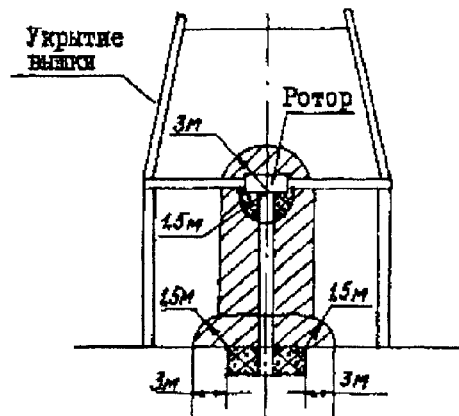
Буровая установка с открытым подроторным пространством
