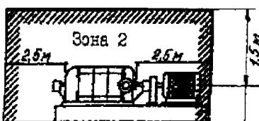
Насос для перекачки нефти
