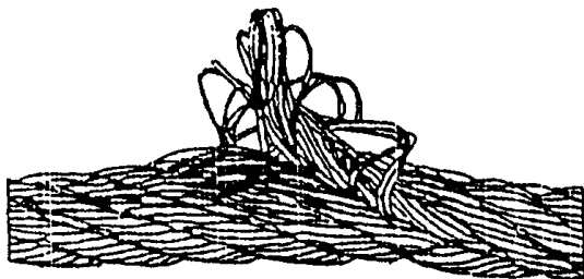
Рис.4 Выдавливание сердечника
