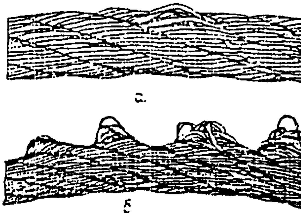
Рис.5. Выдавливание проволок прядей. а – в одной пряди, б – в нескольких
