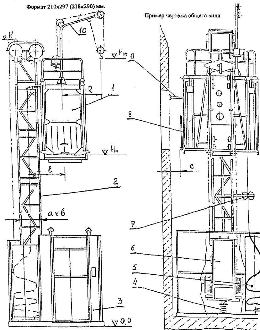
1. Кабина, 2. Мачта, 3. Опорный блок, 4. Буфер, 5. Контейнер электрокабеля, 6. Противовес, 7. Ловушка, 8. Трап, 9. Узел крепления, 10. Устройство монтажное
