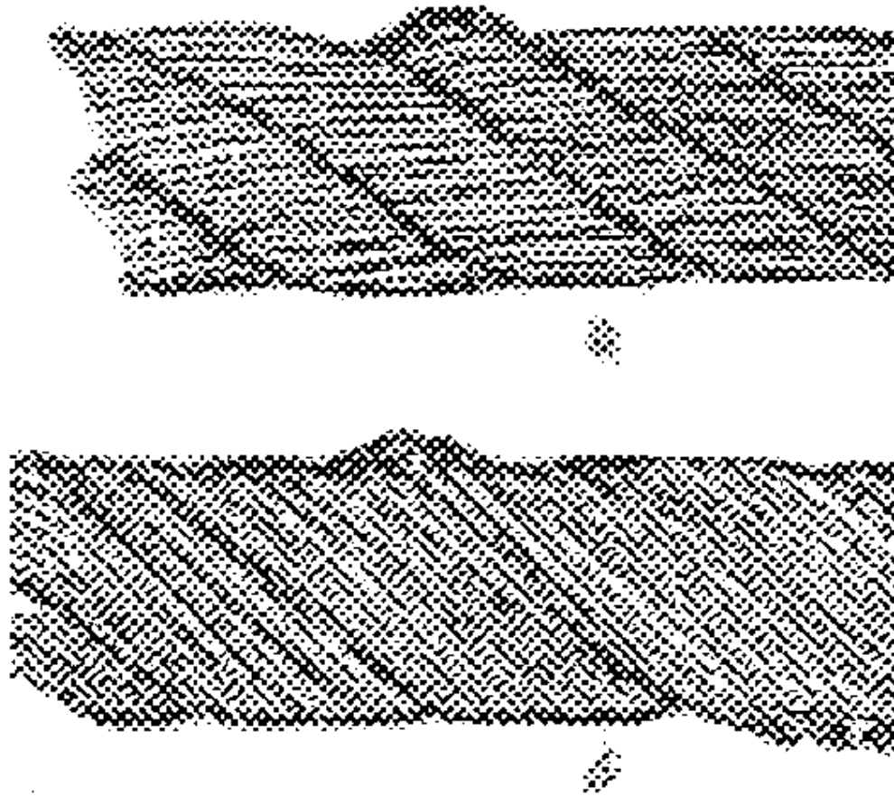
Рис. 2. Сочетание обрывов проволок с их износом а - в канате крестовой свивки, б — в канате односторонней свивки
