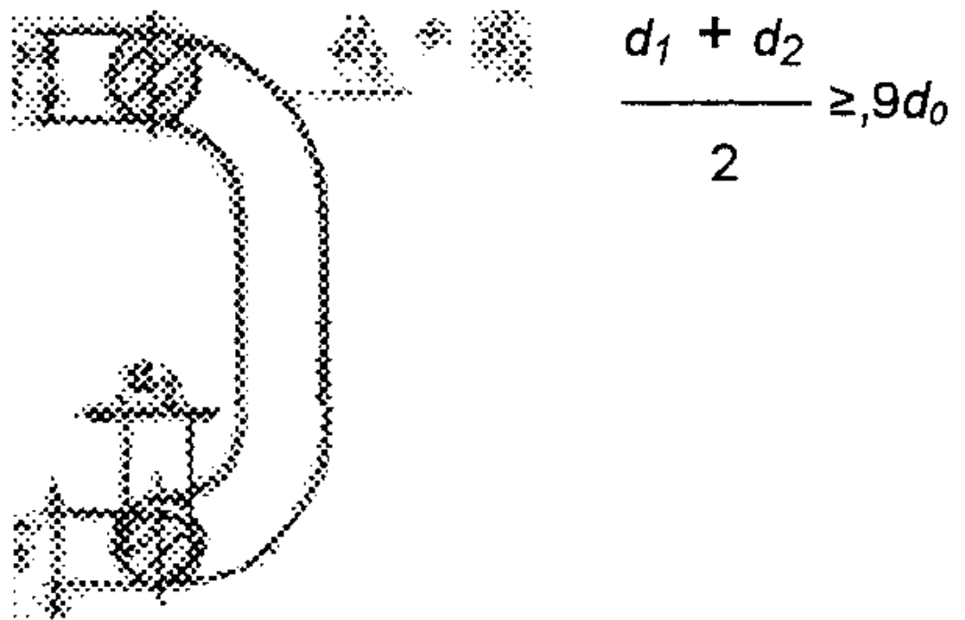
Рис 2. Уменьшение диаметра сечения звена
