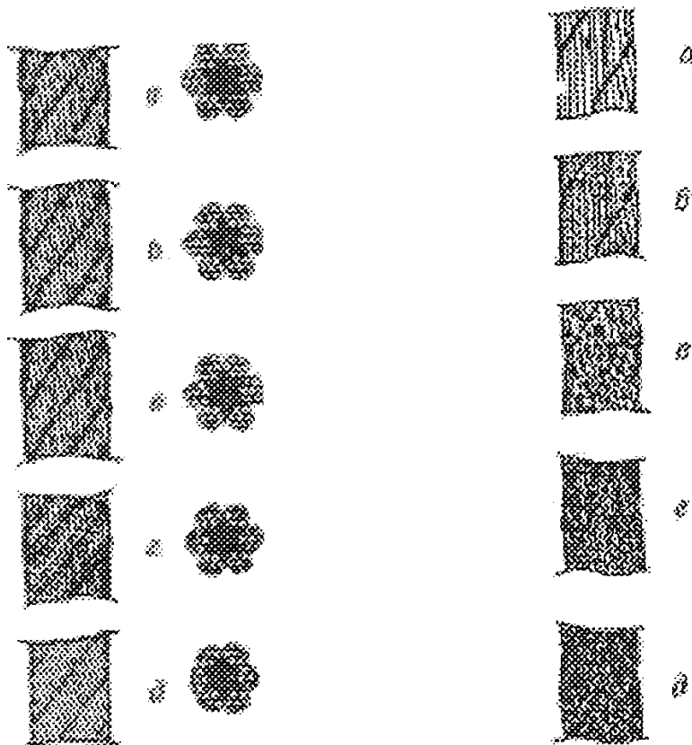
Рис. 5. Износ наружных проволок каната крестовой свивки:
