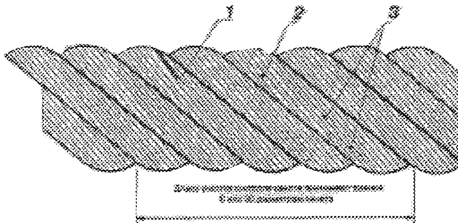
Рис. 4. Пример определения числа обрывов наружных проволок стального каната
