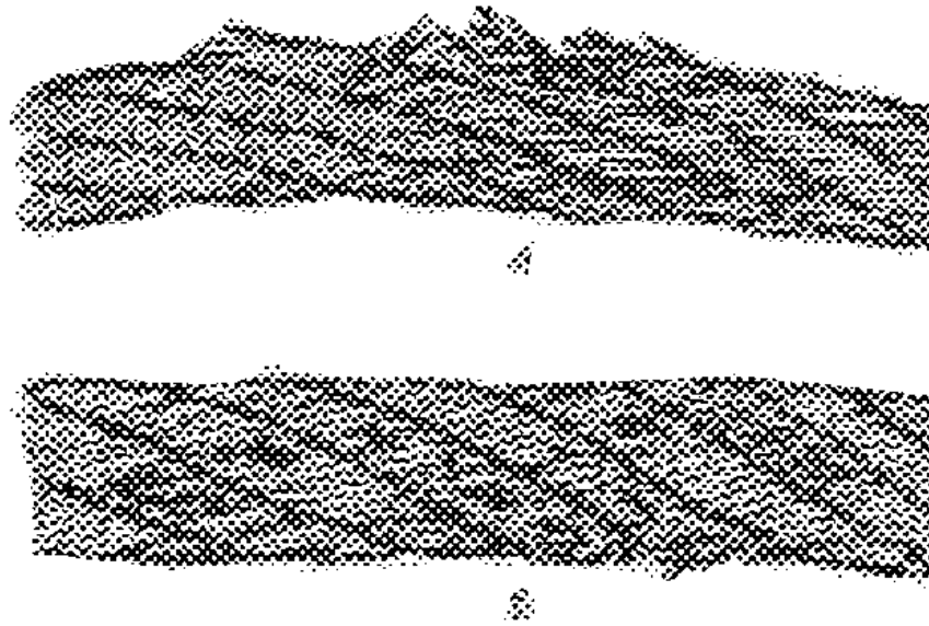
Рис. 3. Обрывы проволок в зоне уравнительного блика
