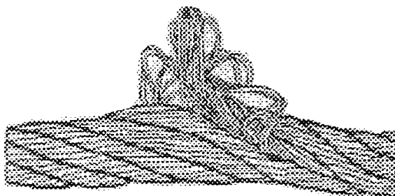
Рис. 11. Выдавливание сердечника
