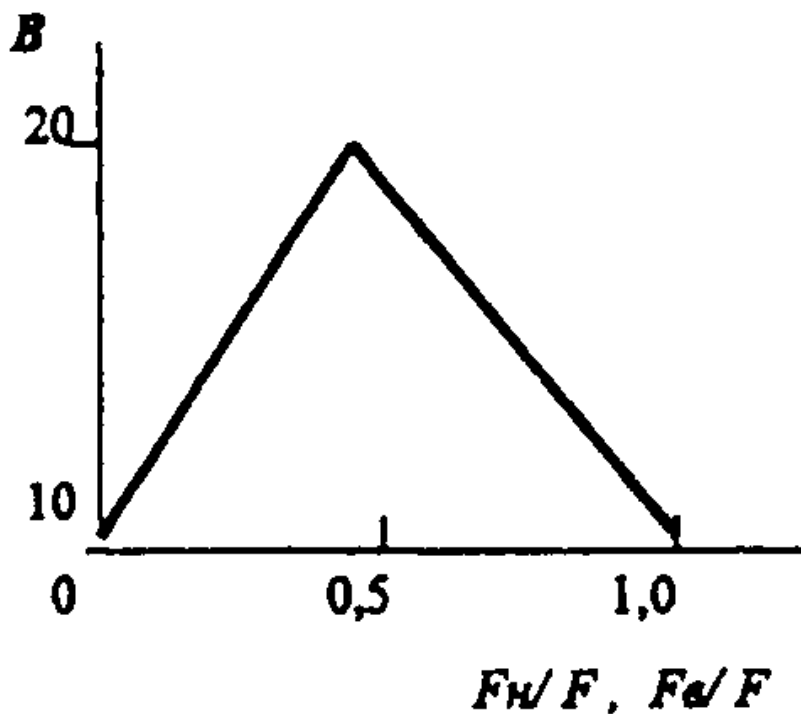
График для определения коэффициента B при расчете коэффициента k_4
