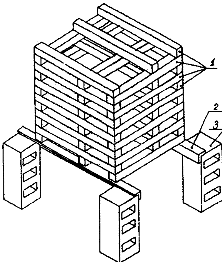
Устройство деревянного штабеля (модельного очага) для прове испытаний по тушению пожара класса А: 1 - деревянные бруски; 2 - стальной уголок; 3 - бетонный (металлический) блок
