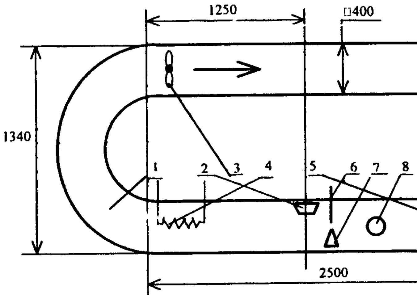
Испытательная камера
