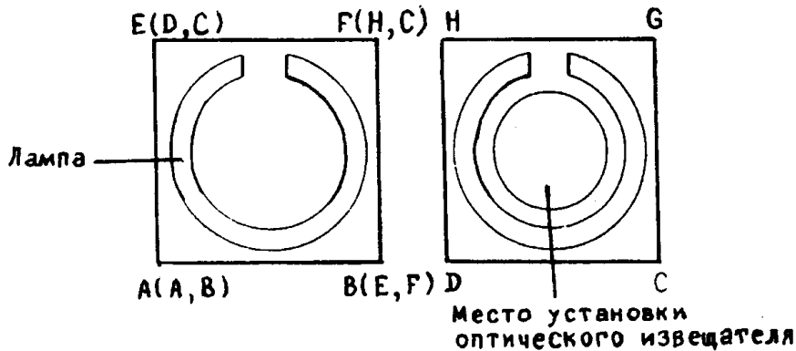
Устройство для проверки сохранения работоспособности оптических извещателей при воздействии фоновой освещенности
