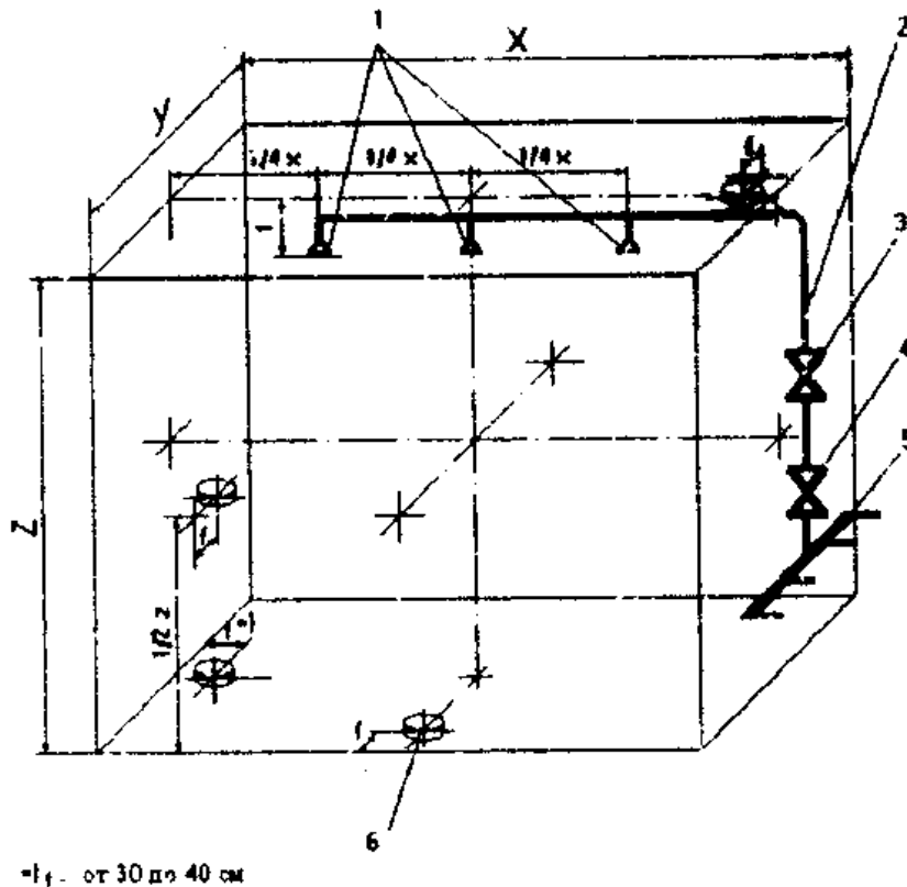
"Рис. 2. Схема расположения газовой арматуры и горелок в огневой камере"
