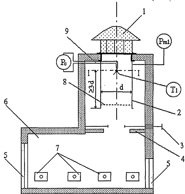
Рис. 2.1. Схема стенда для испытания крышных вентиляторов: 1 - испытываемый образец вентилятора; 2 - всасывающая камера; 3 - дроссельная диафрагма; 4 - перегородка; 5 - технологические проемы; 6 - печь; 7 - форсунки; 8 - выравнивающее устройство; 9 - комбинированный приемник давления (КПД); I-I - мерное сечение; TЭП - термоэлектрический преобразователь (ТЭП); T1 - температура на входе в вентилятор; P ст - статическое давление вентилятора; P в - перепад давления на комбинированном приемнике давления (КПД)
