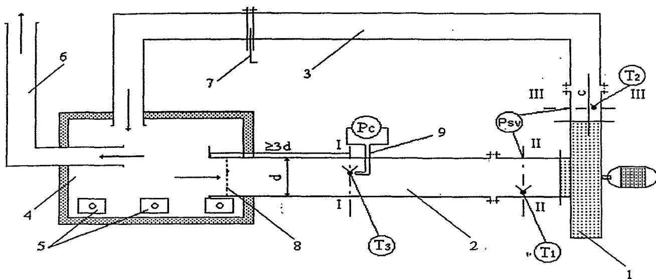
Рис. 1.1. Схема стенда для испытания вентиляторов:
