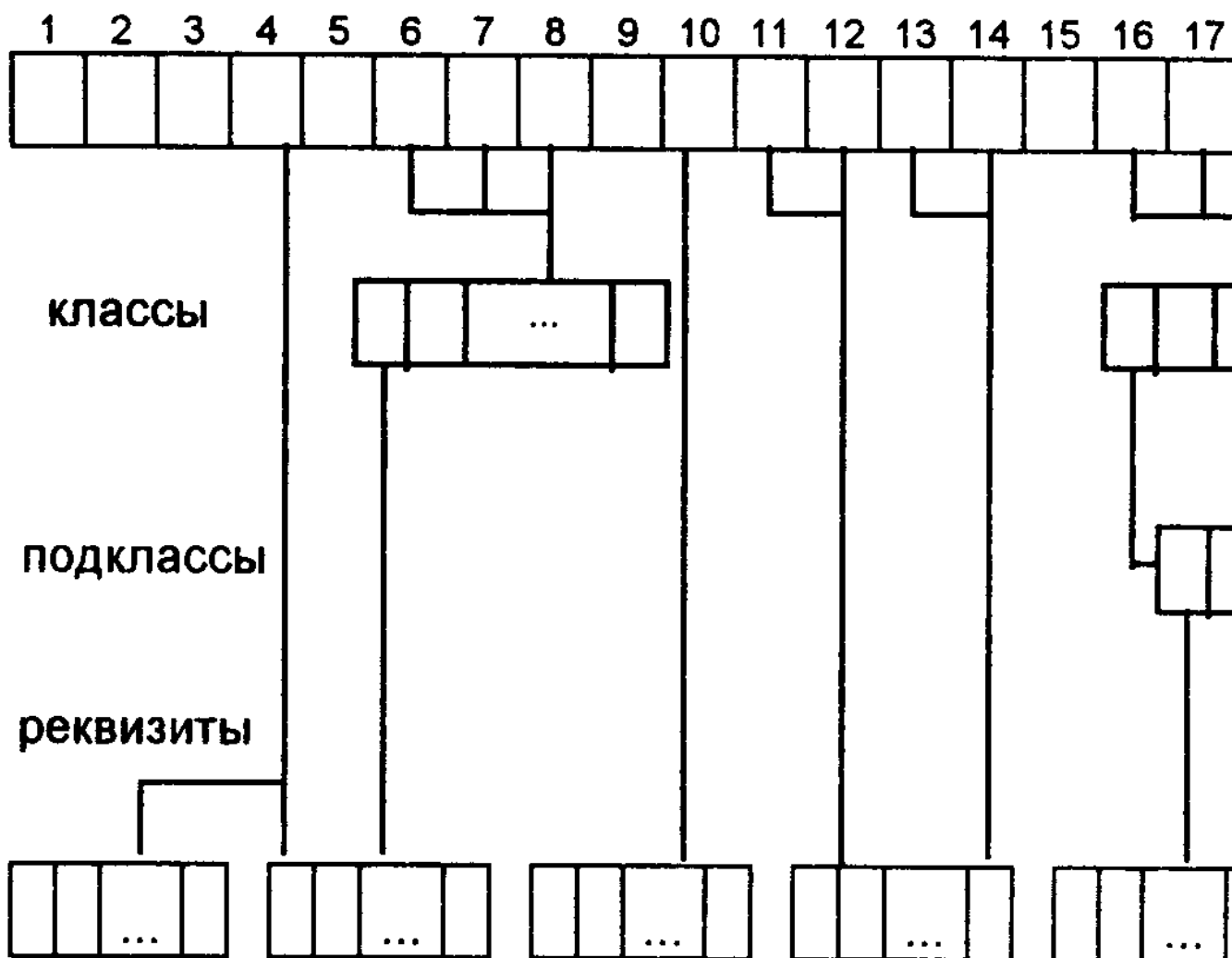
Рис. 2. Структура классификатора
