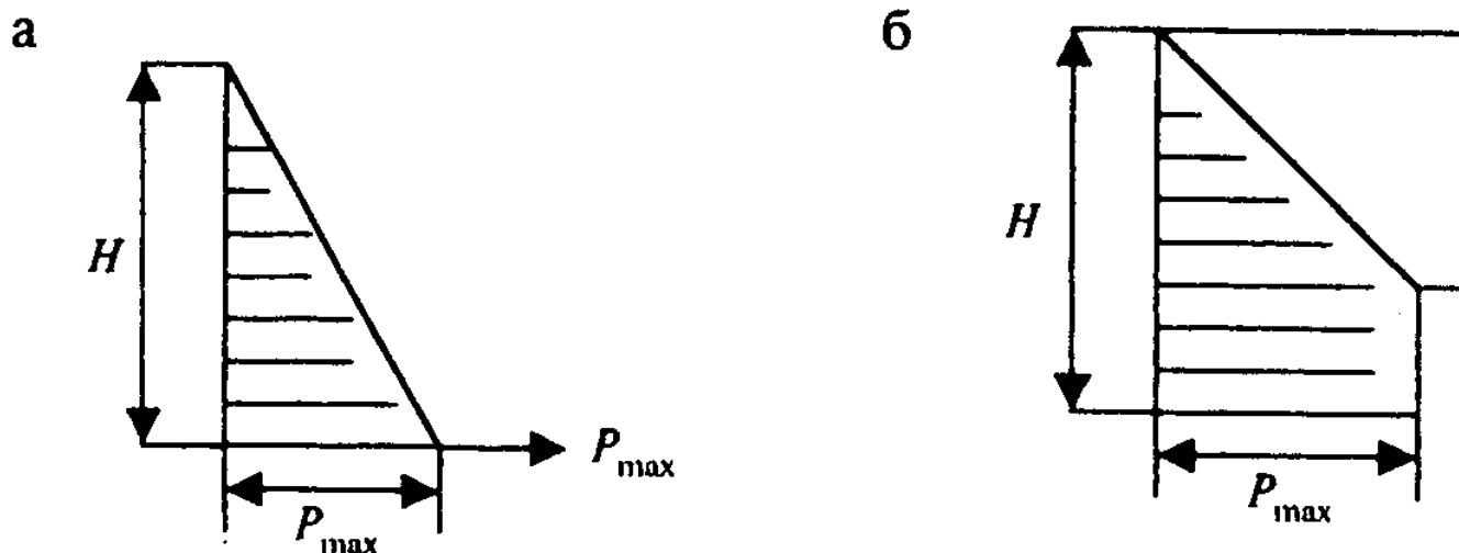
Рисунок Г.1 – Расчетные эпюры бокового давления бето а – гидростатическое давление; б – расчетное давление при уп внутренними вибраторами
