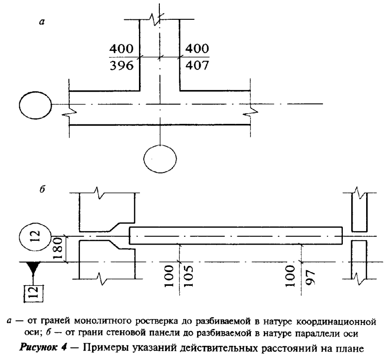
"Рис.4. Примеры указаний действительных расстояний на плане"
