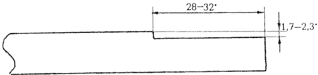
Рисунок 2 — Фальцевая кромка (ФК)
