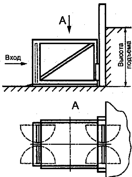
Рисунок 2 — Подъемная платформа без ограждения шахты
