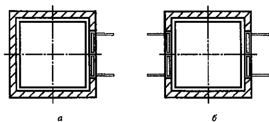
Рисунок 3 — Подъемные платформы
