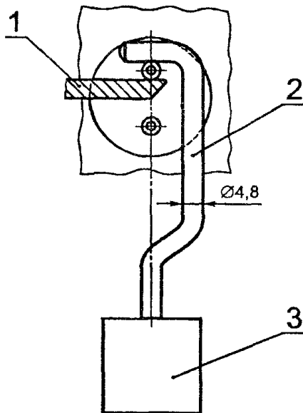
"Рисунок 13 - Устройство для проверки сопротивления стационарных розеток боковой деформации"
