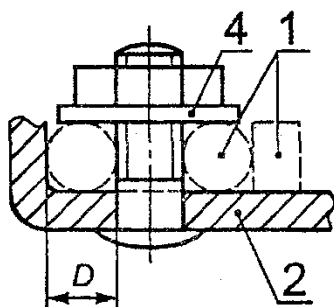
1 — возможный вариант; 2 — неподвижная деталь; 3 — прокладка или прижимная пластина; 4 — прижимная деталь; D — место расположения проводника
