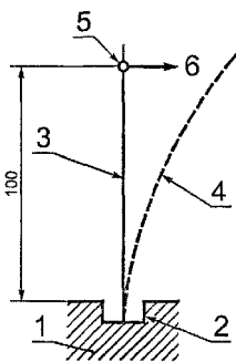
Рисунок 12 а — Принцип действия испытательной установки для проверки на изгиб безвинтовых контактных зажимов
