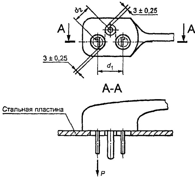
Рисунок 31 — Устройство для проверки механической прочности вилок
