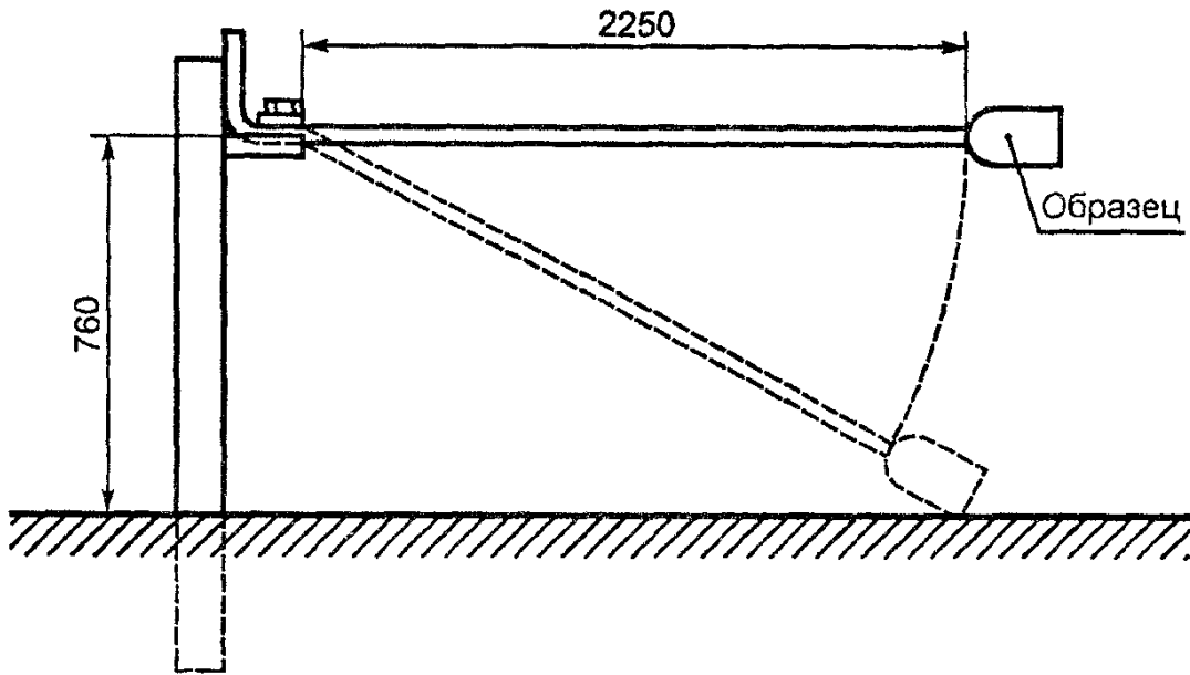
"Рисунок 29 - Установка для испытания на истирание изоляционных трубок штырей вилок"
