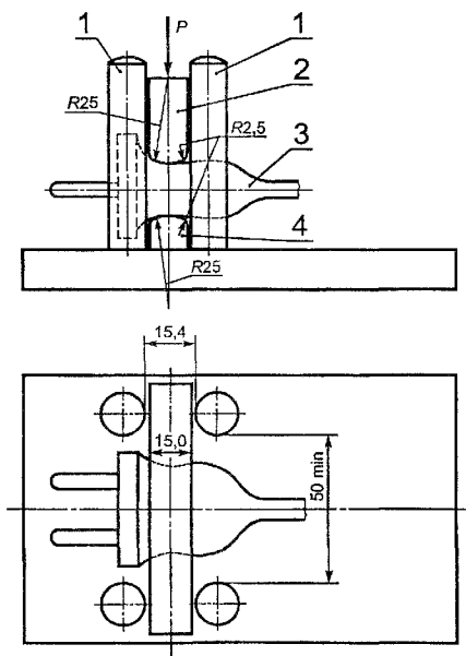
Рисунок 39 — Установка для испытания на сжатие вилок
