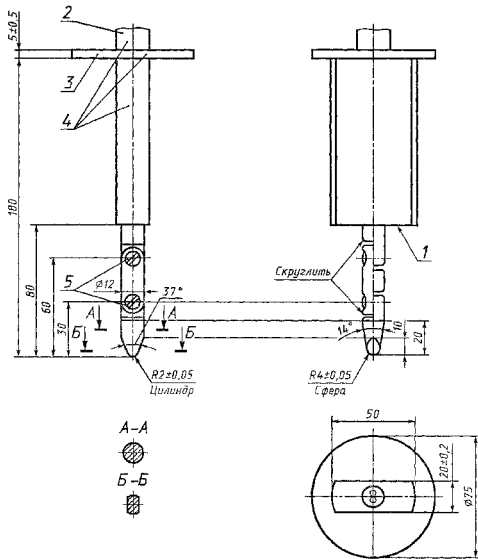
"Рисунок 7 - Самонарезающий режущий винт"
