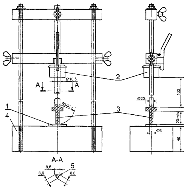
Рисунок 42 — Установка для испытания ударом при низкой температуре
