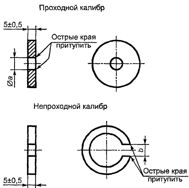
Рисунок Б.3 — Калибры для проверки диаметров штырей вилок
