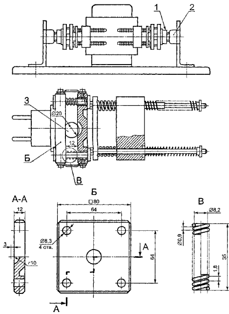
"Рисунок 15 - Блок испытательной стены для проведения испытаний в соответствии с требованиями 16.2.1"
