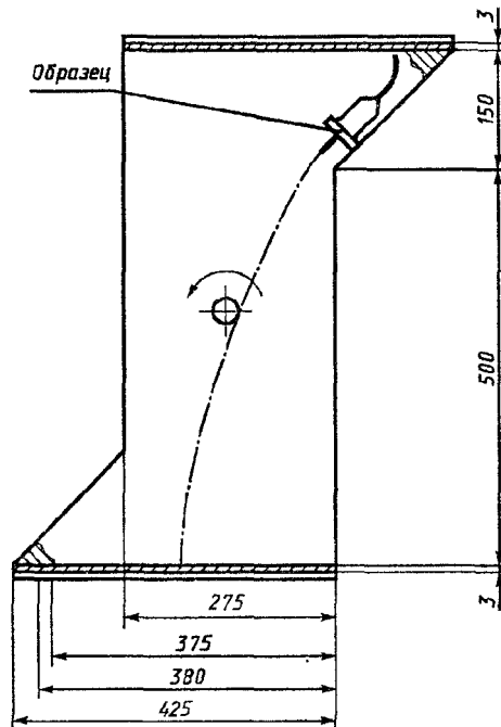
Рисунок 26 — Барабан для испытания соединителей на свободное падение
