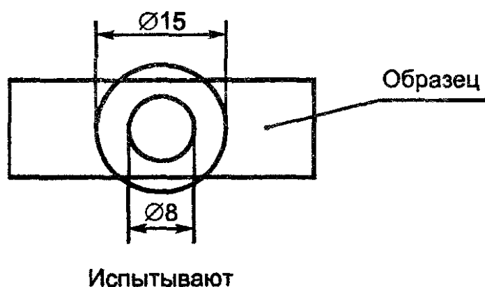
Рисунок 43 — Схематическое изображение требований 28.1.1
