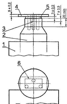
"Рисунок 39 - Установка для испытания на сжатие вилок"
