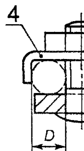
1 — возможный вариант; 2 — неподвижная деталь; 3 — прокладка или прижимная пластина; 4 — прижимная деталь; D — место расположения проводника
