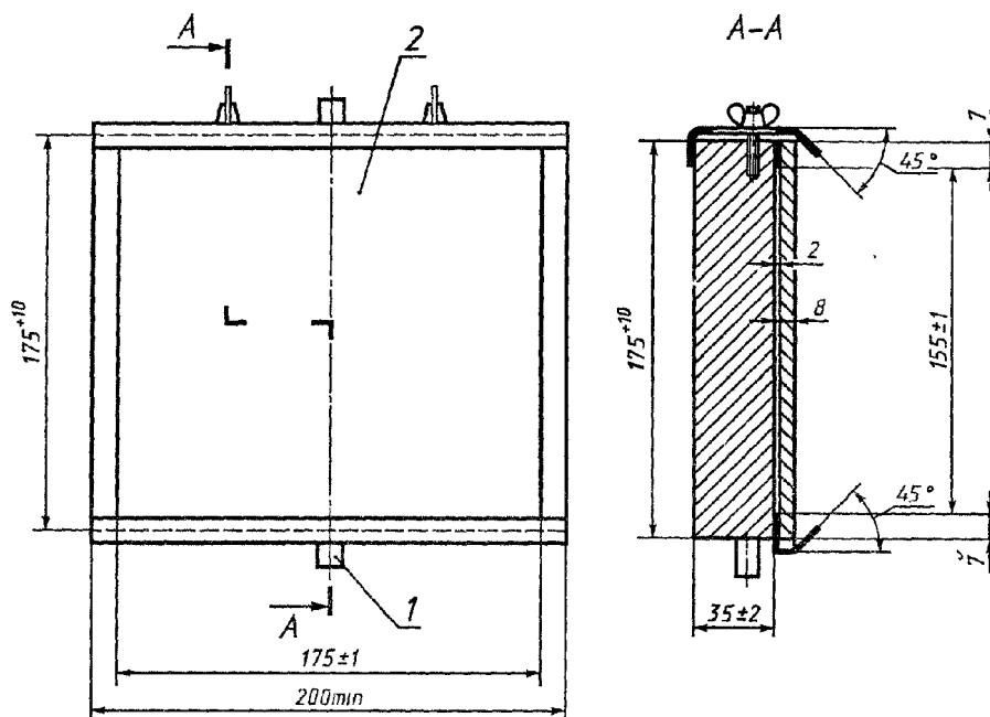
Рисунок 24 — Монтажная опора
