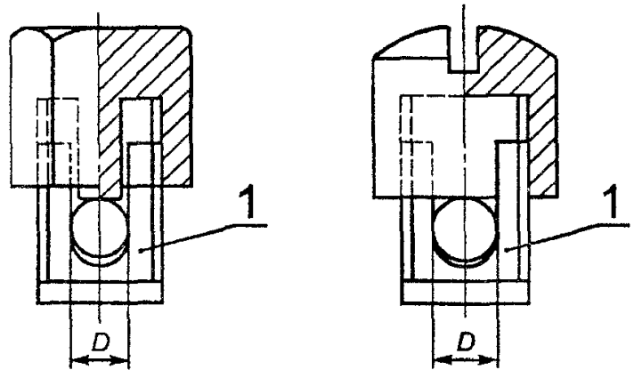
1 — неподвижная деталь; D — место расположения проводника 1
