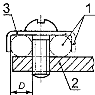
"Рисунок 3 - Зажимы с крепежной головкой, требующие применения прокладки, прижимной пластины или специальной прижимной детали"
