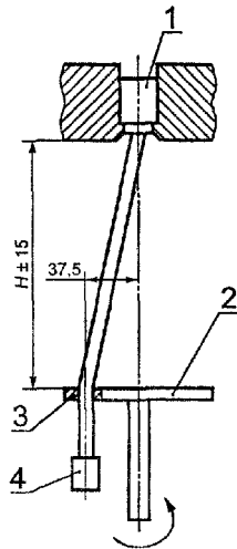
1 — зажим; 2 — плата; 3 — втулка; 4 — груз
