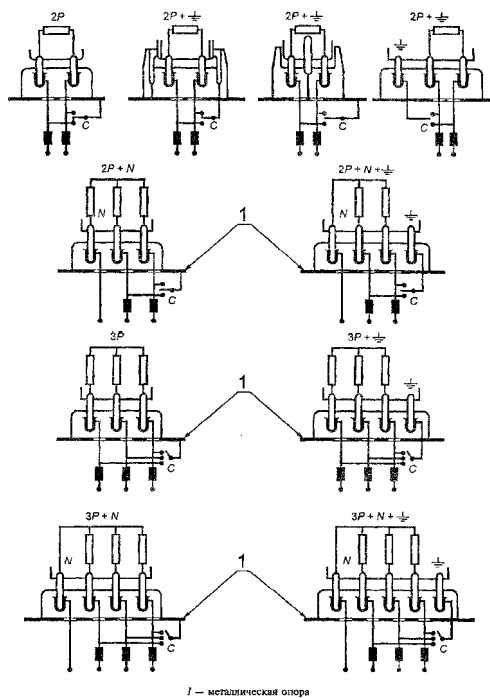
Рисунок 17 — Схемы соединения для испытания на нормальную работу
