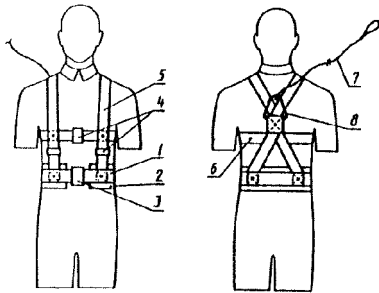
Рисунок 4 — Лямочный пояс, тип Г
