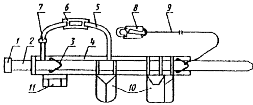
Рисунок 2 — Безлямочный пояс, тип Б
