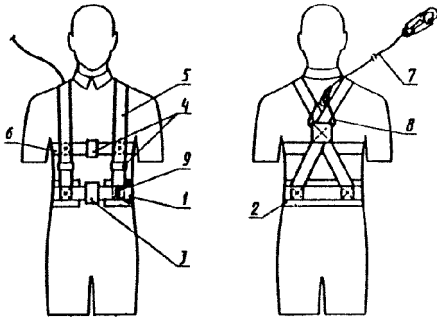
Рисунок 3 — Лямочный пояс, тип В
