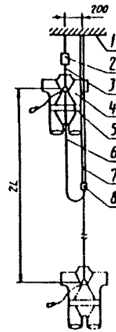
Рисунок 10 — Схема испытания лямочных поясов типов В, Д и Е динамической нагрузкой
