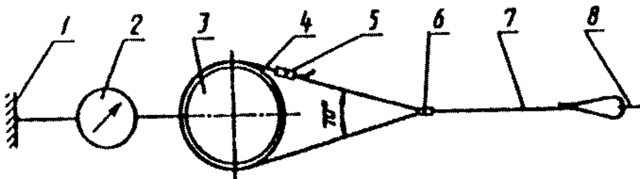
Рисунок 7 — Схема испытания пояса в целом статической нагрузкой
