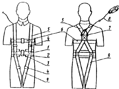
Рисунок 5 — Лямочный пояс, тип Д
