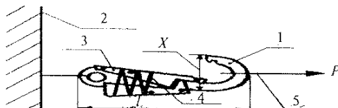
Рисунок 8,а — Схема испытания карабина статической нагрузкой
