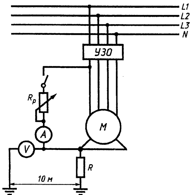
Рисунок В.3 — Схема проверки УЗО по методу 3
