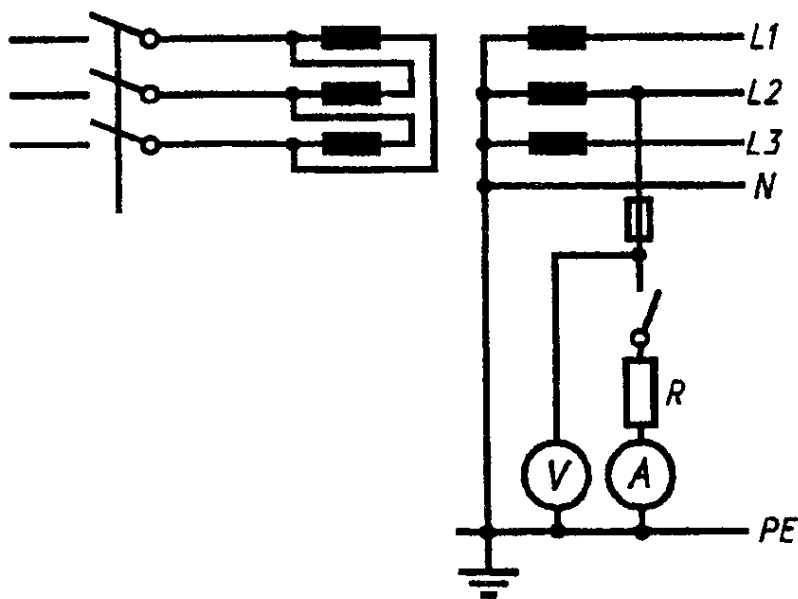
Рисунок D.1 – Схема измерения по методу 1
