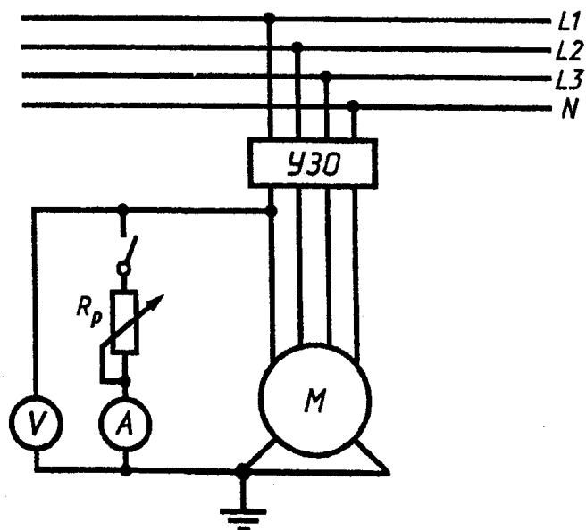
Рисунок В.1 — Схема проверки УЗО по методу 1
