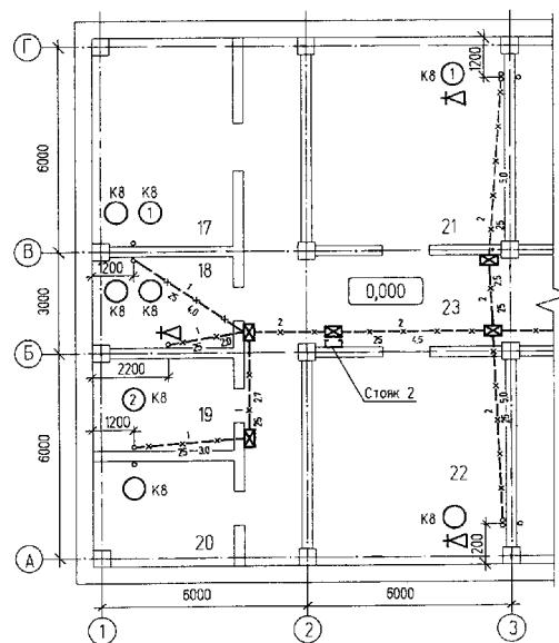
ПРИЛОЖЕНИЕ Ю (справочное) Пример выполнения плана каналов скрытой проводки и абонентских устройств
