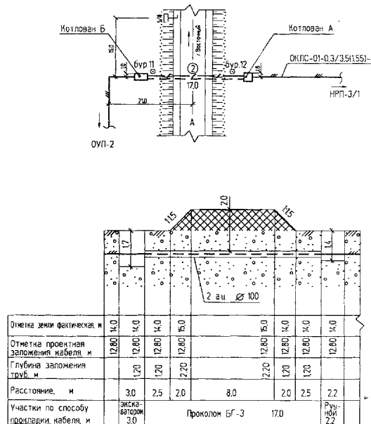
"Пример выполнения плана и продольного профиля кабельного перехода через автодорогу"
