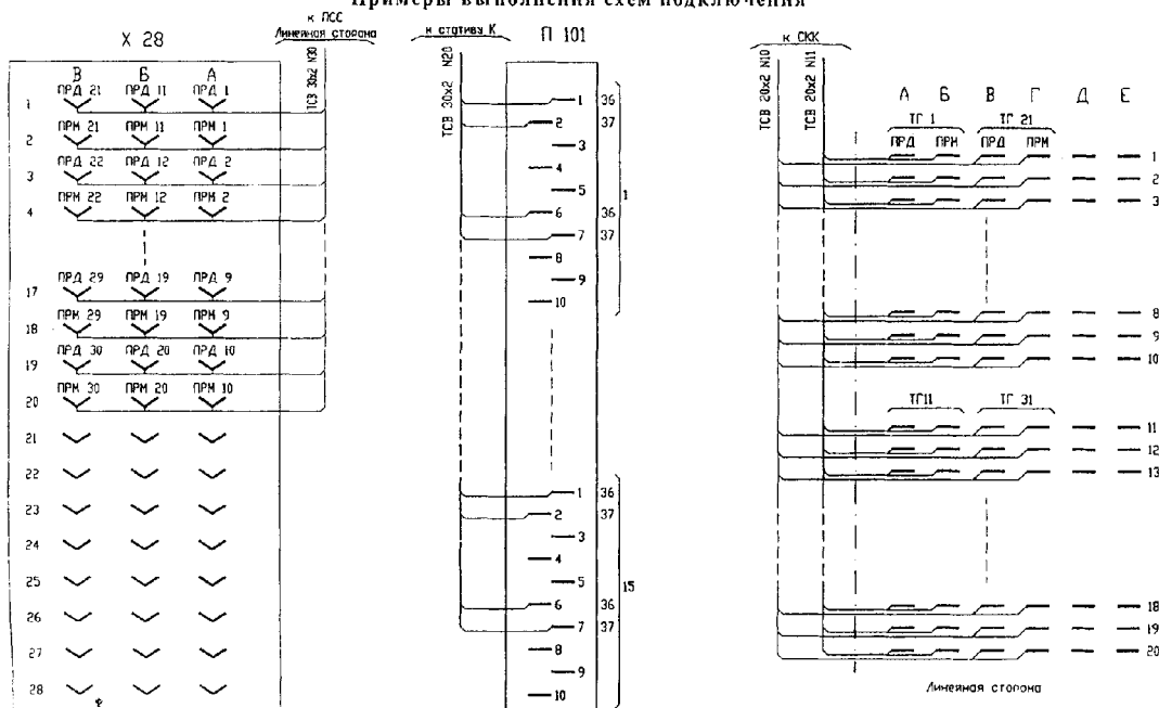
"Примеры выполнения схем подключения"
