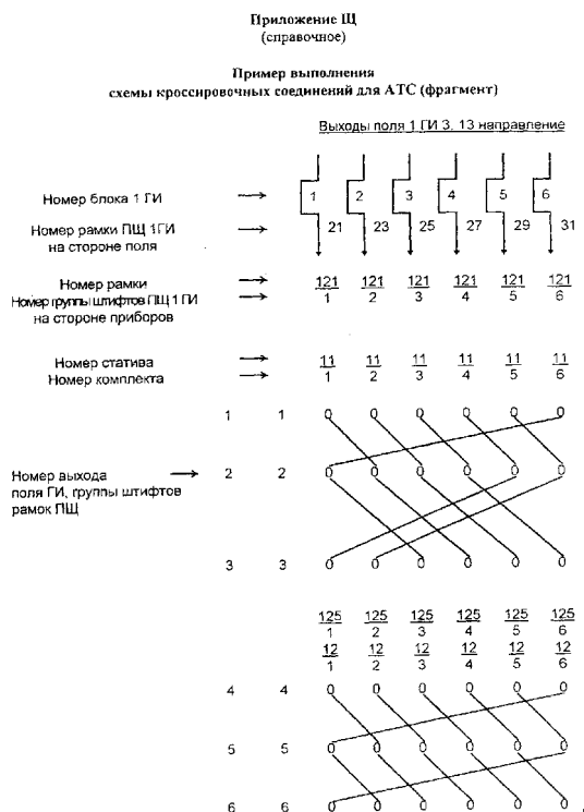
"Пример выполнения схемы кроссировочных соединений для АТС (фрагмент)"
