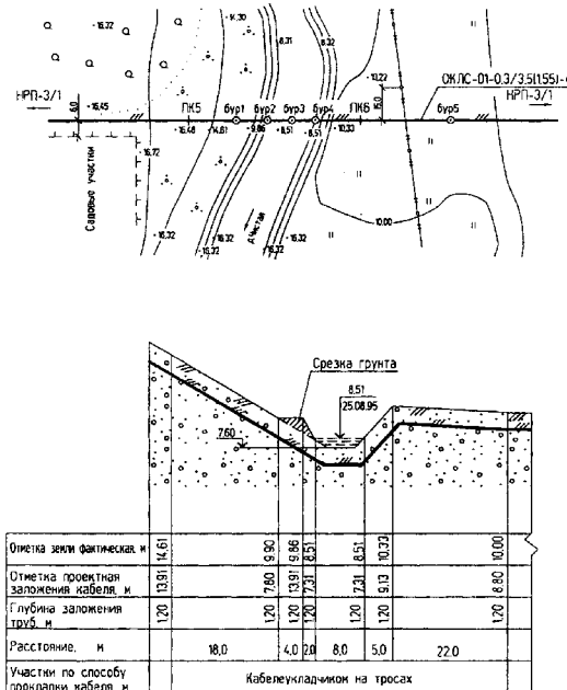
"Пример выполнения плана и продольного профиля кабельного перехода через несудоходную реку"
