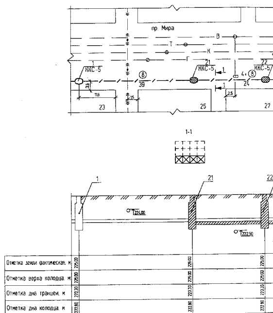
Примеры выполнения плана и продольного профиля кабельной канализации
