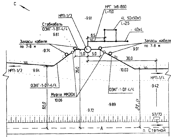
"Пример выполнения плана трасс кабелей и заземляющего устройства на площадке НРП"
