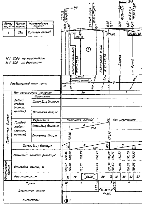
"Пример оформления продольного профиля железнодорожного пути на неспланированной застроенной территории"
