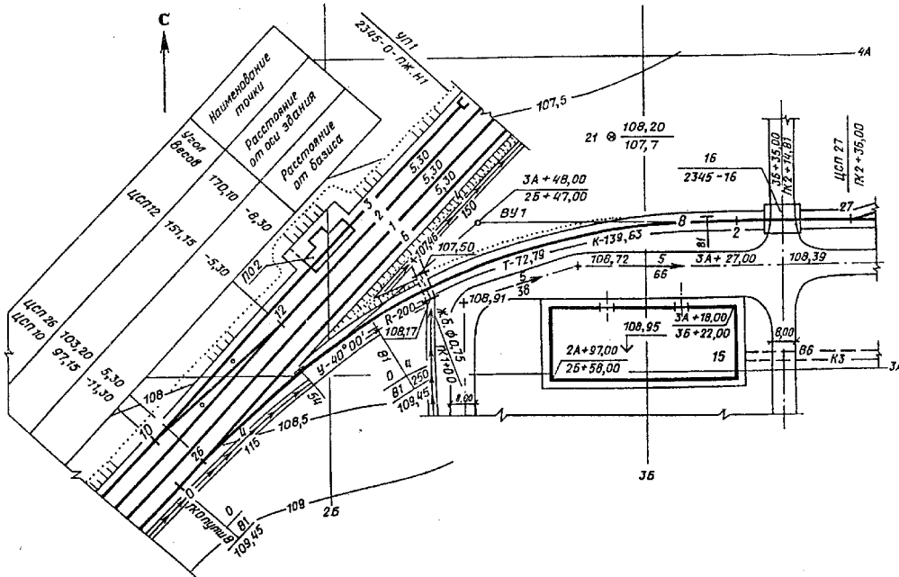
"Пример оформления плана железнодорожных путей на застроенной территории"
