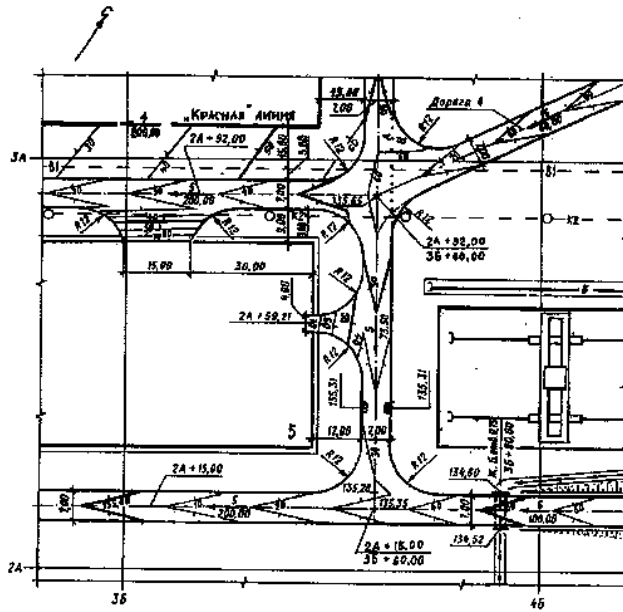
Рисунок А1 — В проектных горизонталях
