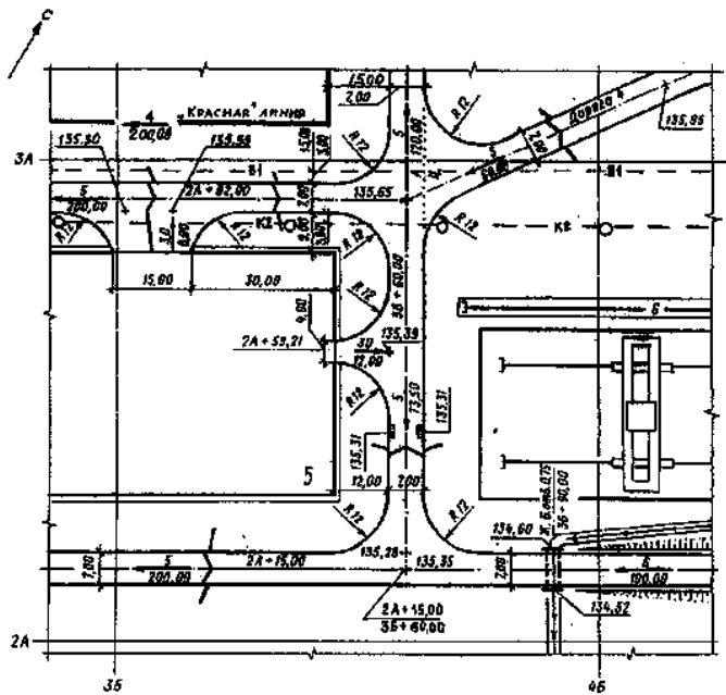
Рисунок А2 — В проектных отметках
