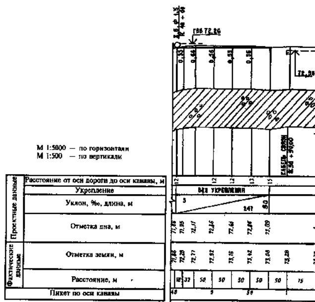
"Пример оформления продольного профиля водоотводной канавы"
