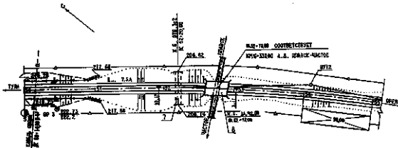
Пример оформления плана автомобильной дороги общего пользования
