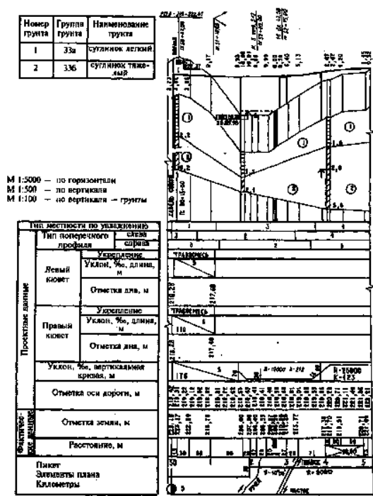
Пример оформления продольного профиля автомобильной дороги общего пользования
