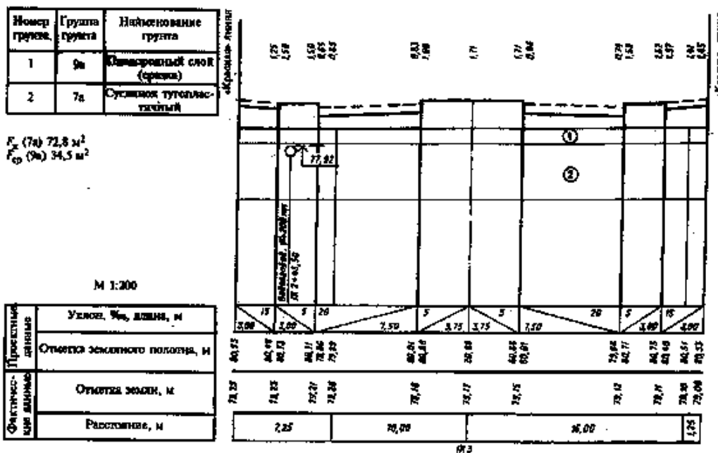
Пример оформления поперечного профиля автомобильной дороги на застроенной территории
