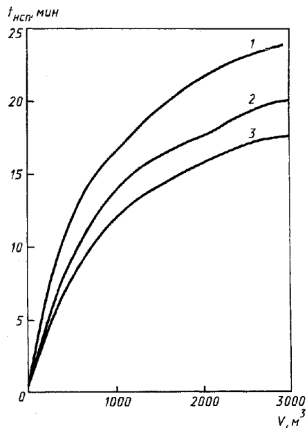
"Рис. Л.1 Зависимость минимальной продолжительности начальной стадии пожара t_{НСП} от объема V , высоты H помещения и количества пожарной нагрузки q "
