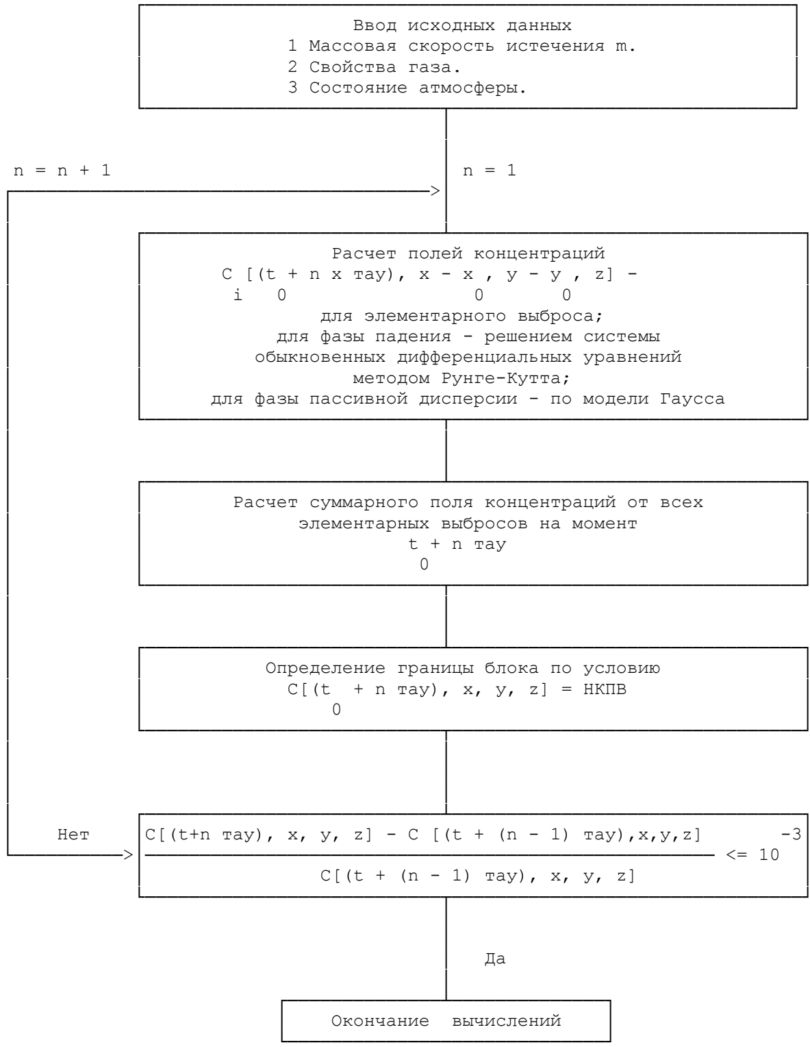
Рисунок Г.1 - Алгоритм расчета параметров паровоздушного облака
