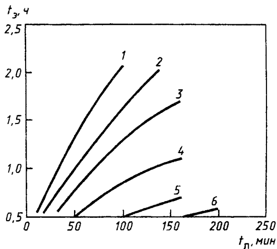
"Рис. Л.3 Зависимость эквивалентной продолжительности пожара t_э от продолжительности пожара для железобетонных и огнезащитных металлических конструкций перекрытия в условиях локальных пожаров t_л (или продолжительности НСП t_{НСП} ) при горении твердых и трудногорючих материалов"
