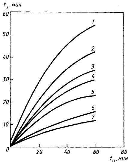
"Рис. Л.5 Зависимость эквивалентной продолжительности пожара t_э от продолжительности пожара t_л для горизонтальных незащищенных металлических конструкций"
