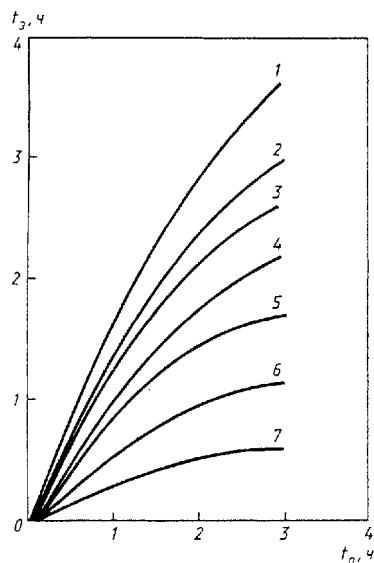
Рисунок Л.7 — Зависимость эквивалентной продолжительности пожара t_э от характерной продолжительности пожара t_п для огнезащищенных металлических и железобетонных конструкций перекрытия
