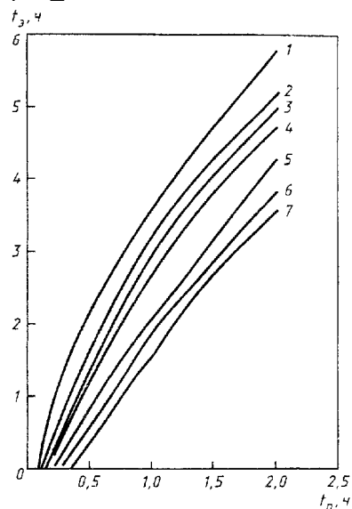
"Рис. Л.7 Зависимость эквивалентной продолжительности пожара t_э от характерной продолжительности пожара t_п для огнезащищенных металлических и железобетонных конструкций перекрытия"
