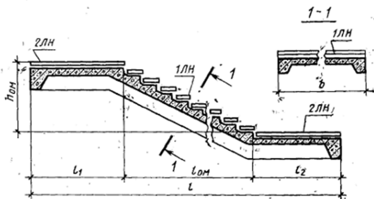
Марш типа ЛМП с двумя полуплощадками
