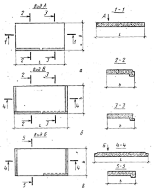
а - площадки длиной 2200 и 2800 мм; б - то же, длиной 2350 и 2950 мм; в - концевая площадка
