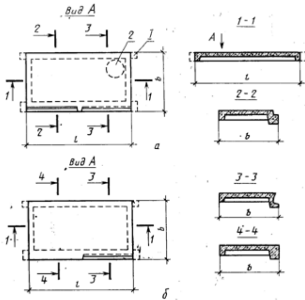
Площадка типа 2ЛП
