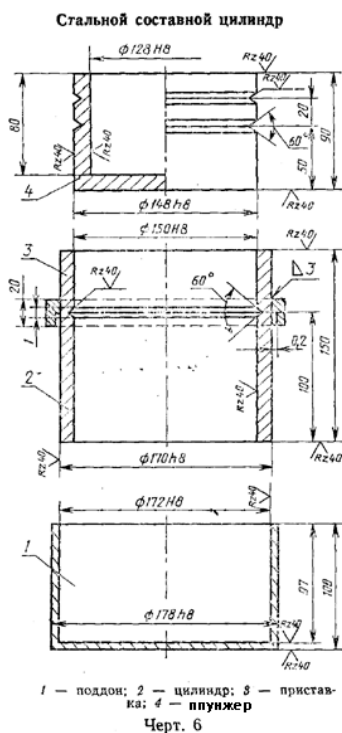
"Черт. 6. Стальной составной цилиндр"
