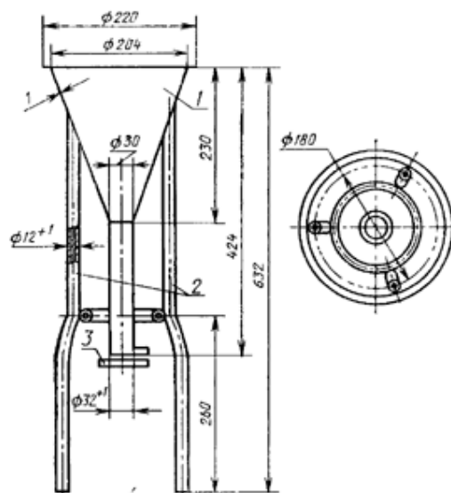
1 — воронка; 2 — опоры; 3 — заслонка Черт. 1
