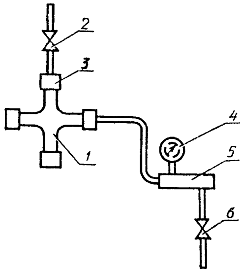
1—изделие; 2—кран для выпуска воздуха; 3—заглушка; 4—манометр; 5—насос; 6—кран для подачи воды Черт. 17
