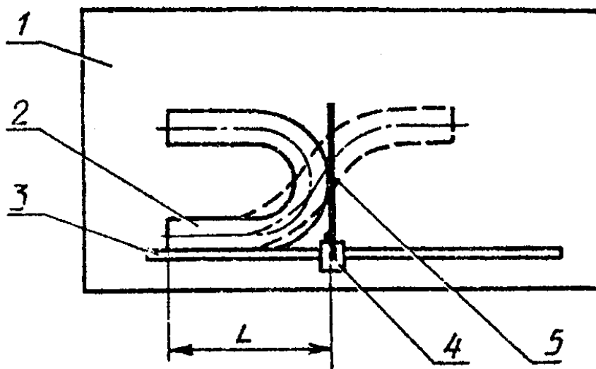
1—контрольная плита; 2—изделие; 3—контрольная линейка; 4—ползун; 5—упор
