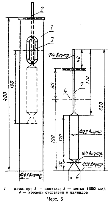
Металлический цилиндр и мерная пипетка
