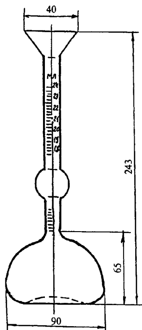
Рисунок 8 — Прибор Ле Шателье
