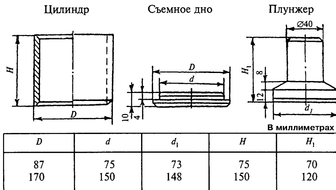
Рисунок 4 — Цилиндры стальные
