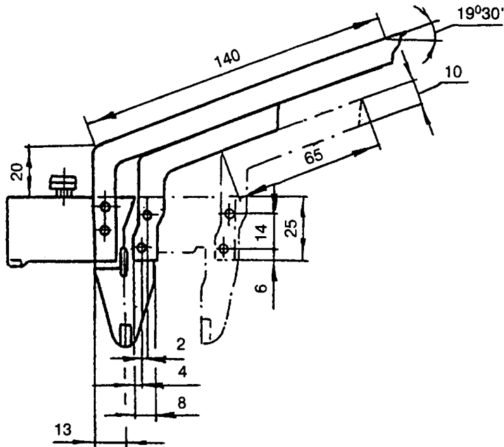
Рисунок 3 – Передвижной шаблон
