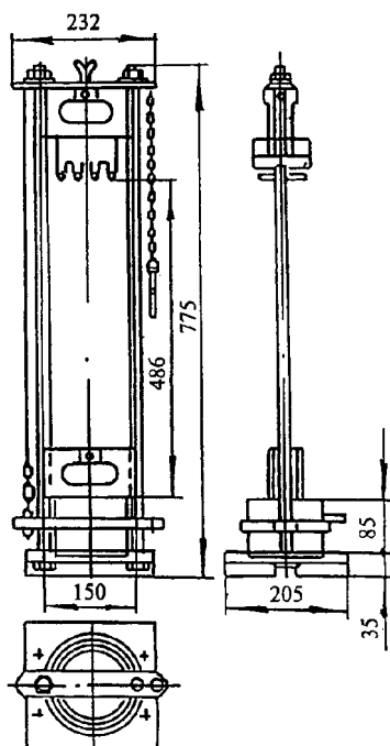
Рисунок 7 – Копер ПМ
