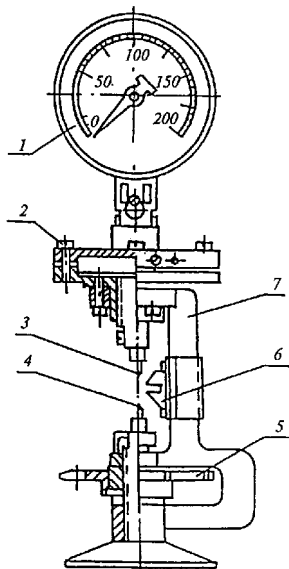
1 — манометр; 2 — гидравлическая мессдоза; 3 — верхний зуб; 4 — нижний зуб; 5 — диск винтового механизма; 6 — шелевой упор; 7 — корпус прибора
