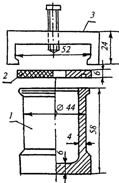
Рисунок 10 — Сосуд из коррозионно-стойкого материала
