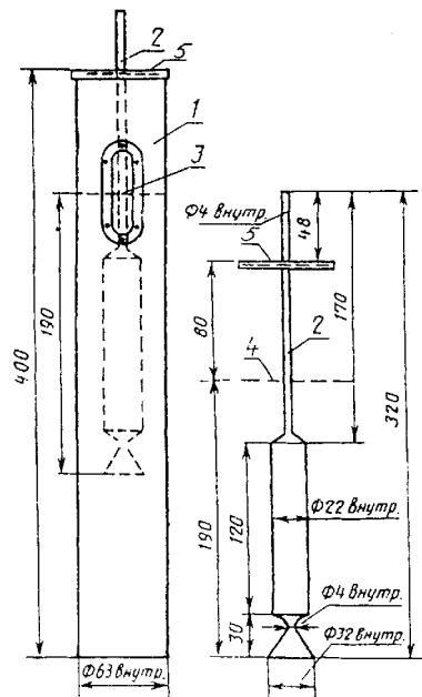
1 — цилиндр; 2 — пипетка; 3 — метка на цилиндре (1000 мл); 4 — уровень суспензии в цилиндре; 5 — опорная крышка пипетки
