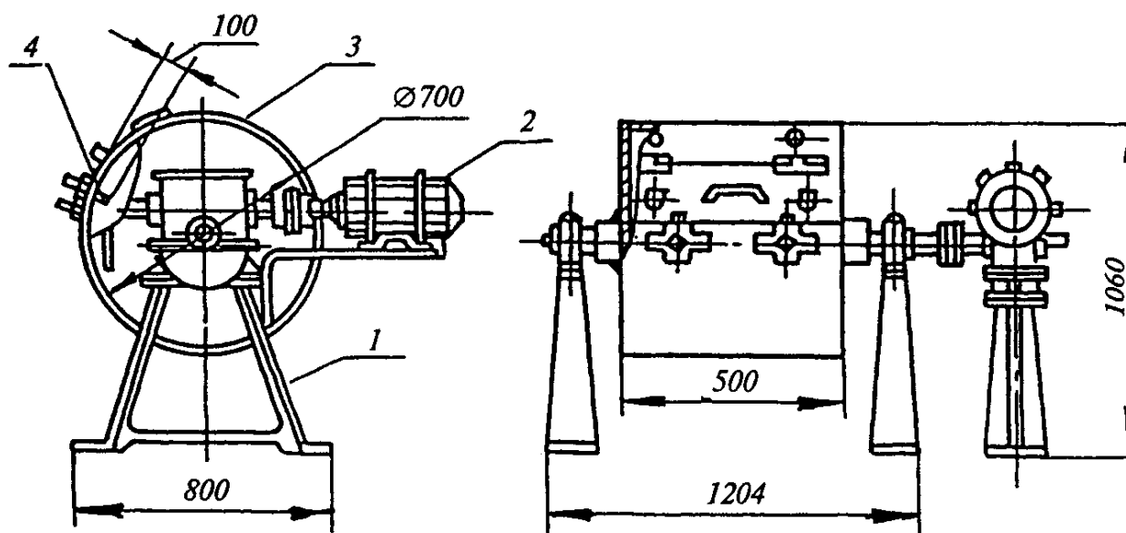
1 — станина; 2 — двигатель; 3 — барабан; 4 — полка барабана
