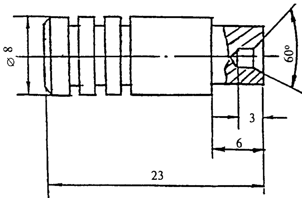
Рисунок 13 — Репер для испытаний
