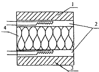
1 — нагреватель; 2 — тепломеры; 3 — холодильник; 4 — испытываемый образец
