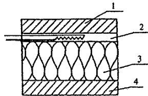
1 — нагреватель; 2 — тепломер; 3 — испытываемый образец; 4 — холодильник
