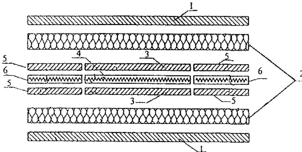
1 — холодильник; 2 — испытываемые образцы; 3 — плиты нагревателя зоны измерения; 4 — обмотка нагревателя зоны измерения; 5 — плиты нагревателя охранной зоны; 6 — обмотка нагревателя охранной зоны
