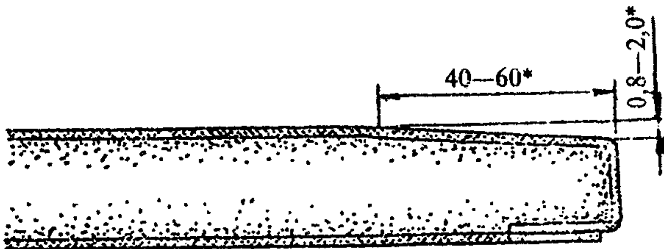
Рисунок 2 — Утоненная с лицевой стороны кромка (УК)
