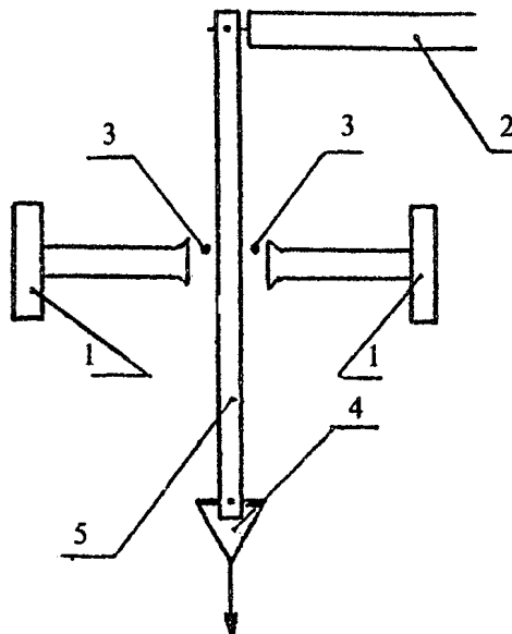
Рисунок 7 — Схема установки для испытания образцов на сопротивляемость воздействию открытого пламени с двух сторон
