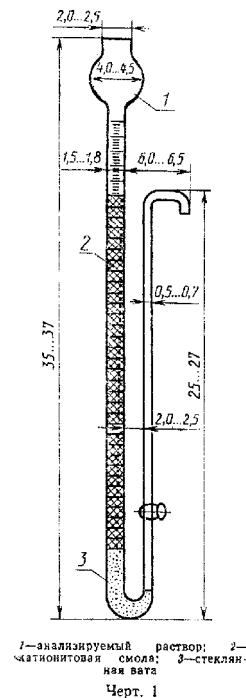
Зарядка ионообменной колонки
