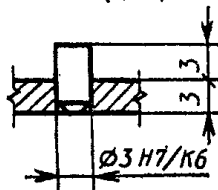
1—ручка; 2—стержень; 3—лопатка; 4—штырь
