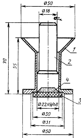
1—воронка; 2—пуансон; 3—графитовая подложка; 4—смесь СОП со смесью для сплавления
