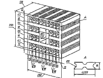
Рисунок А19 — Кирпич с 30 вертикальными канавками и углублением для зацепки при кладке (пустотность 45 %)
