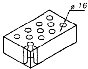
Рисунок А13 — Кирпич с 11 сквозными отверстиями (пустотность 8,2 %)
