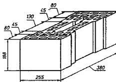
Рисунок А27 — Камень с пустотностью 55 %
